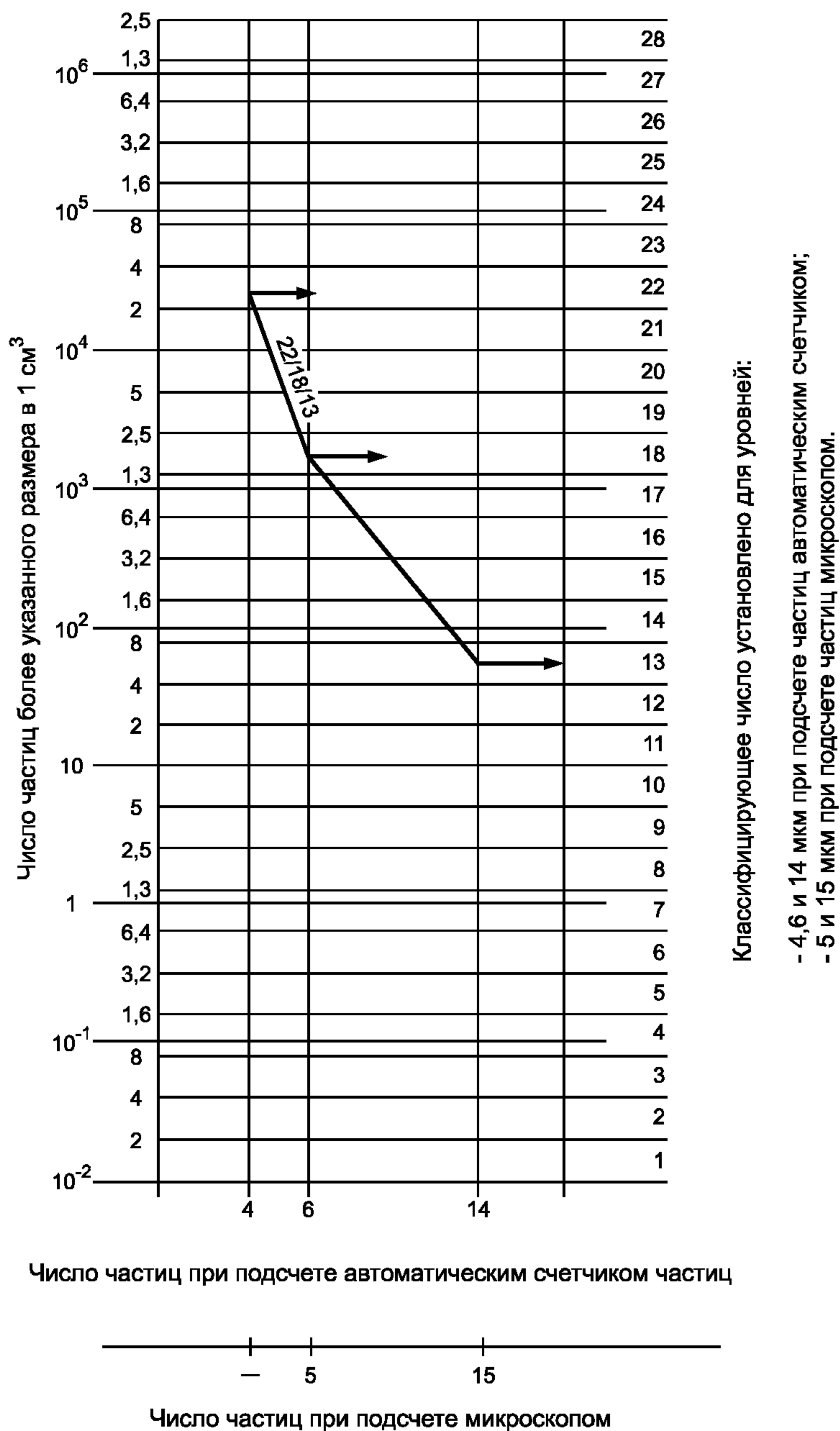
Рисунок Б.1 — Графическое представление кодового числа
