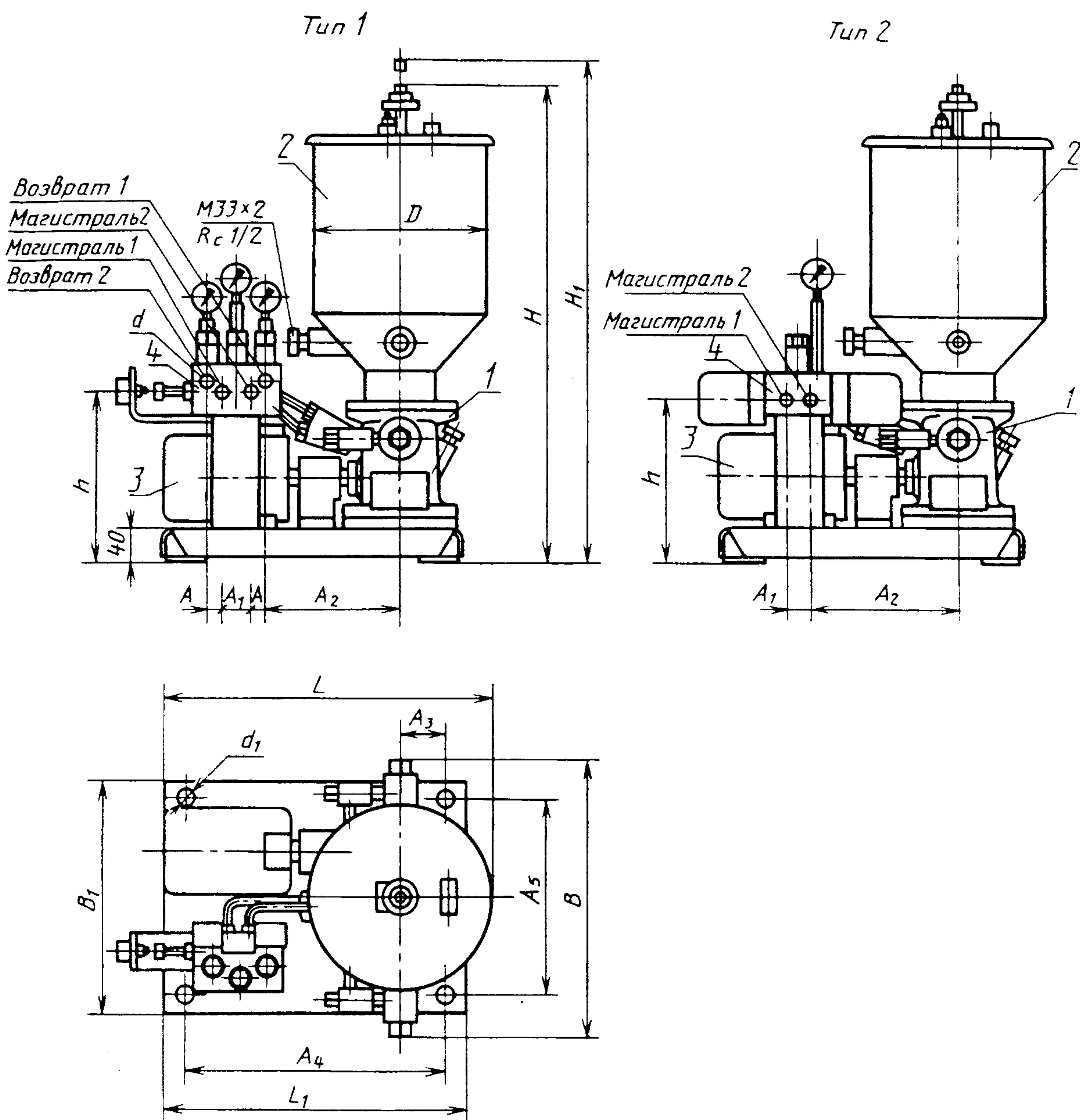
1 — насос; 2 — резервуар; 3 — электродвигатель; 4 — двухмагистральный распределитель
