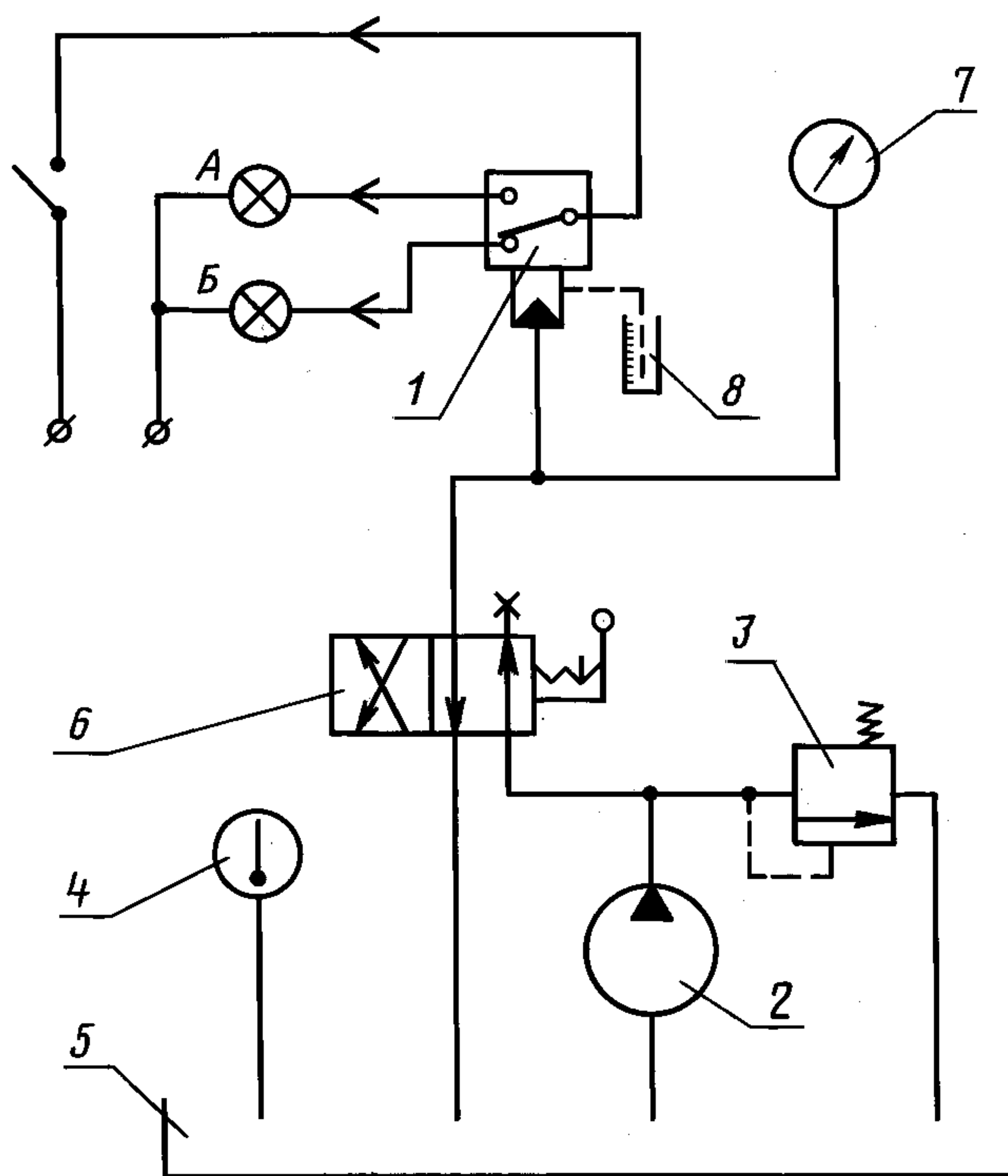
Схема испытания реле
