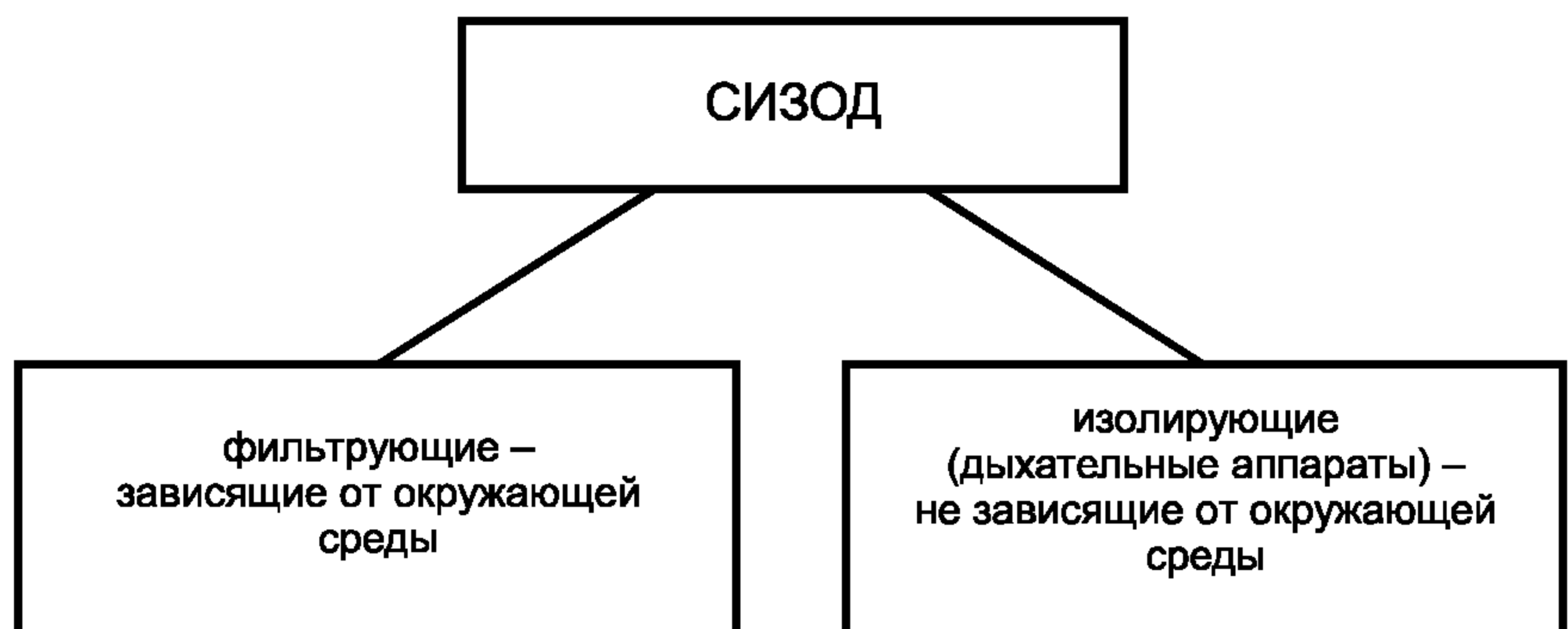
Рисунок 2 — Классификация средств индивидуальной защиты органов дыхания
