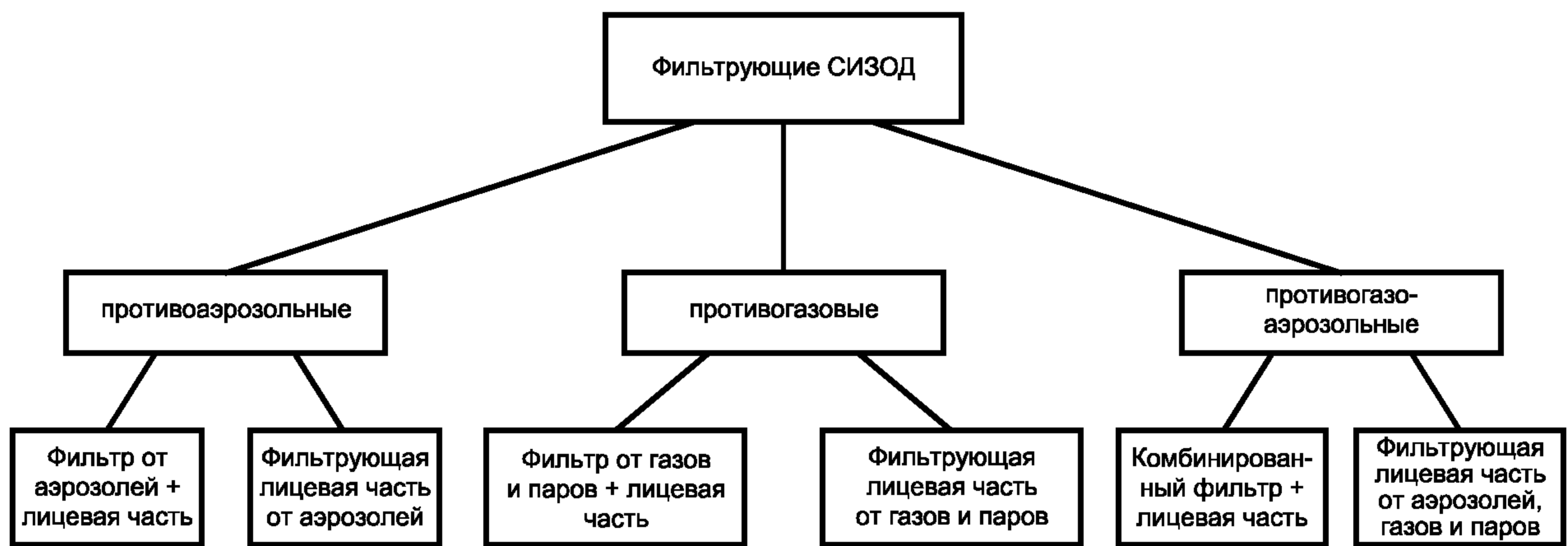
Рисунок 3 — Классификация фильтрующих средств индивидуальной защиты органов дыхания
