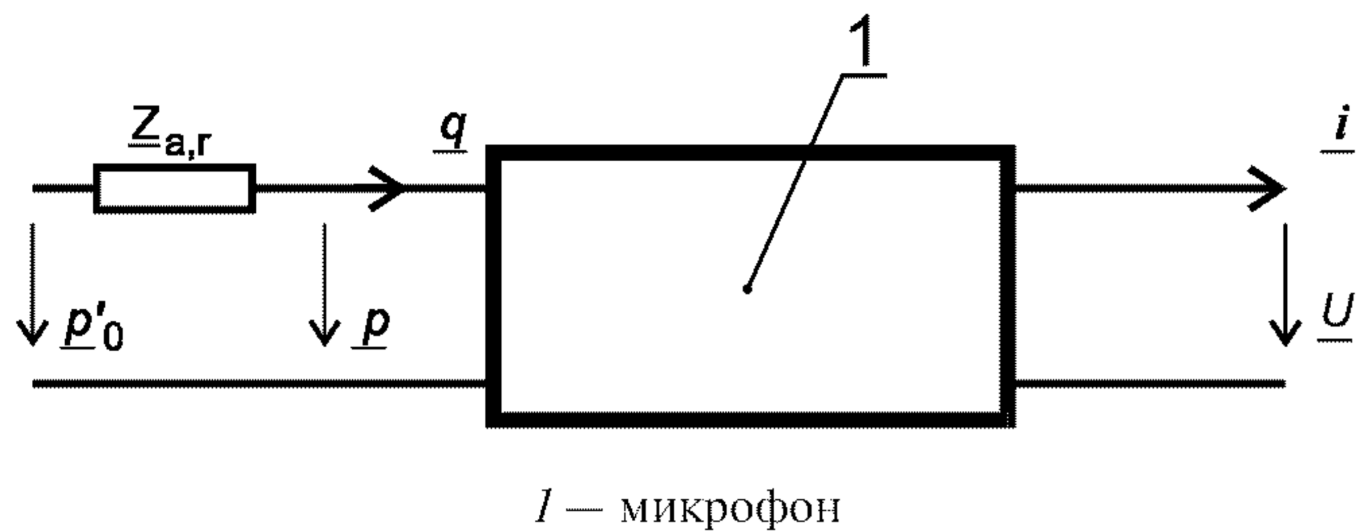
Рисунок 1 — Эквивалентная схема микрофона-приемника в свободном поле
