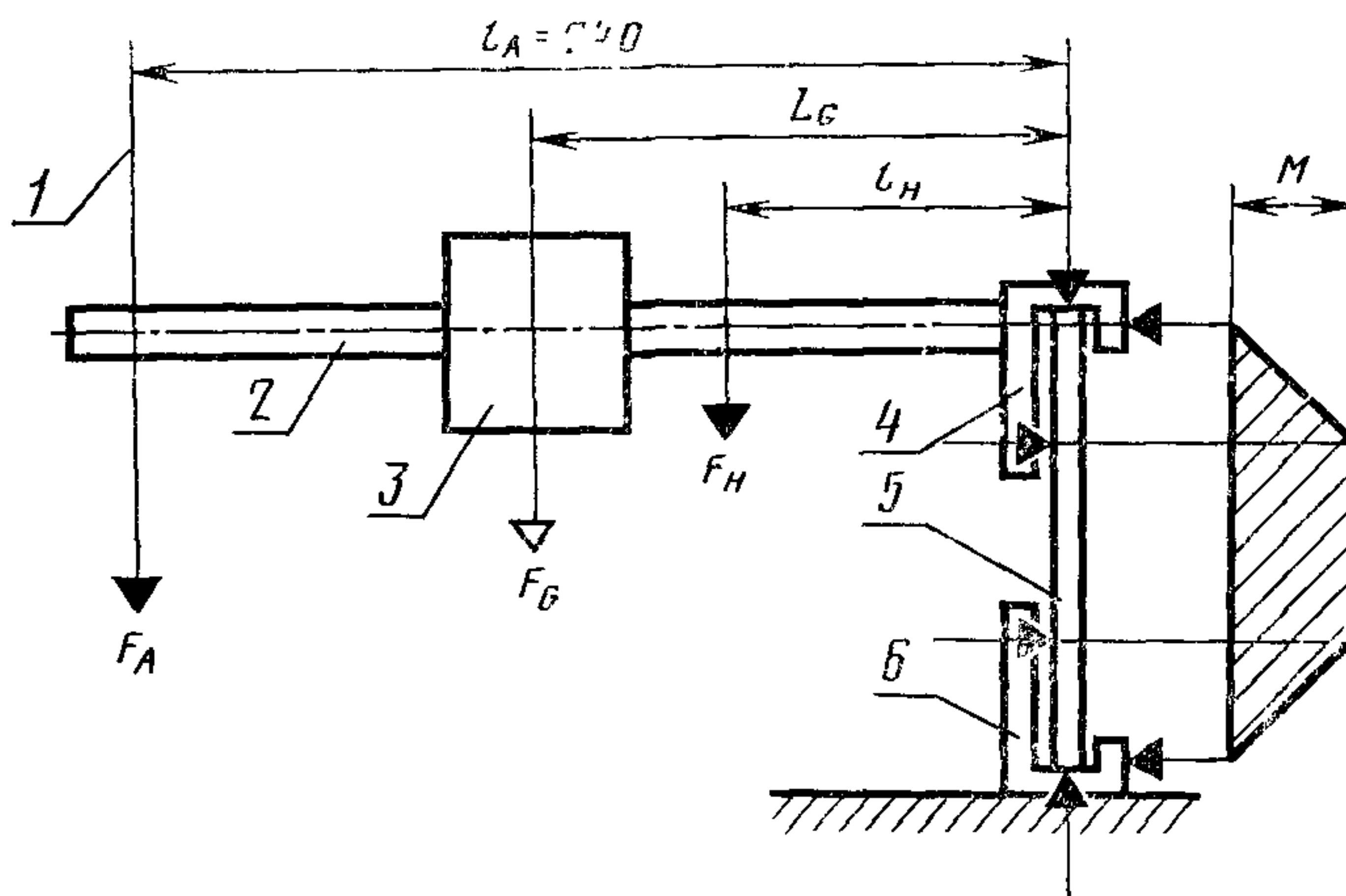
Зажимно-нагрузочное устройство
