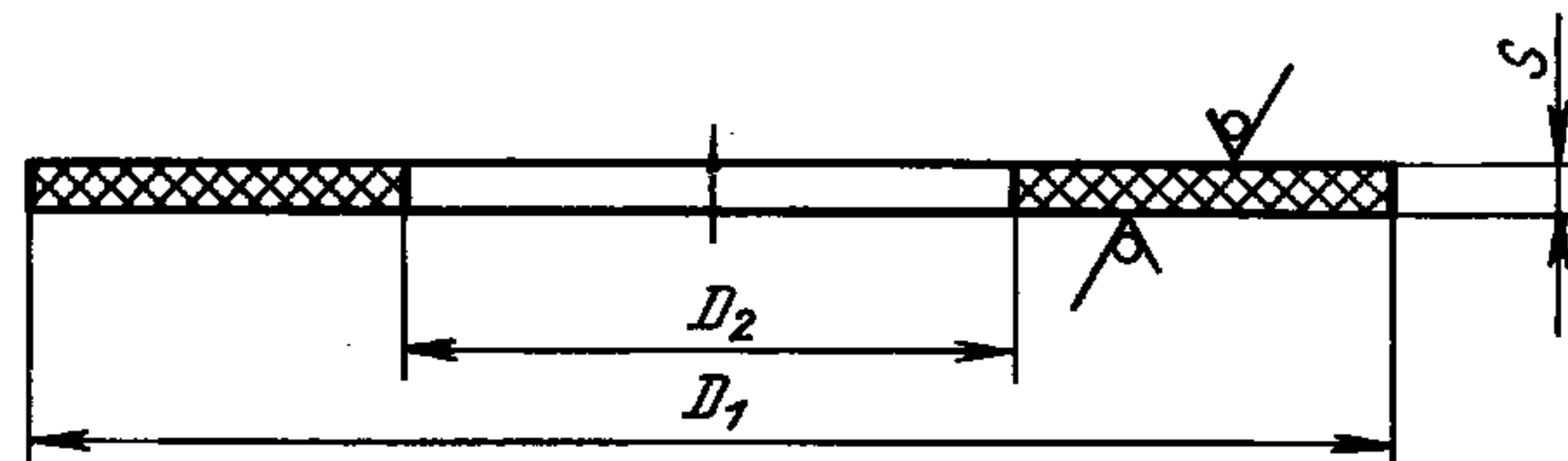
Размеры, мм
