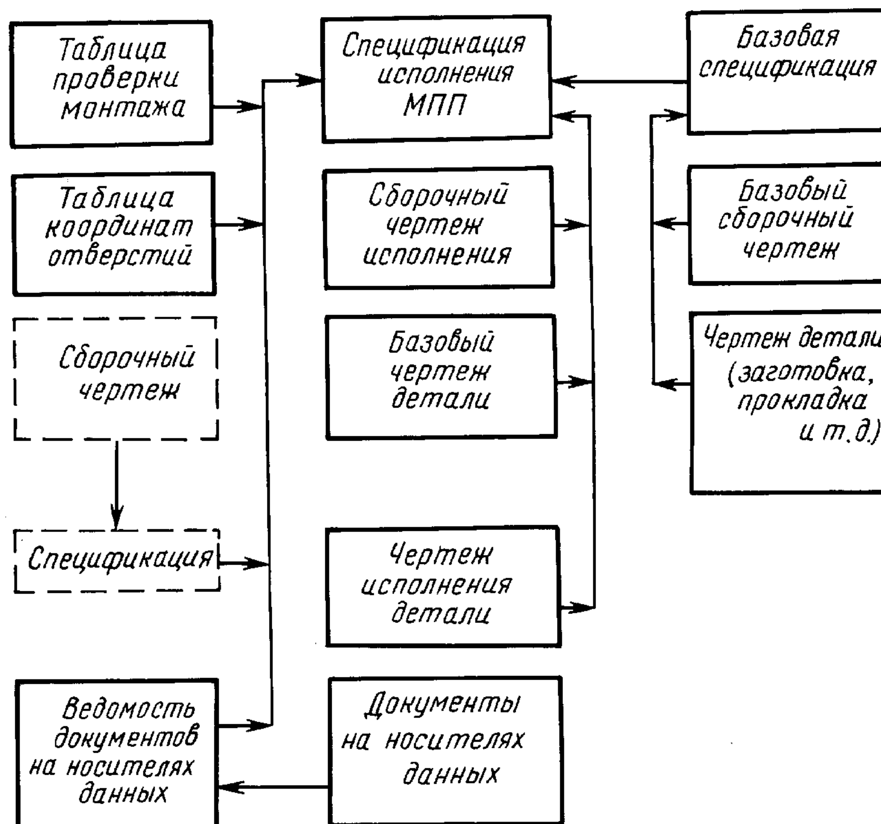
Пример построения комплекта конструкторских документов для МПП
