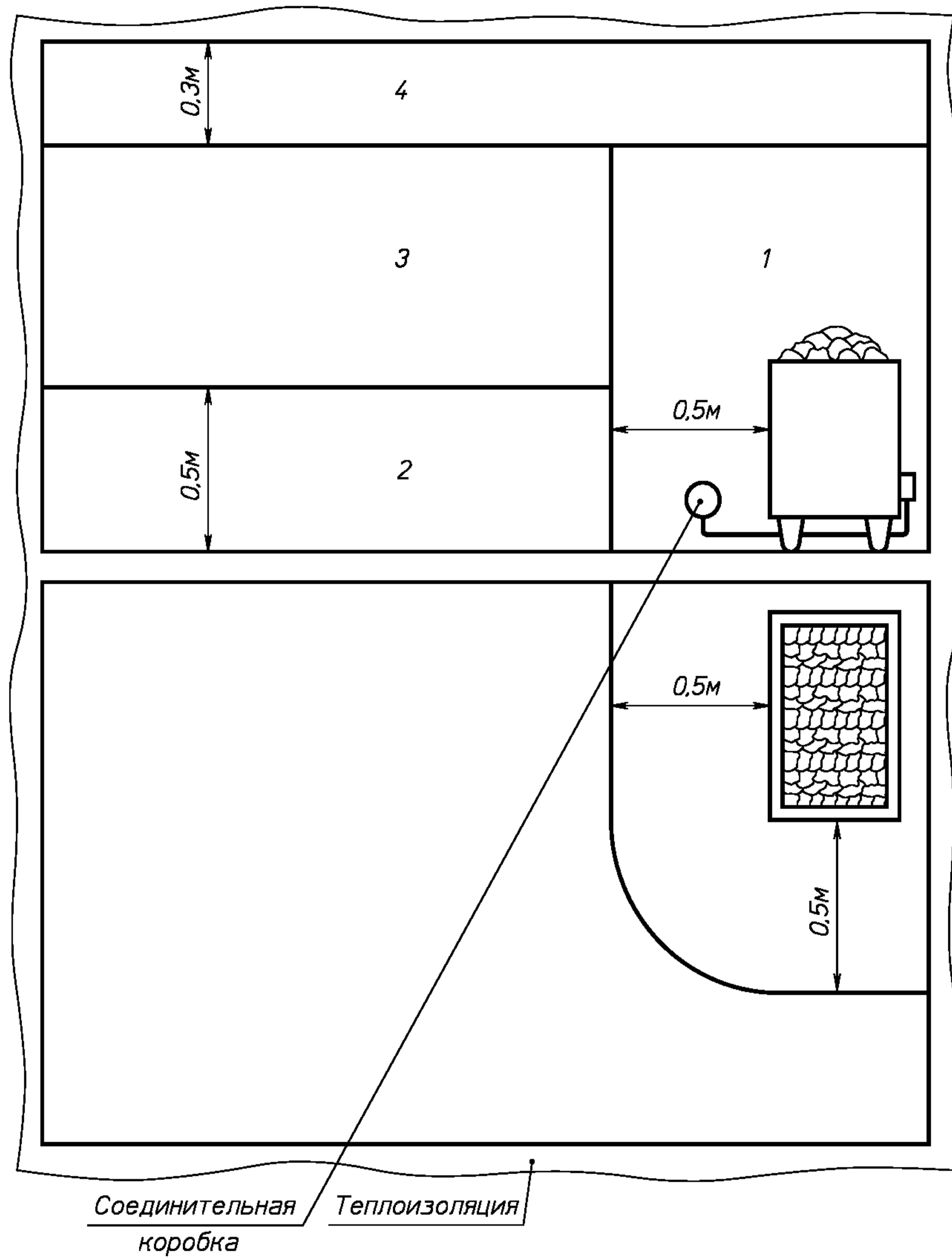
Рисунок 703А — Зоны температуры окружающей среды
