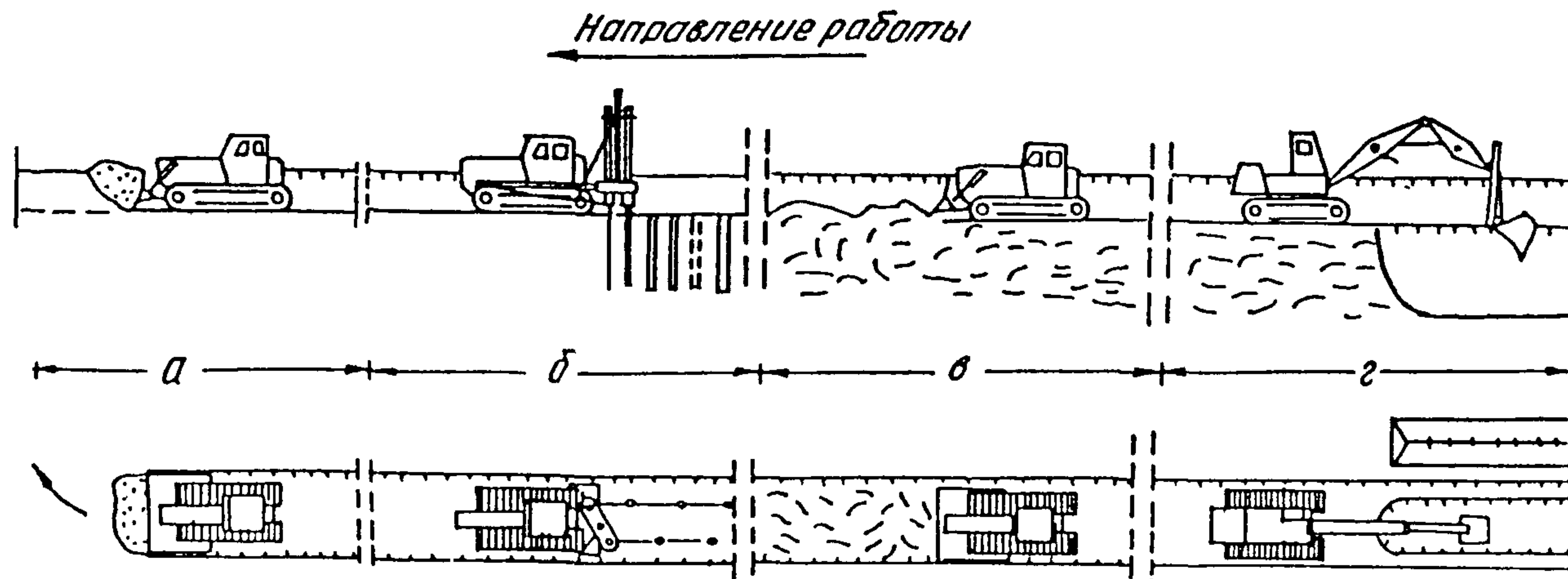
Рис.5. Схема разработки траншей в мерзлом грунте с предварительным рыхлением их буровзрывным способом:
