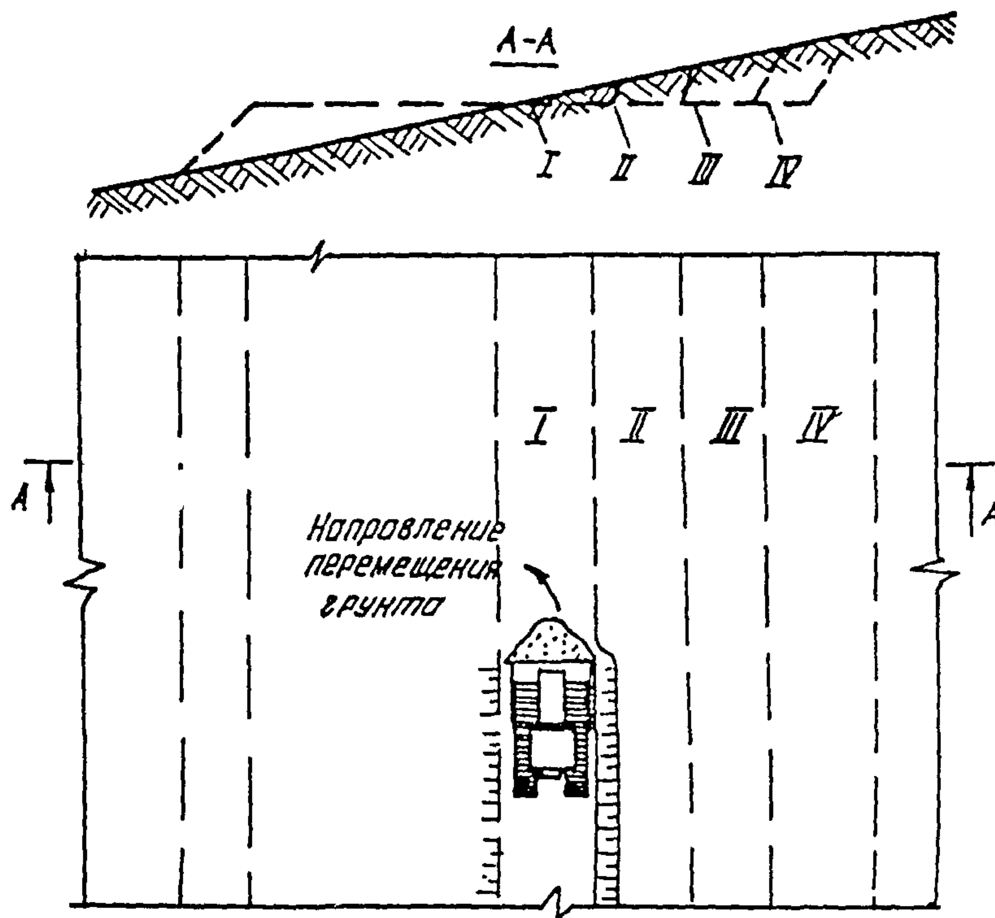
Рис.3. Схема разработки полки на склонах продольными проходами бульдозера:
