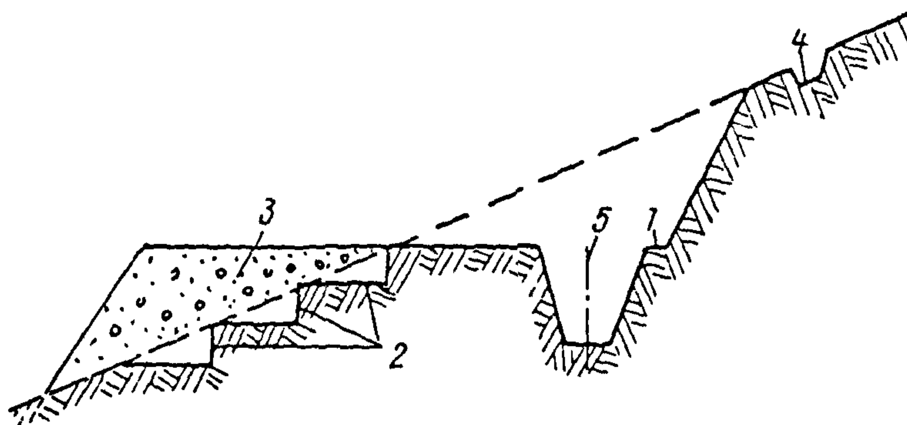
Рис.1. Схема поперечного разреза полки: 1 - полувыемка; 2 - уступы для устойчивости полунасыпи; 3 - полунасыпь; 4 - нагорная водоотводная канава; 5 - траншея для трубопровода
