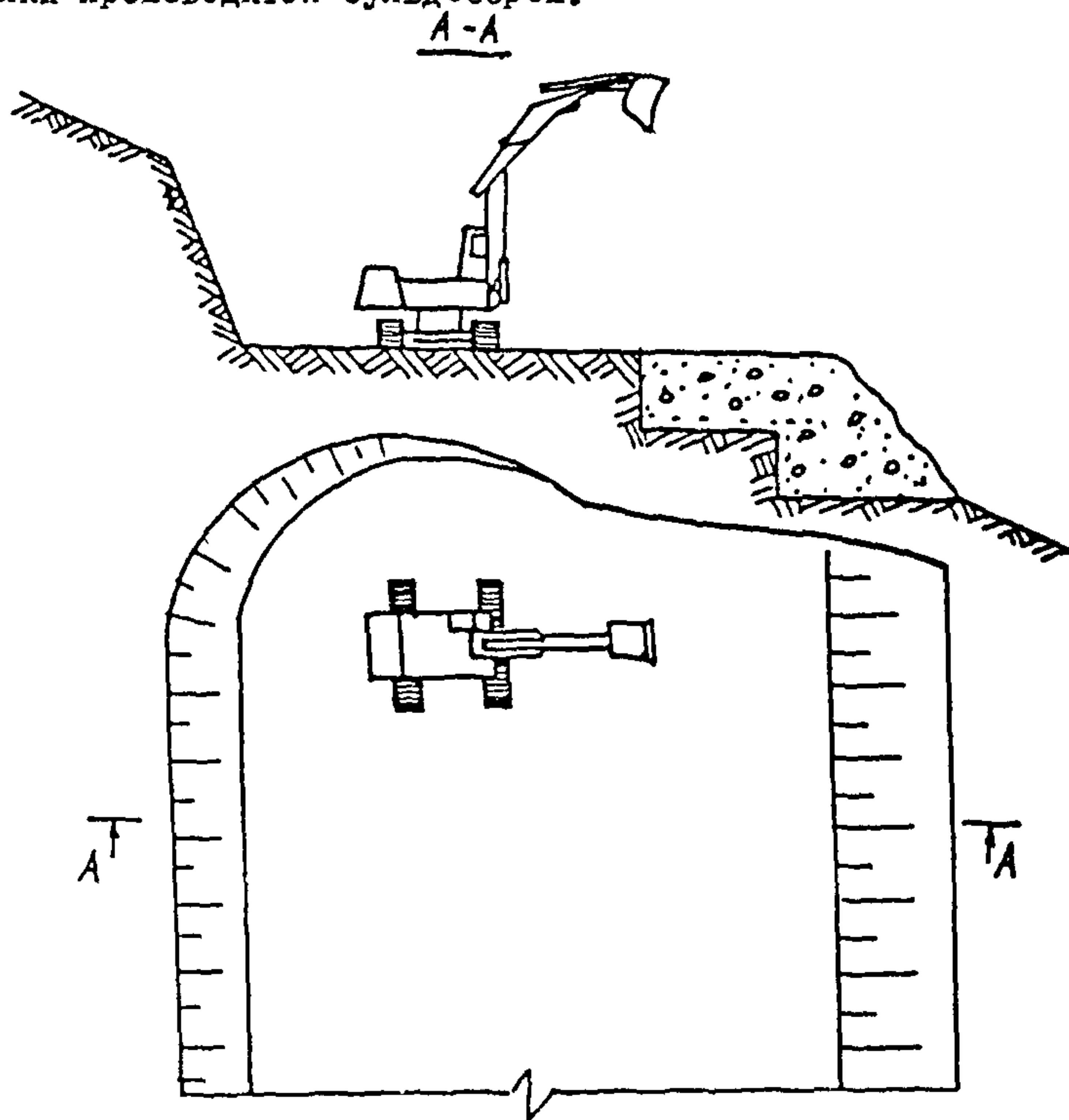
Рис.4. Схема разработки полков экскаватором
