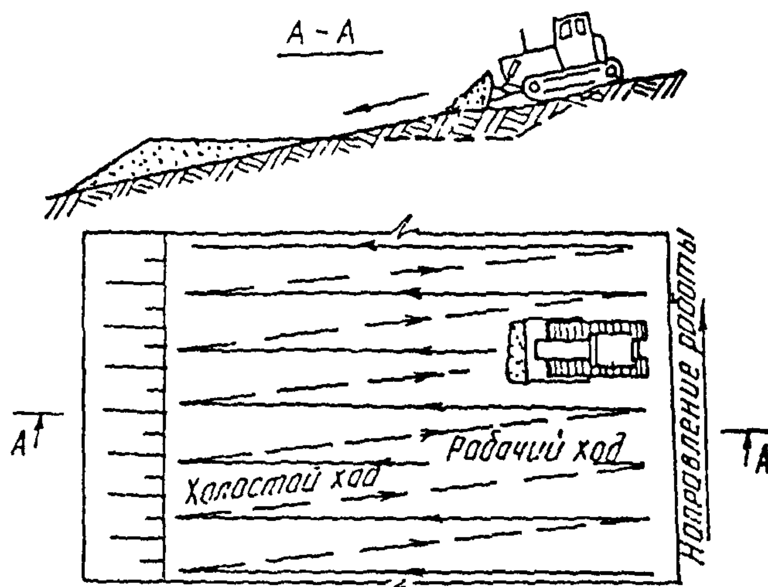
Рис.2. Схема разработки полок на склонах поперечными проходами бульдозера
