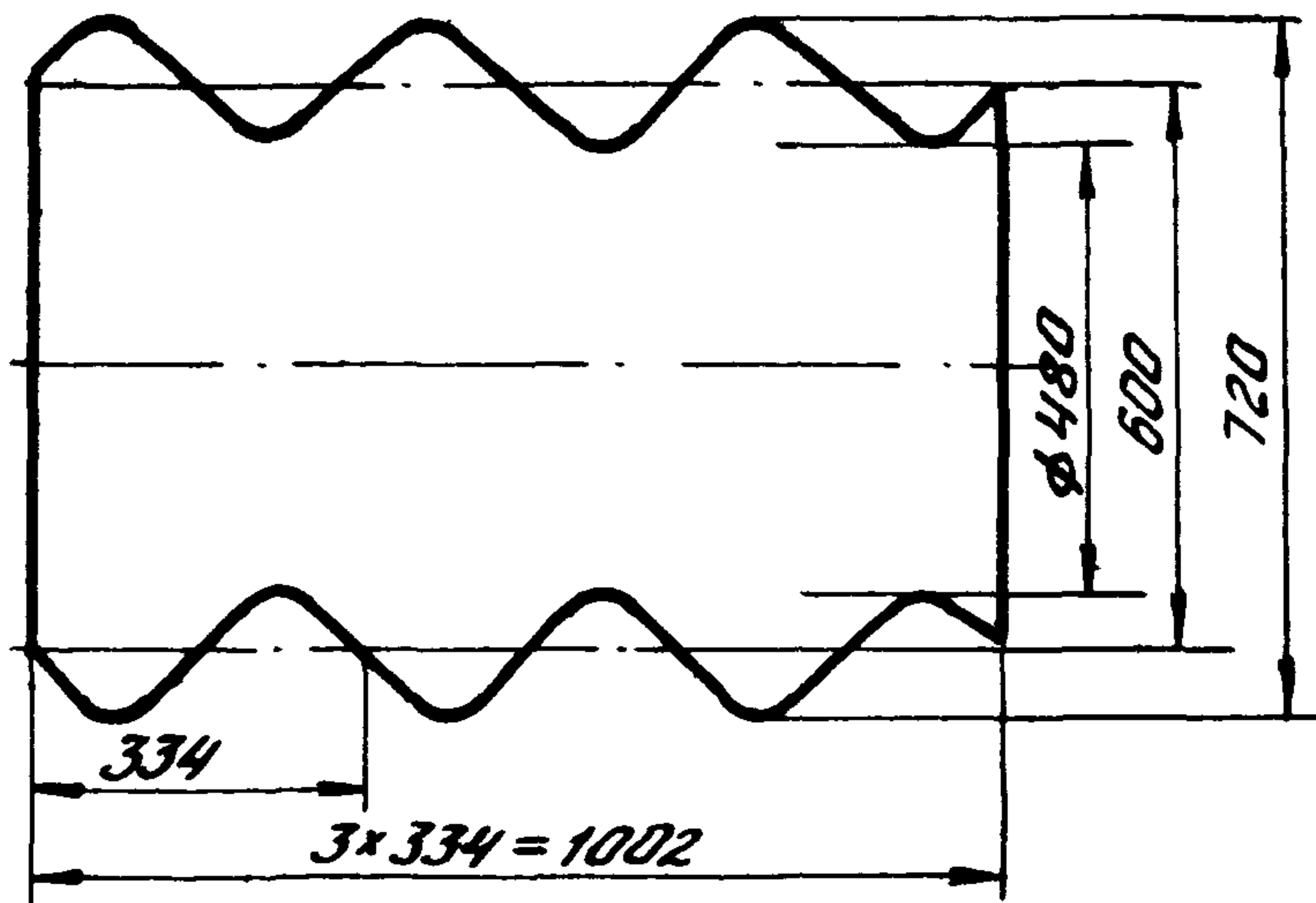
Рис. 4. Секция глушителя с гофрированной стенкой
