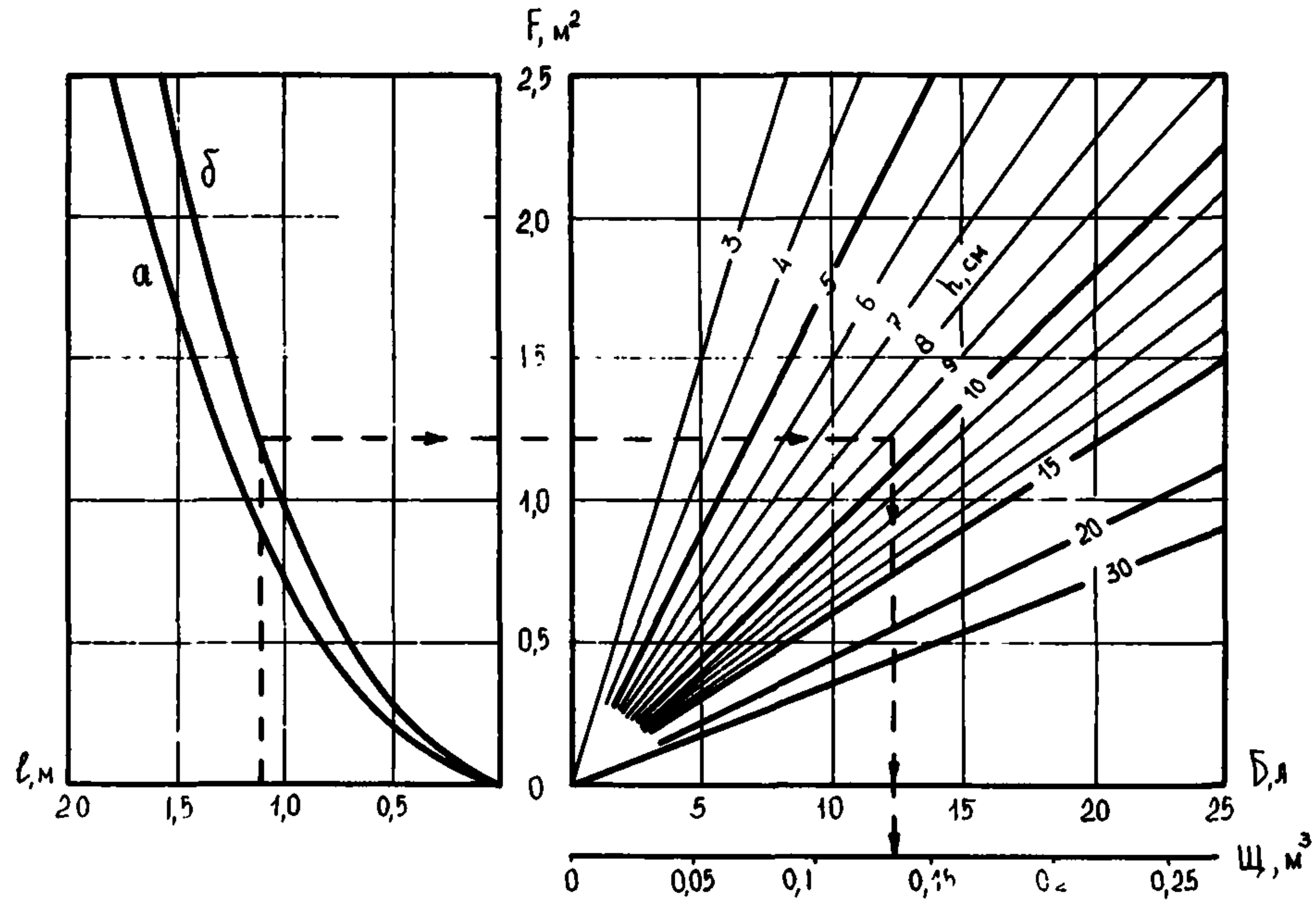
Рис. I. Расход битума ( B, \text{л} ) и щебня ( \text{Щ}, \text{м}^3 ) в зависимости от полусуммы размеров выбоины ( l, \text{м} ) и ее глубины ( h, \text{см} ). а - форма выбоины подобна кругу; б - форма выбоины подобна прямоугольнику; F - площадь выбоины, кв.м.
