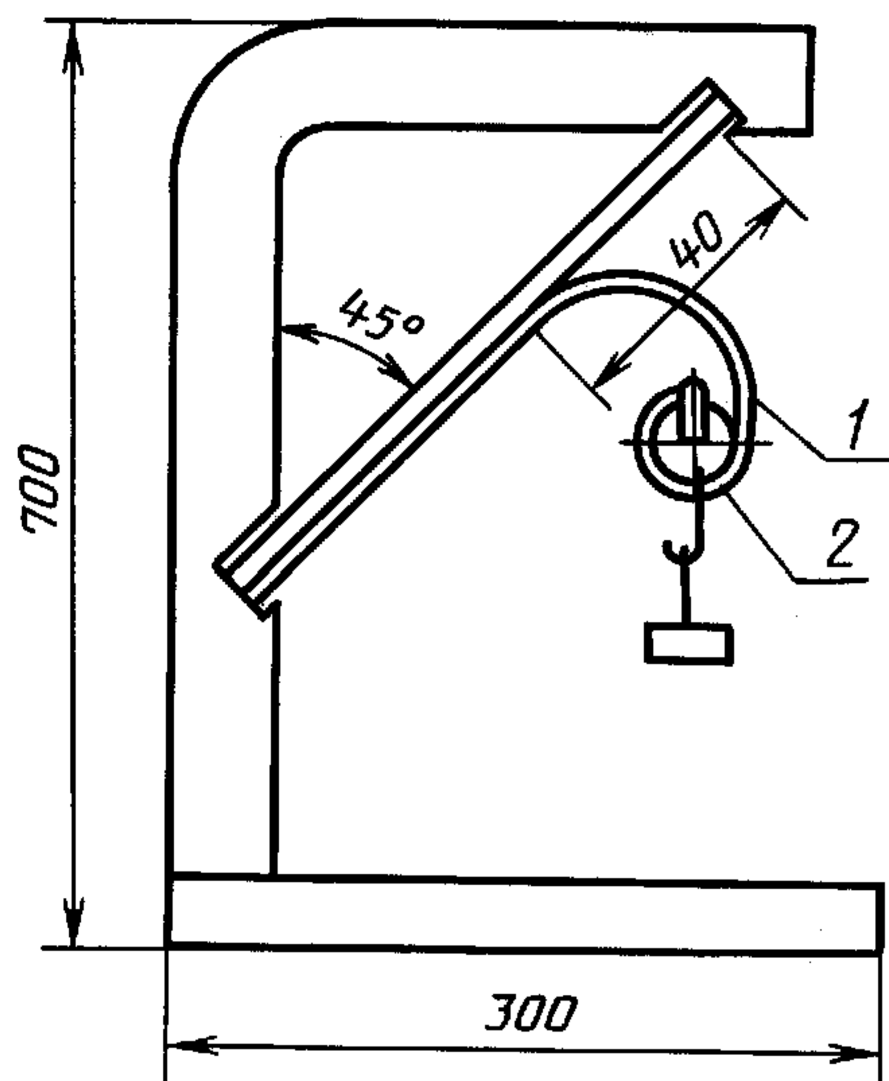
Схема приспособления для определения качества снимаемости
