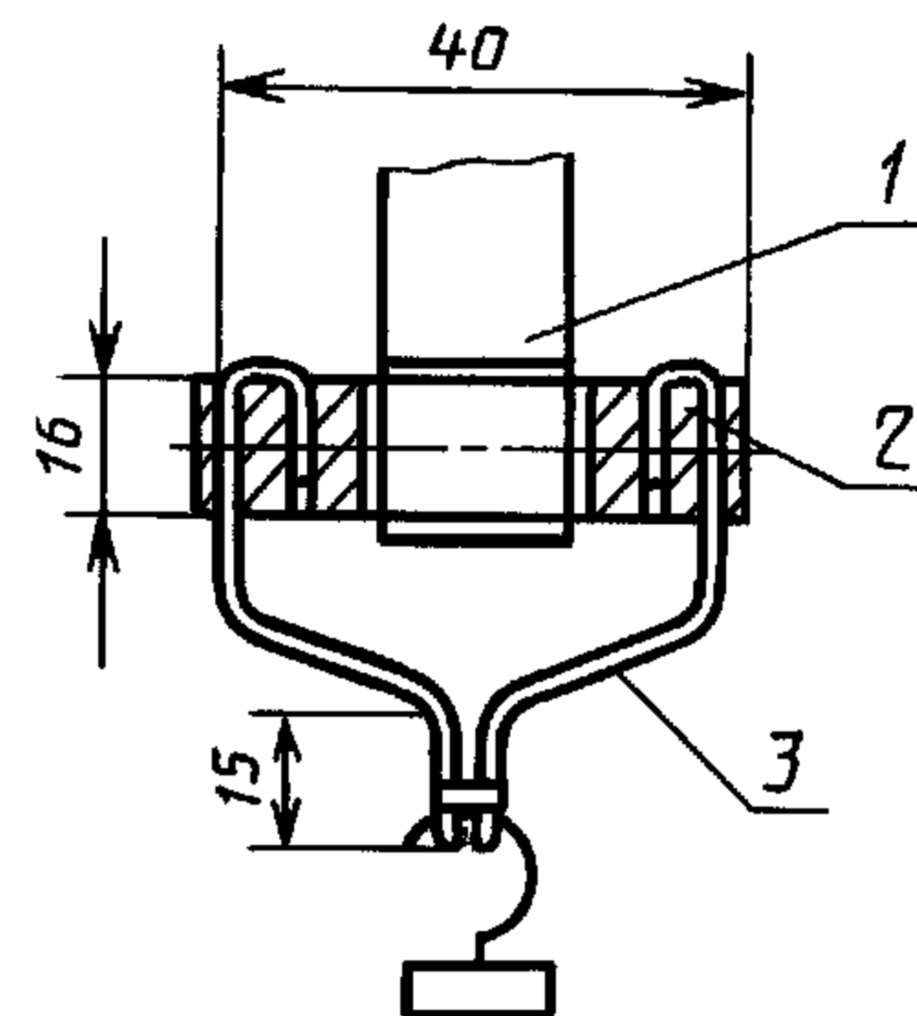
Схема зажимного устройства
