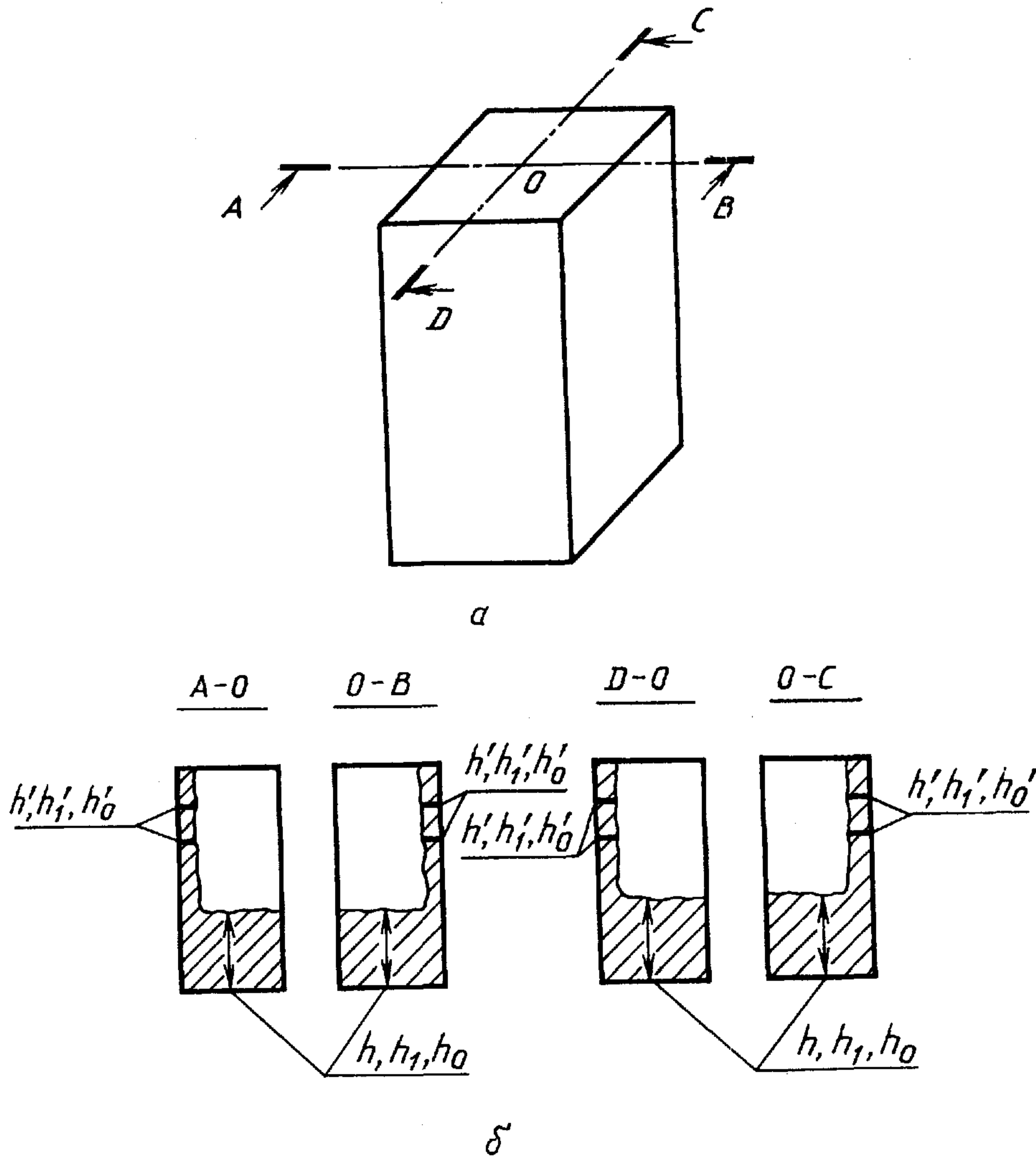
Схема раскалывания образцов древесины и измерения глубины пропитки
