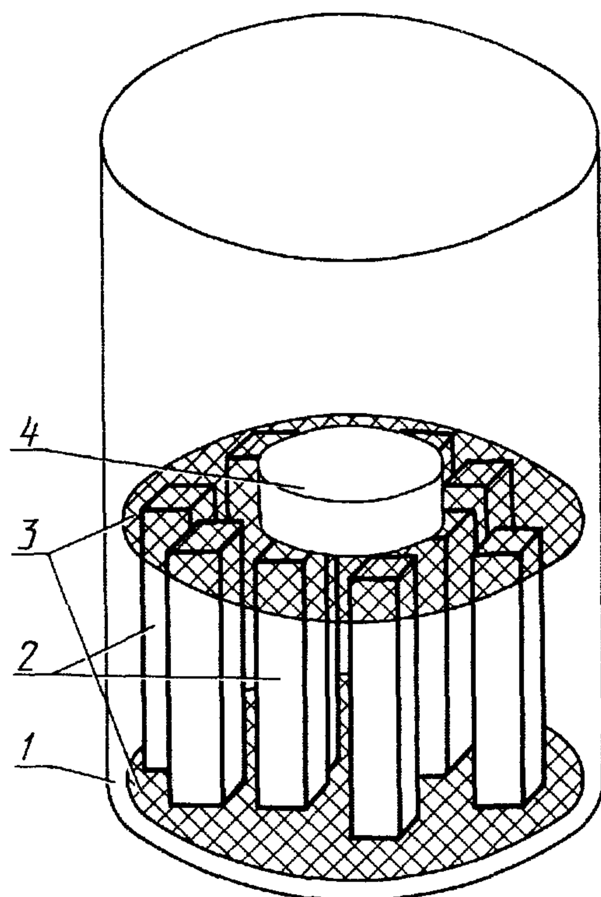
Схема укладки образцов древесины для пропитки
