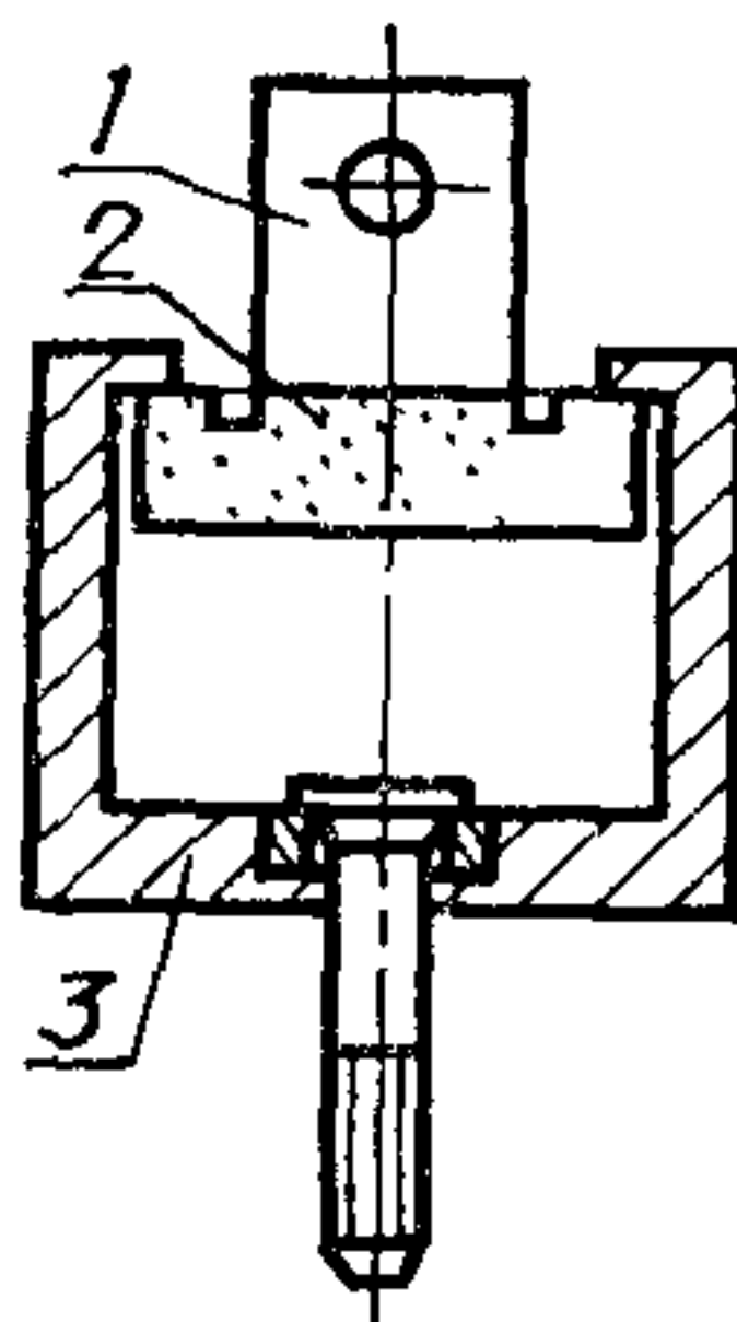
1—испытательная головка; 2—образец; 3—захват.
