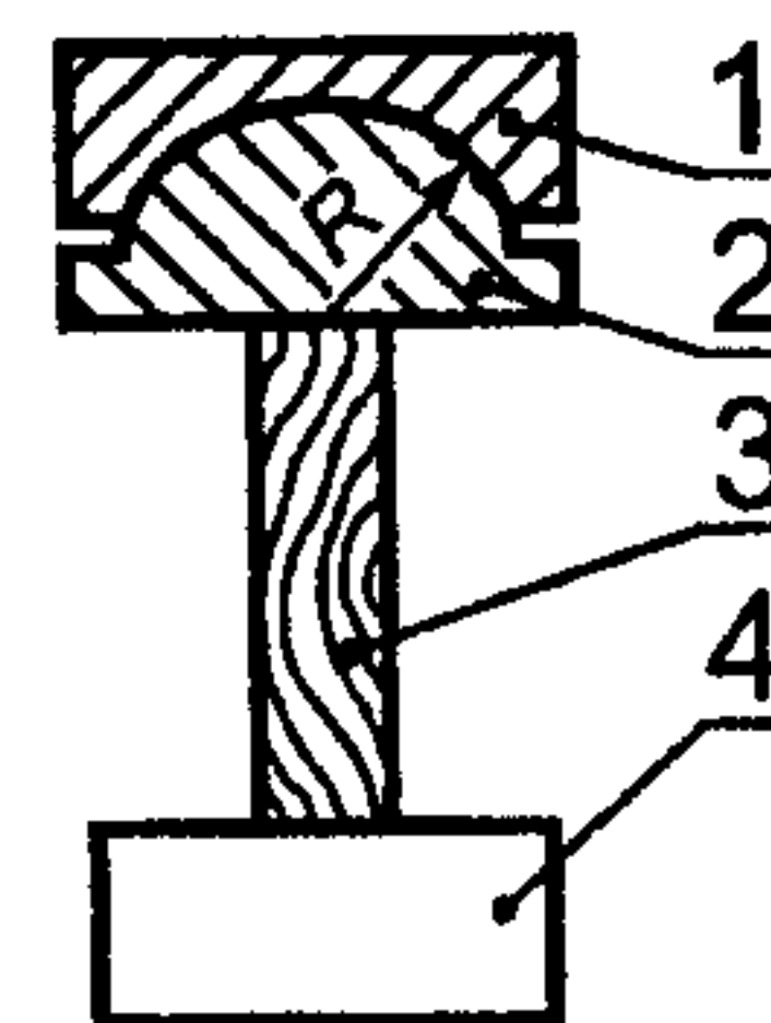
1, 2 — самоустанавливающиеся пластины; 3 — образец; 4 — нижняя платформа испытательной машины
