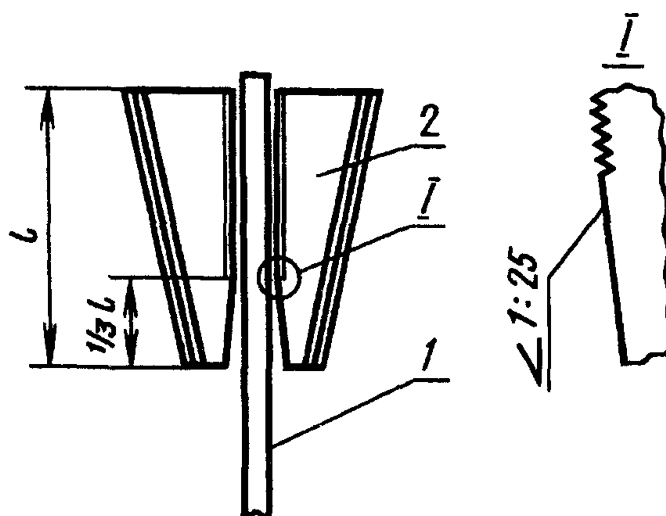
1 — образец; 2 — щечка захвата
