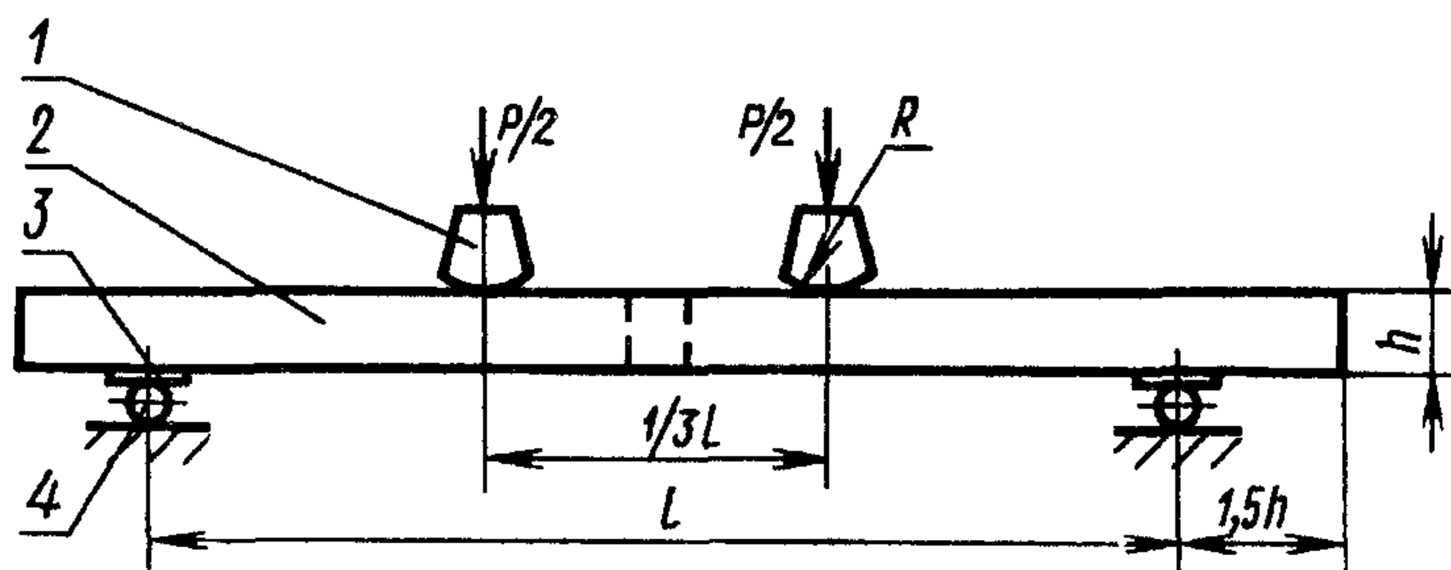
1 — нагружающий нож; 2 — образец; 3 — стальная площадка; 4 — ось (каток)
