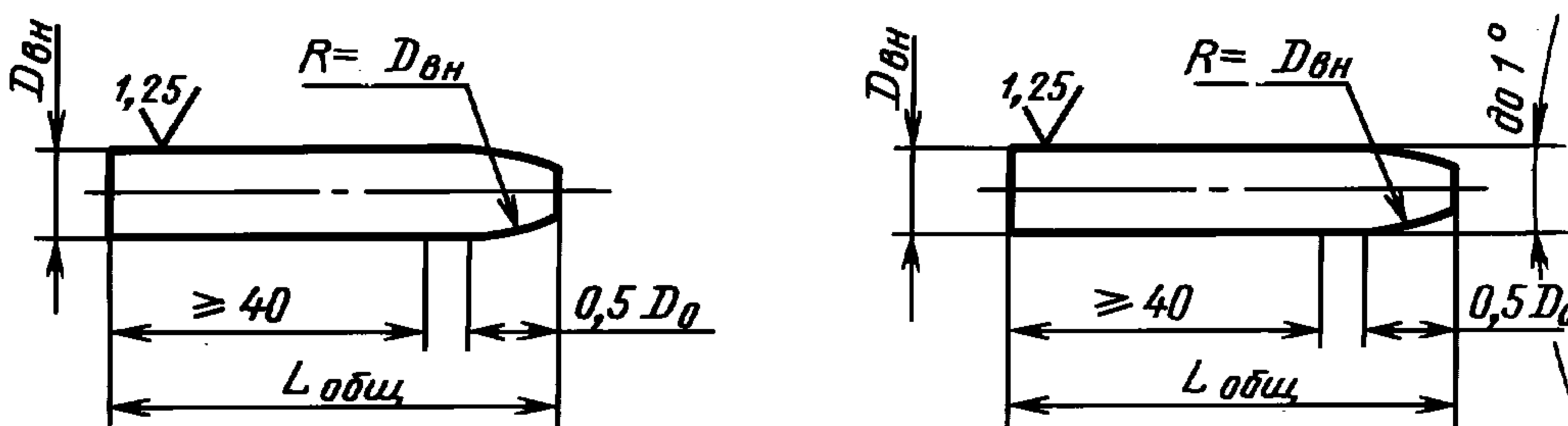
Цилиндрическая пробка
