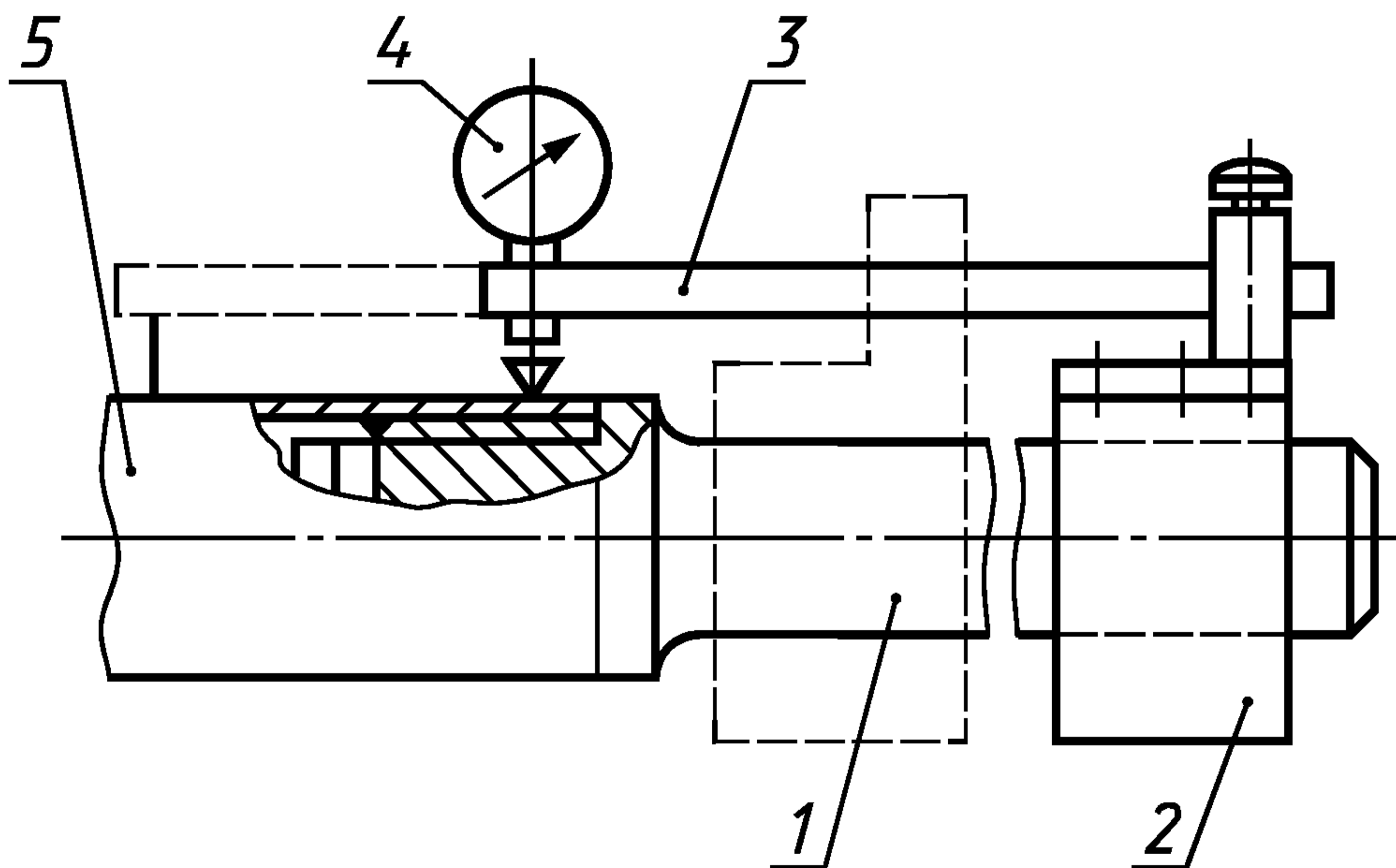
1 — оправка; 2 — втулка; 3 — державка; 4 — индикаторная головка; 5 — труба
