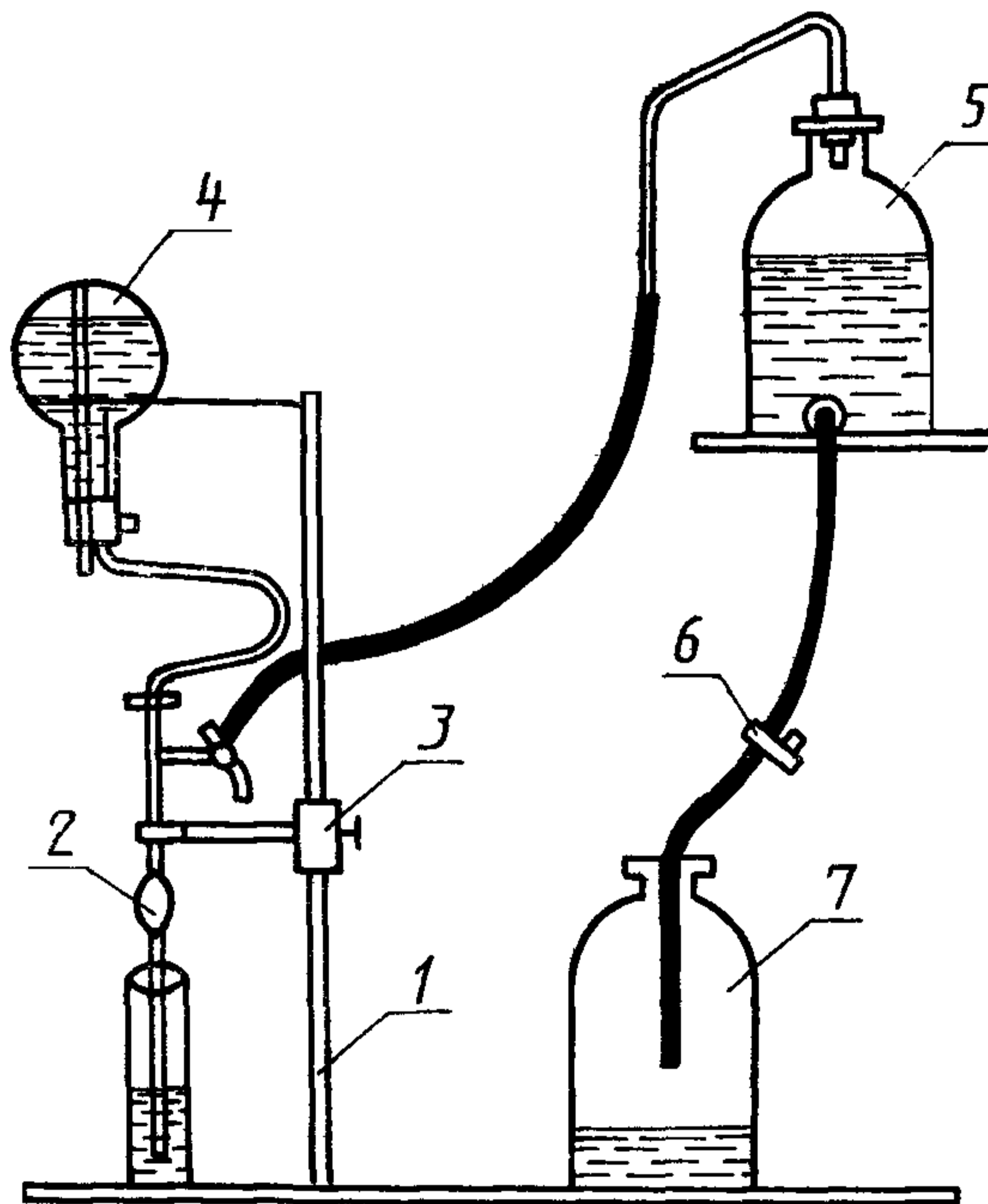
1 — штатив; 2 — пипетка вместимостью 25 см 3 ; 3 — упор; 4 — колба для промывания пипетки; 5 — аспиратор; 6 — зажим; 7 — водослив
