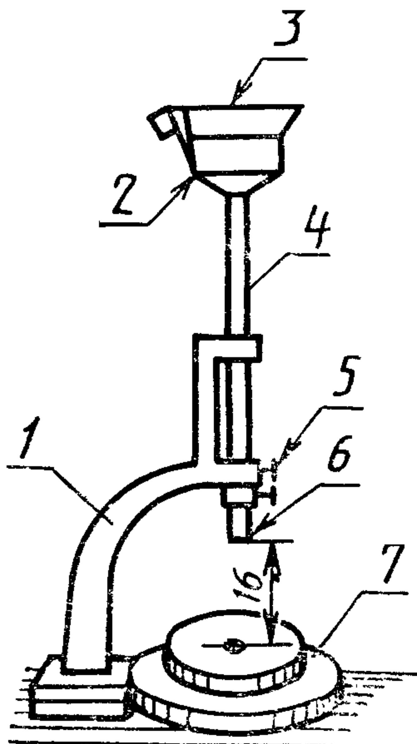
1 — станина; 2 — деревянный диск; 3 — фарфоровая чашка; 4 — цилиндрический стержень; 5 — винт; 6 — упор; 7 — опорная плита
