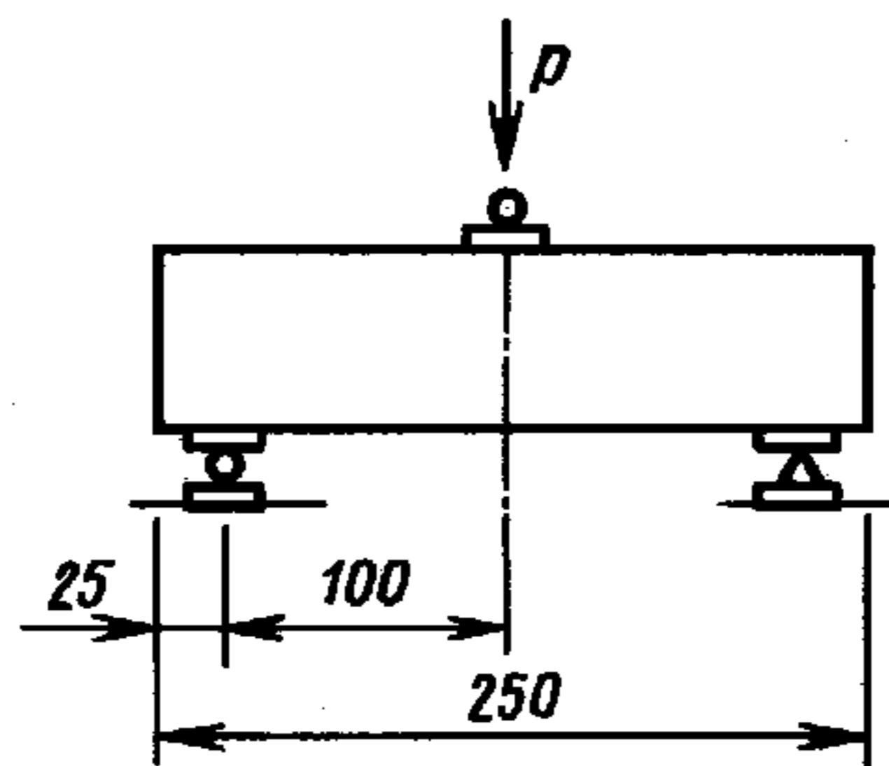
Схема испытания кирпича на изгиб
