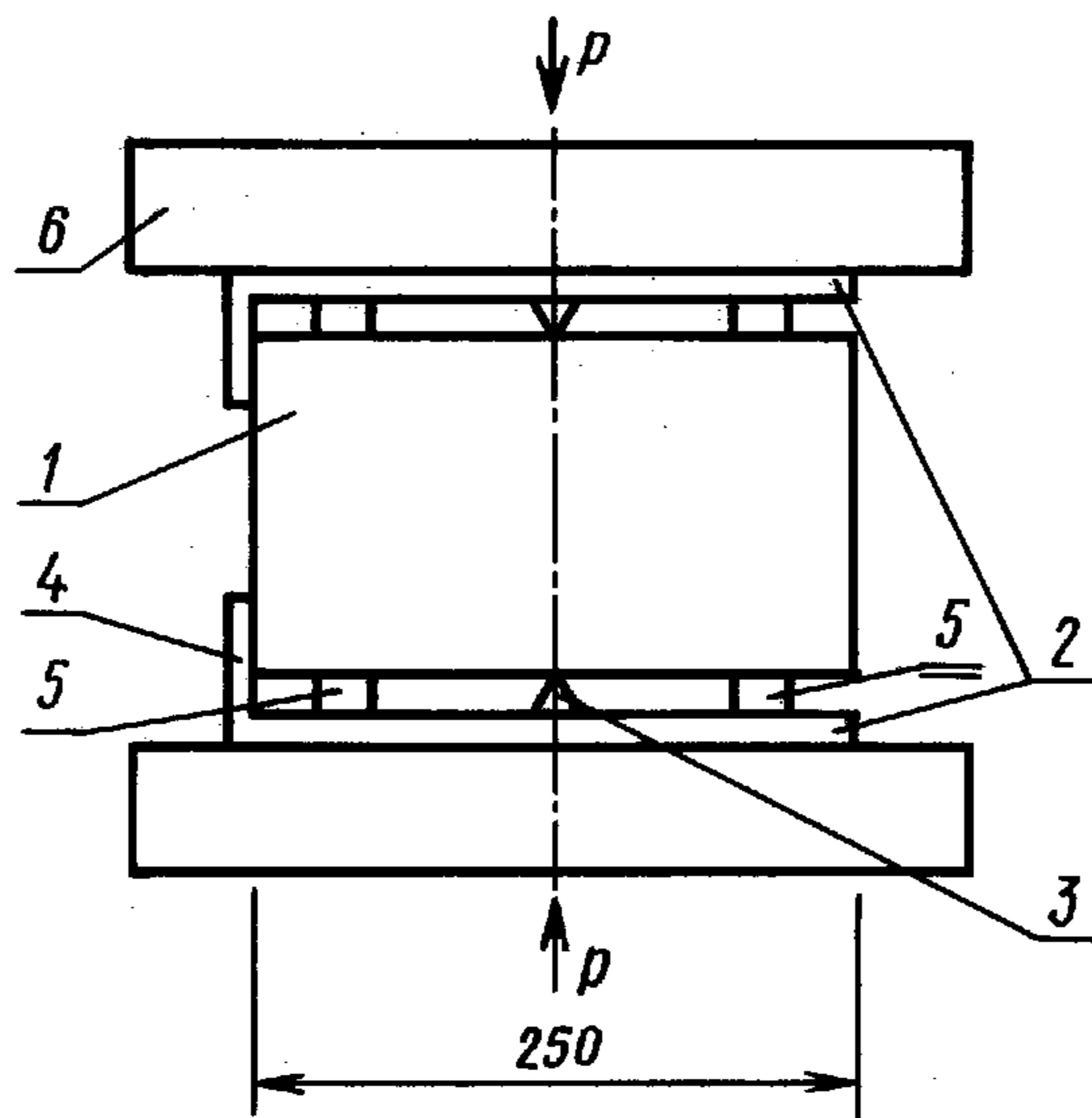
Схема раскладывания кирпича в прессе
