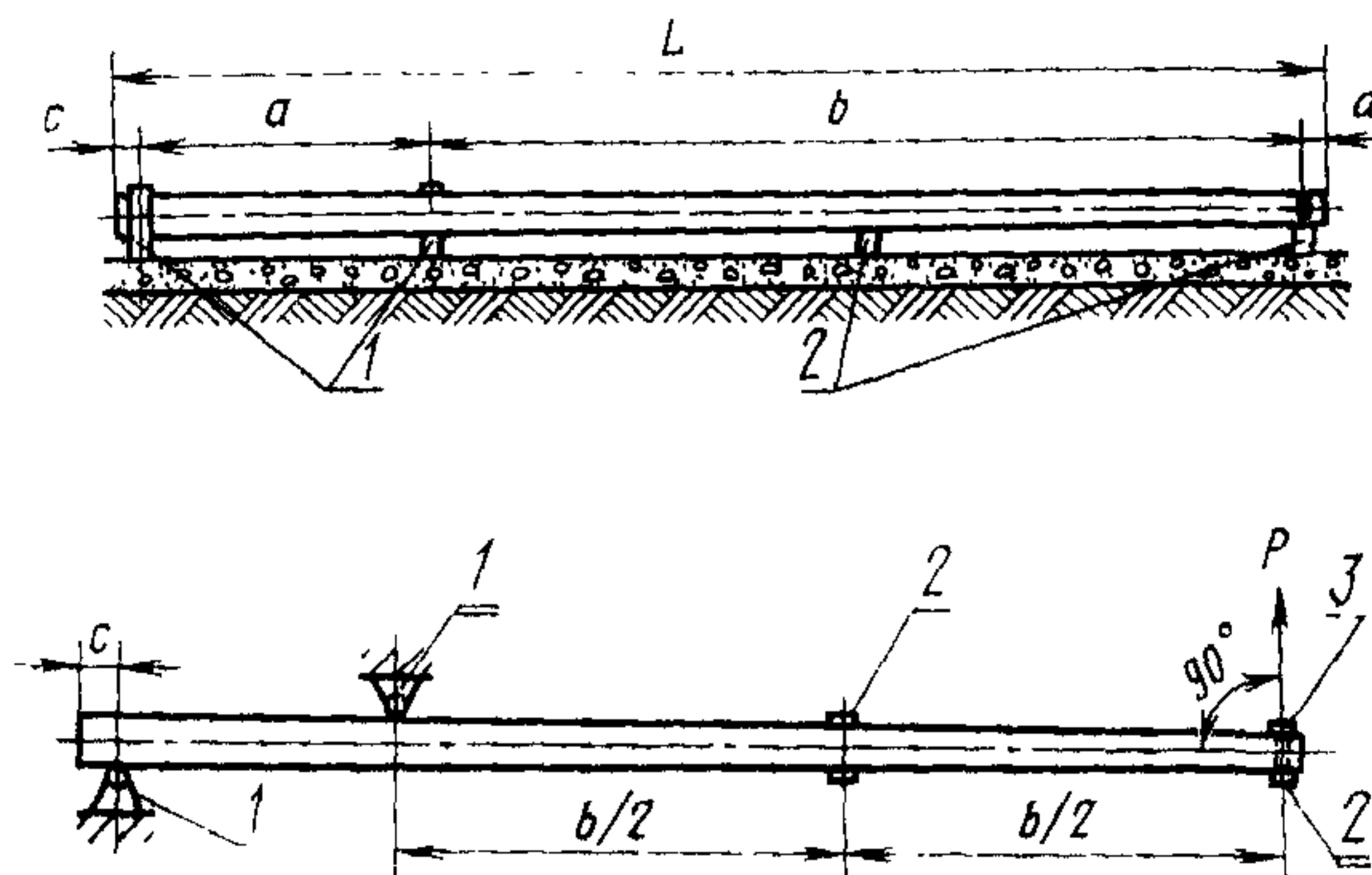
Схема испытания стоек
