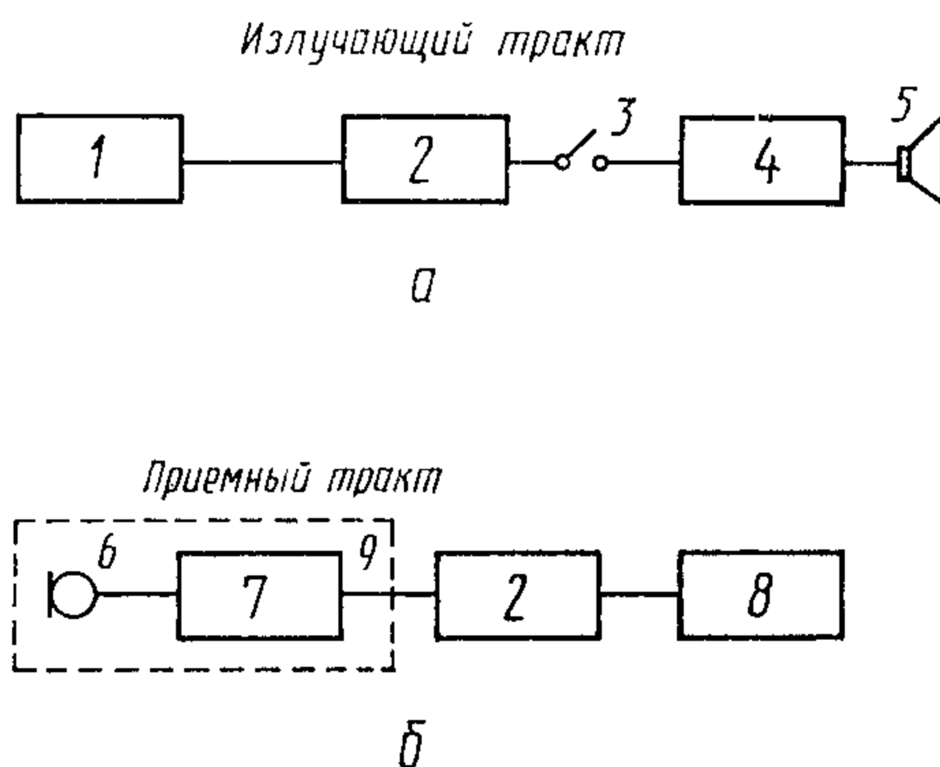
Блок-схема аппаратуры для измерения времени реверберации
