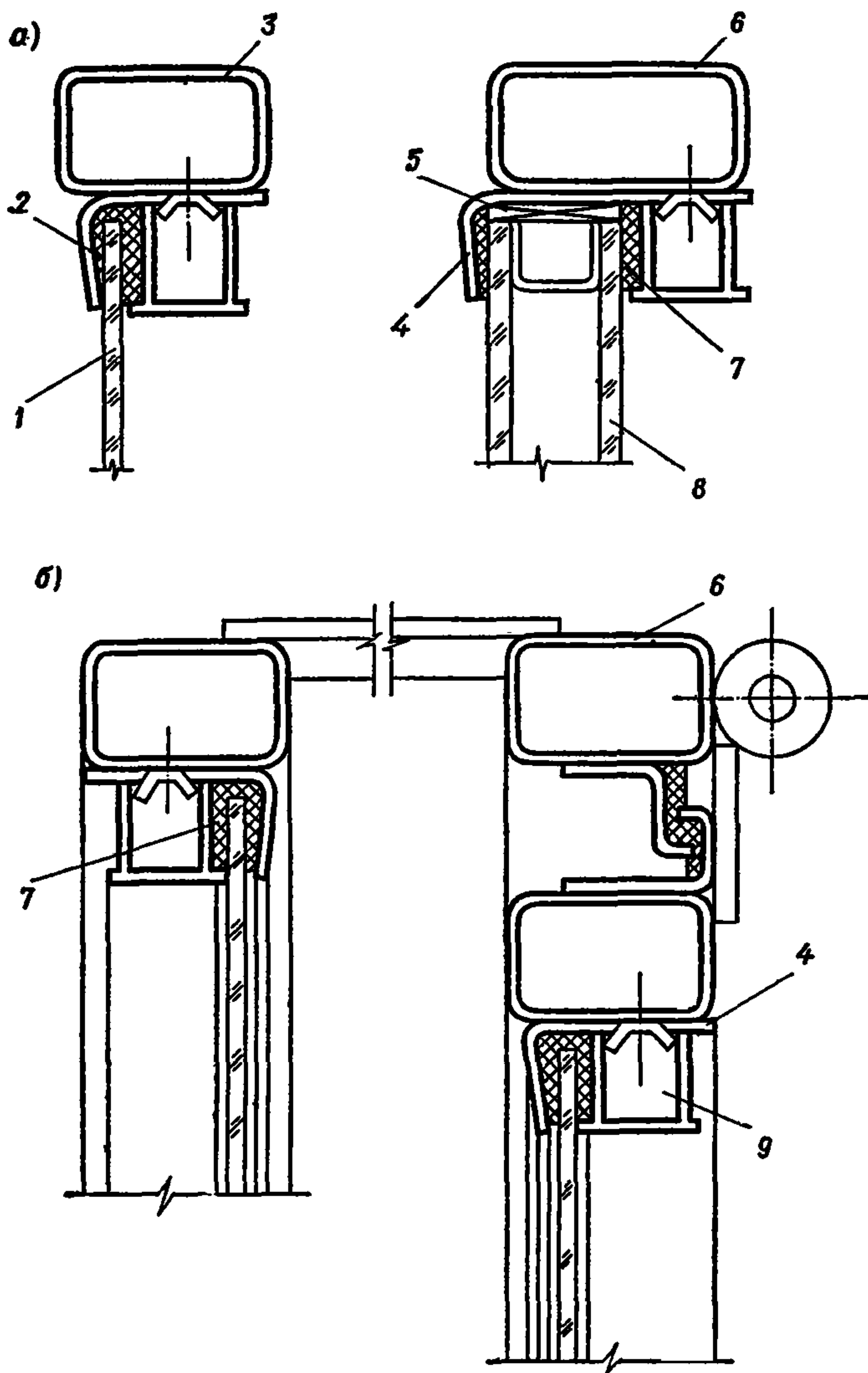
Рис. 3. Схемы сечений переплетов при остеклении
