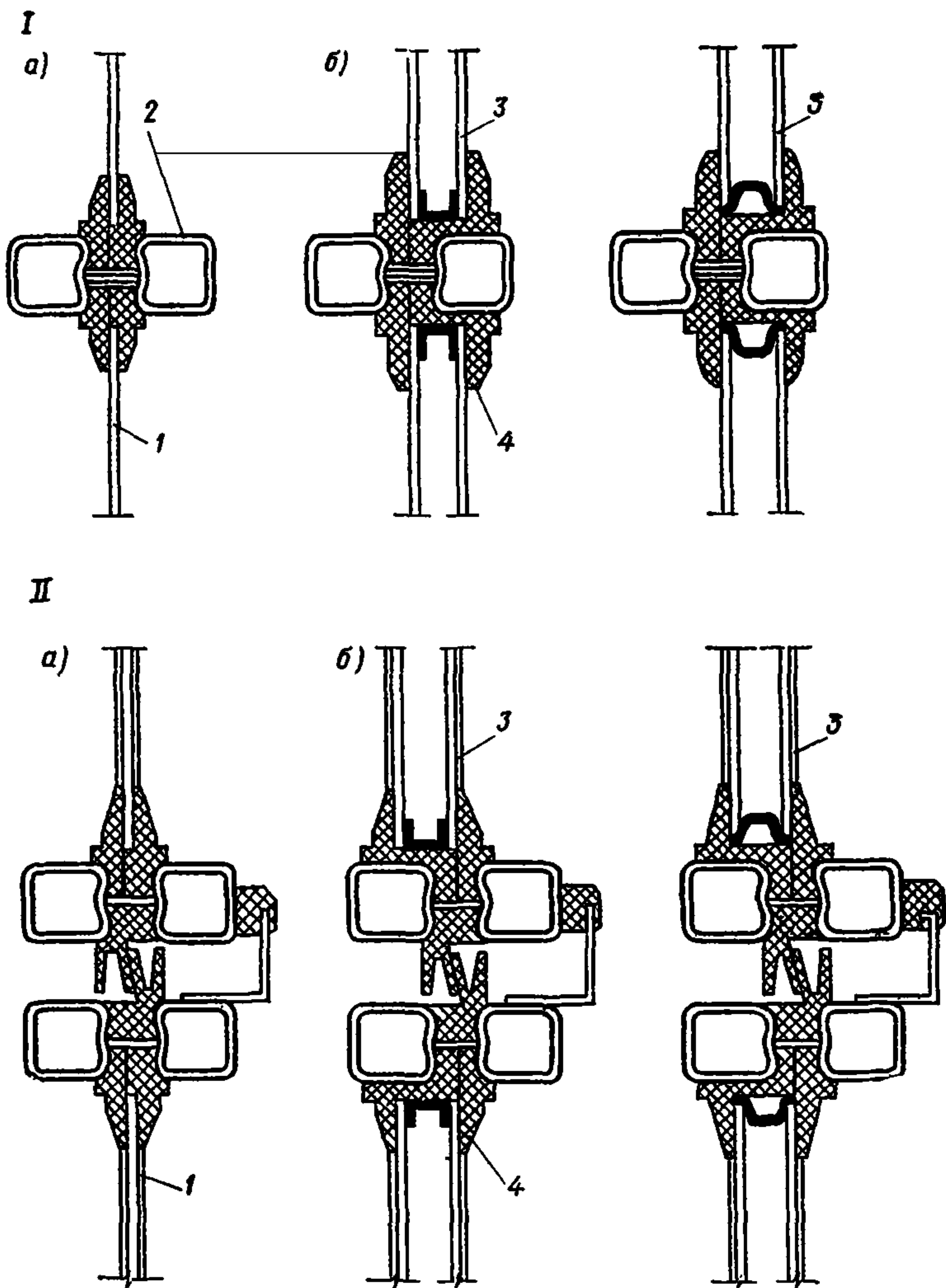
Рис. 2. Схемы сечений переплетов без фрамуг (I) и с фрамугами (II) при остеклении a — одинарном; б — двойном; 1 — стекло; 2 — профиль переплета; 3 — стекло-пакет; 4 — резиновый профиль
