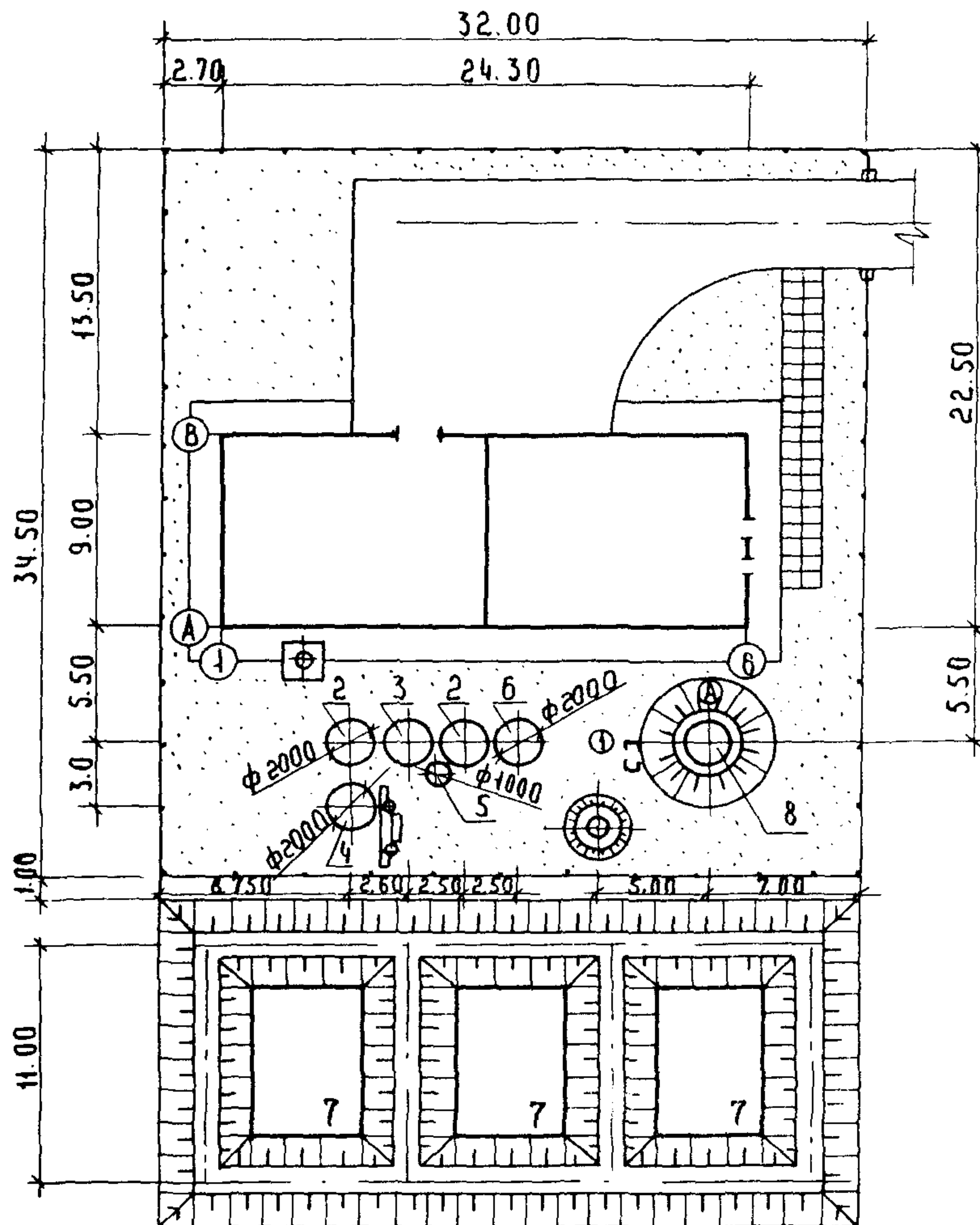
ПЛАН СТАНЦИИ
