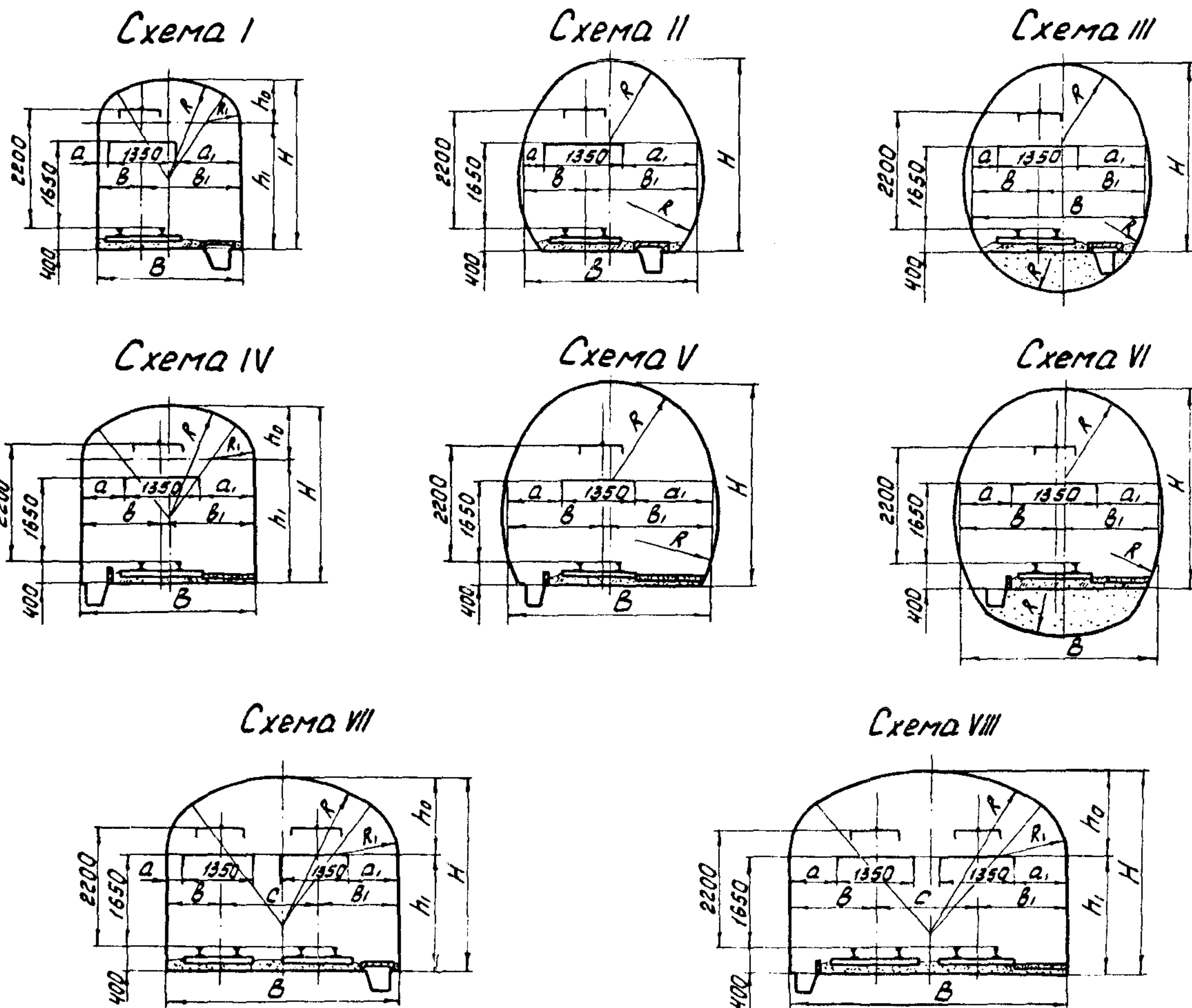
Конструктивные размеры сечений выработок
