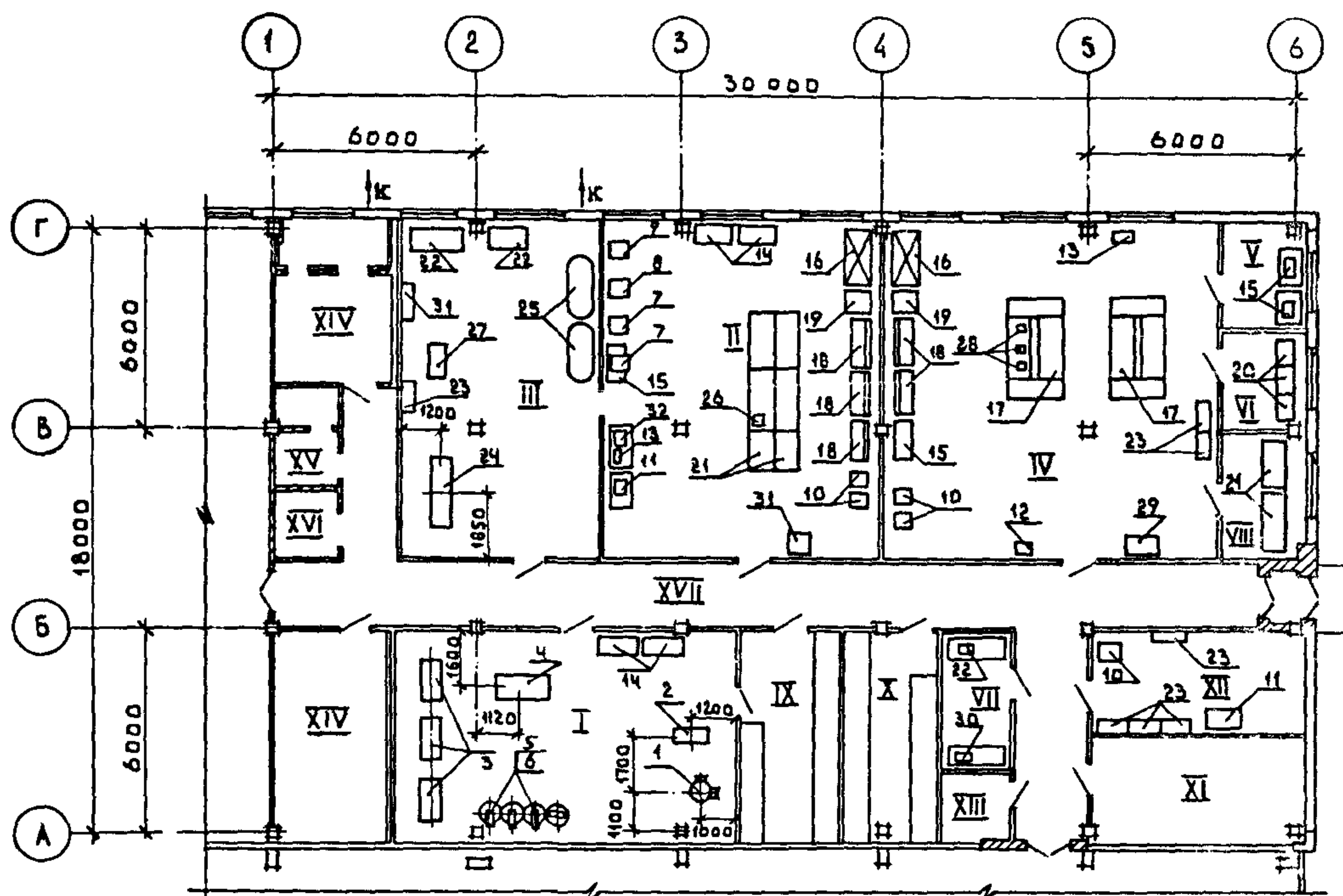
ЭКСПЛИКАЦИЯ ПОМЕЩЕНИЙ
