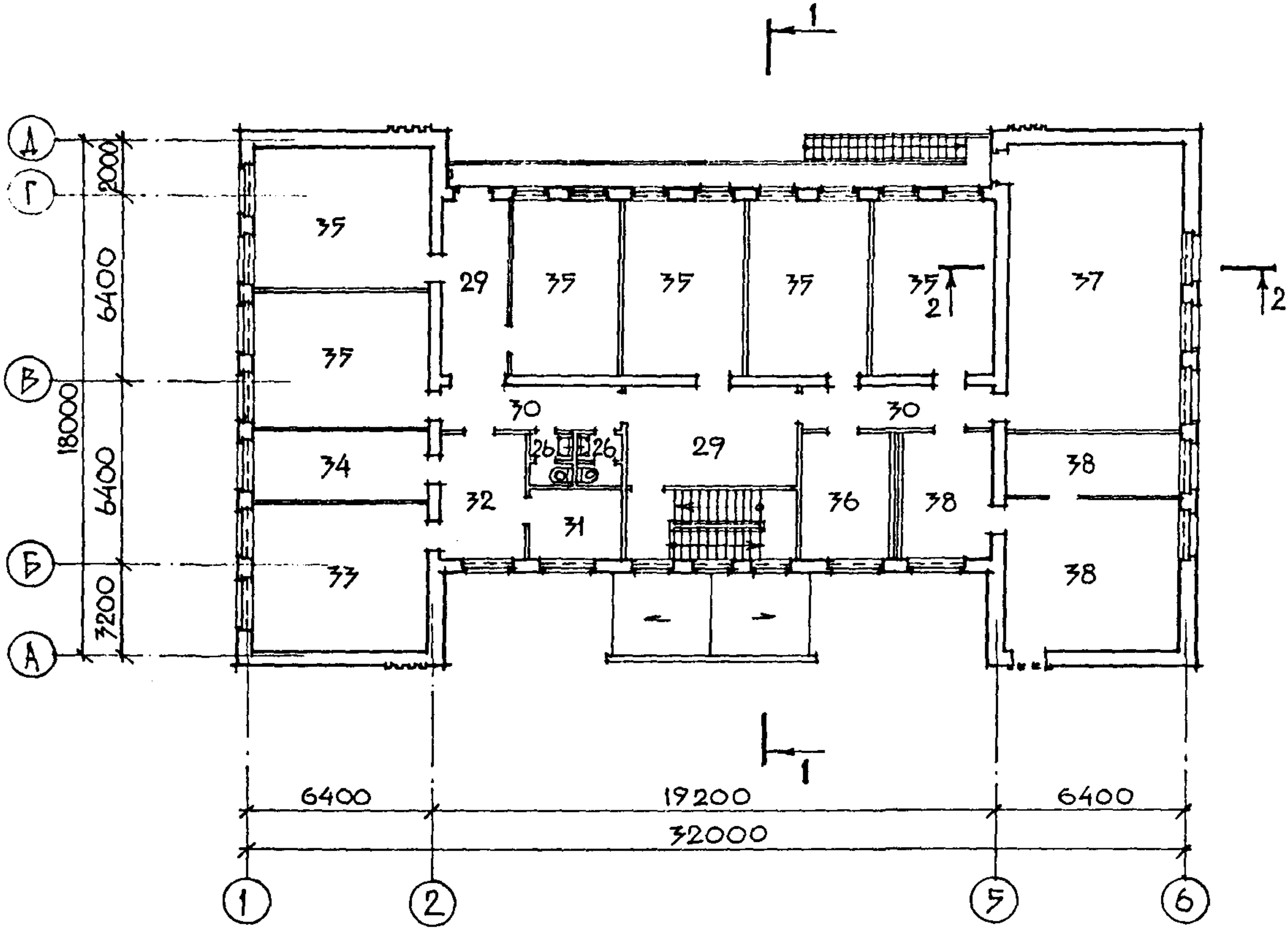
ПЛАН НА ОТМ. 3.300
