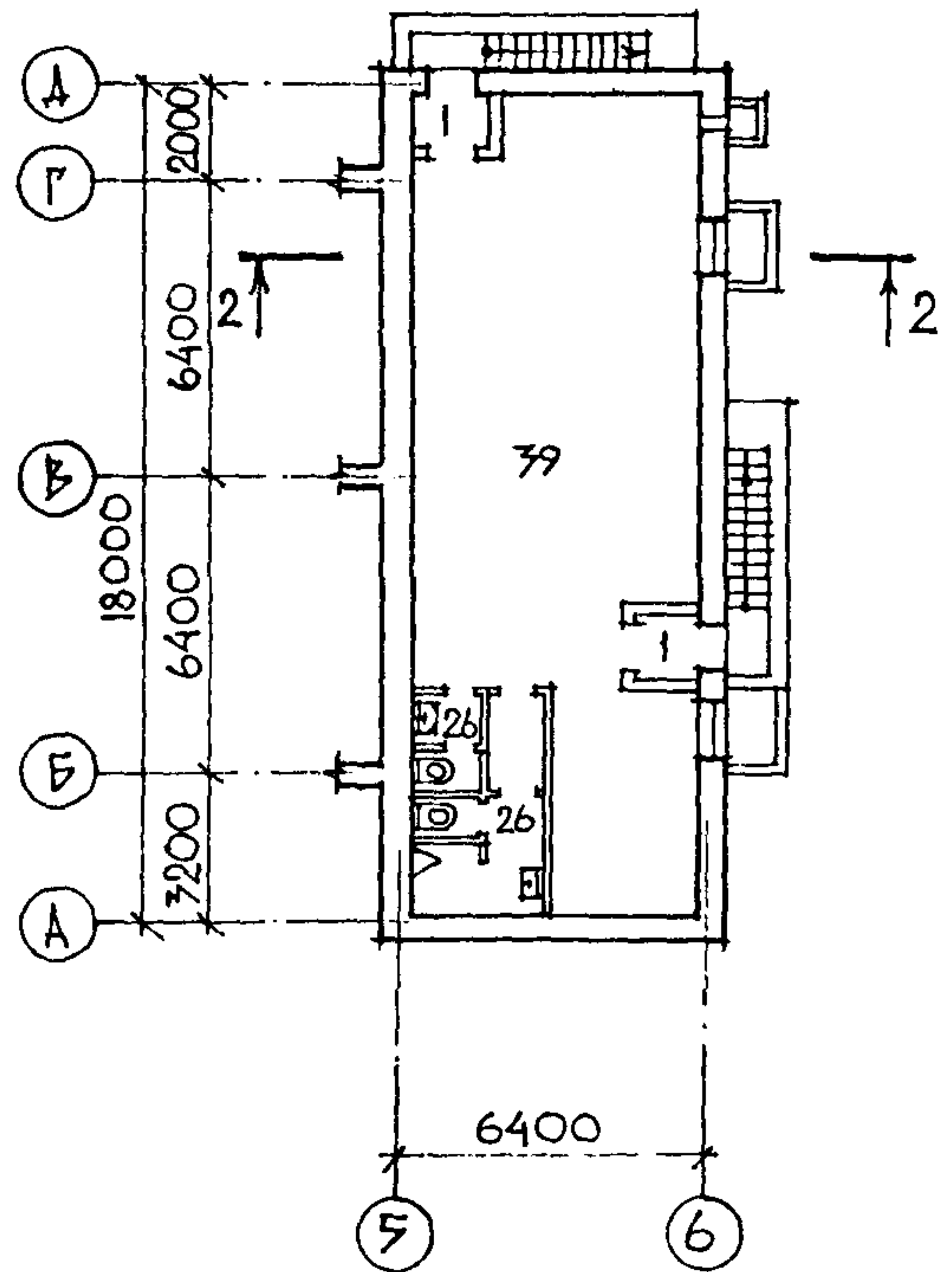
ПЛАН НА ОТМ. -2.450 /вариант с подсобными помещениями/
