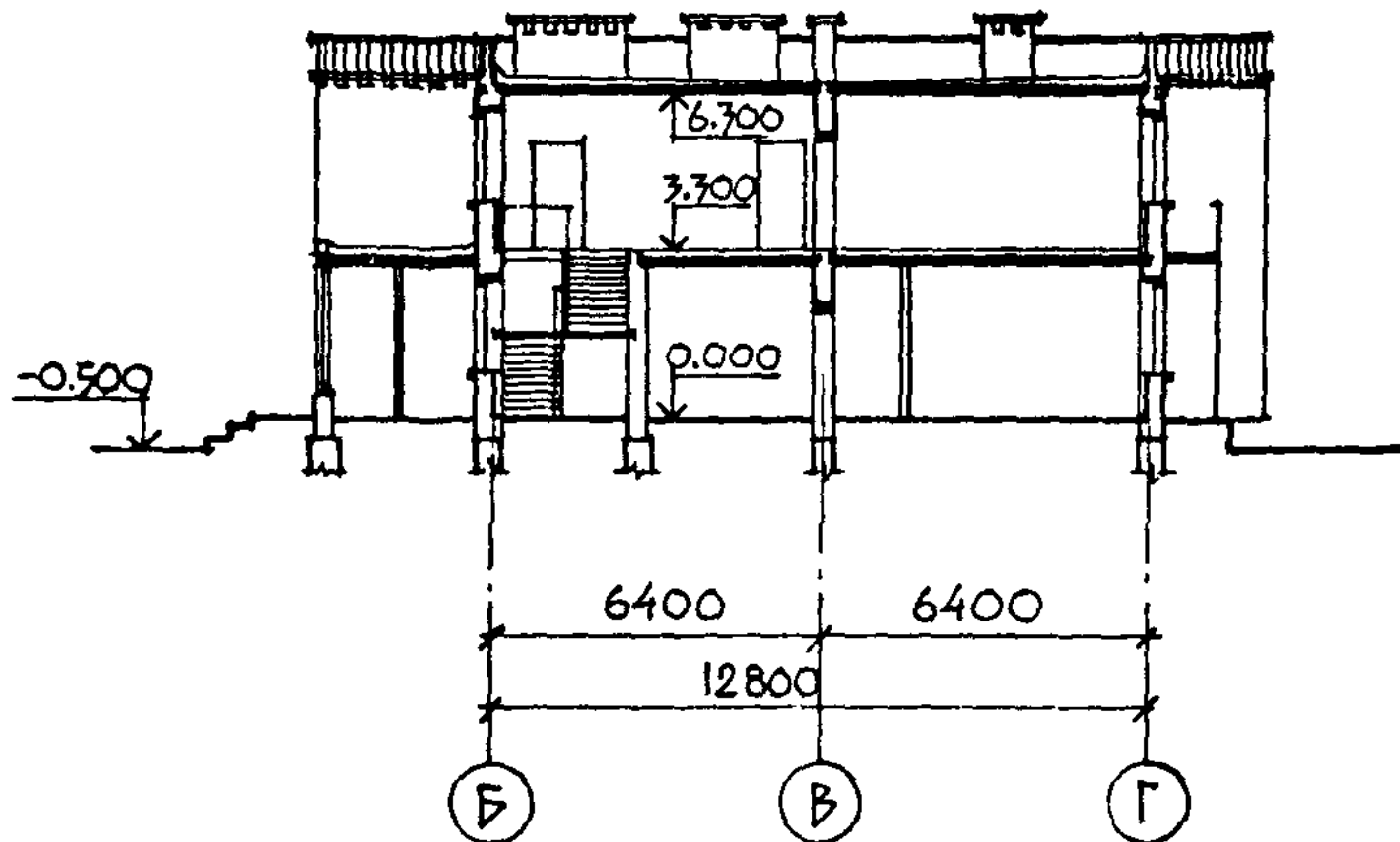
РАЗРЕЗ I-I
