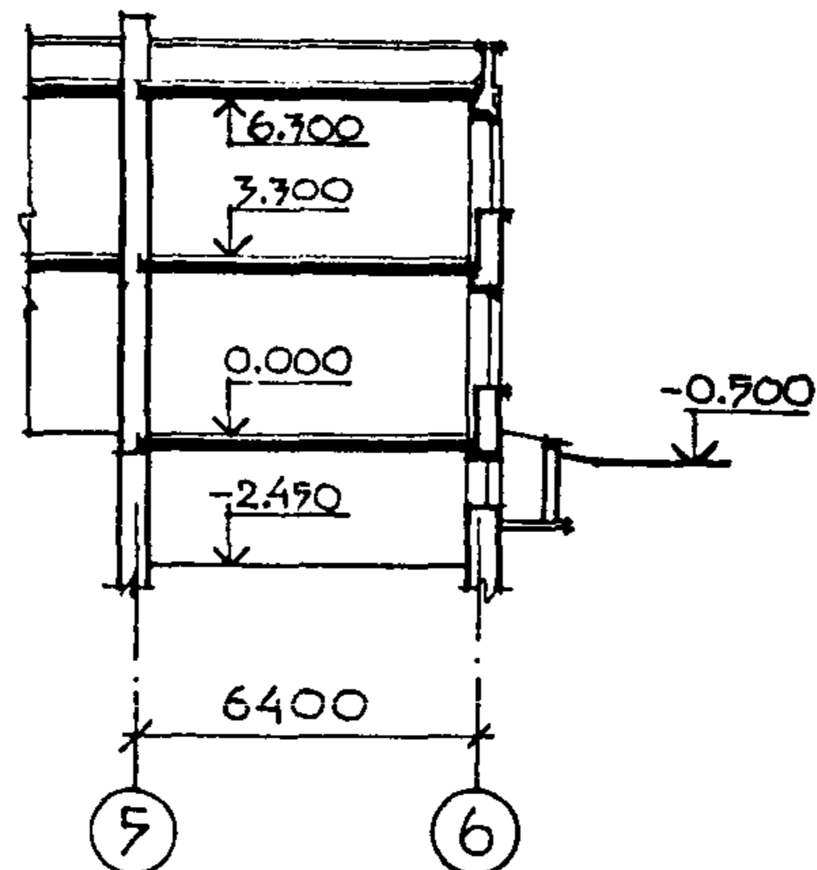
РАЗРЕЗ 2-2
