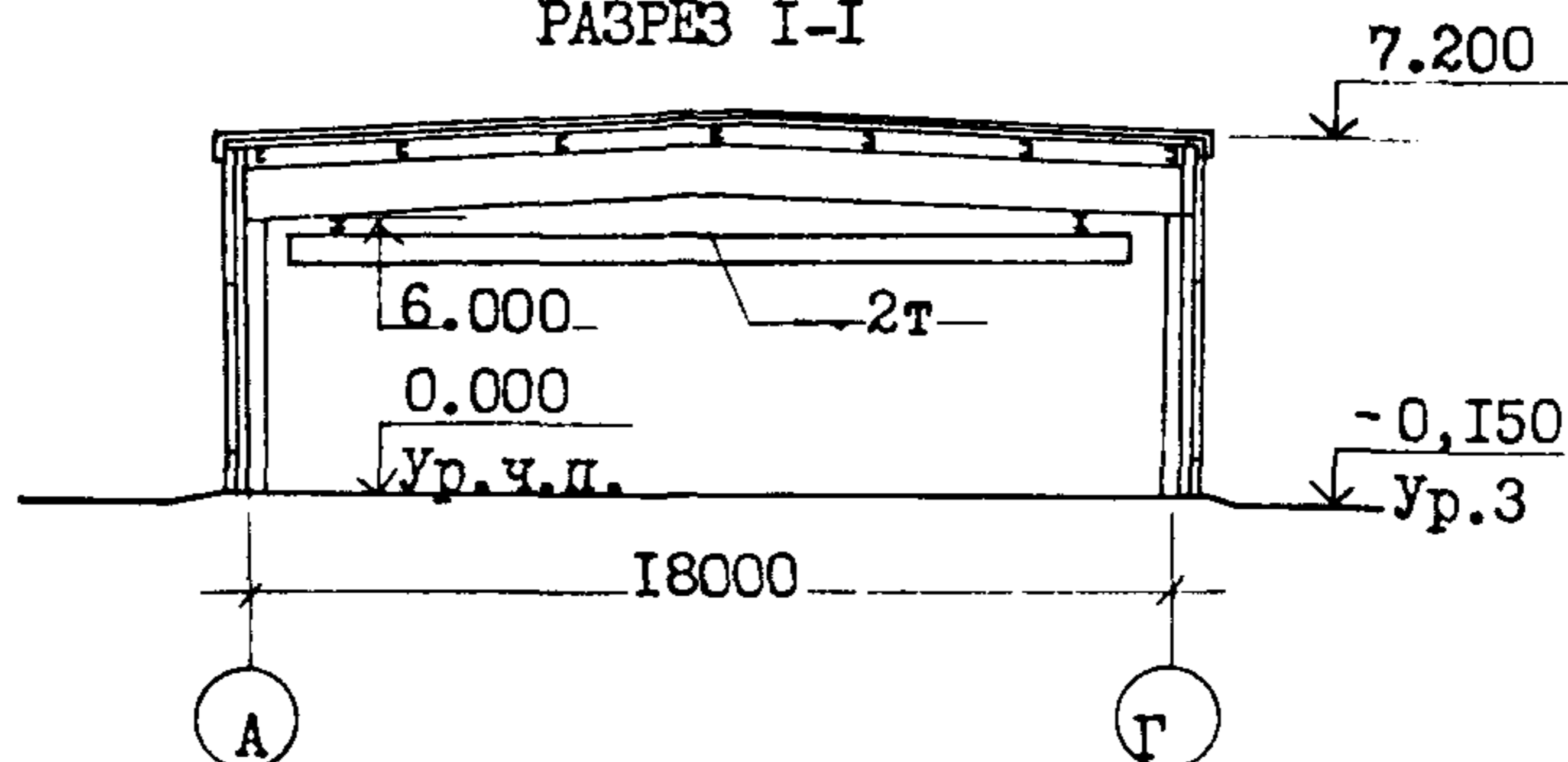
РАЗРЕЗ I-I
