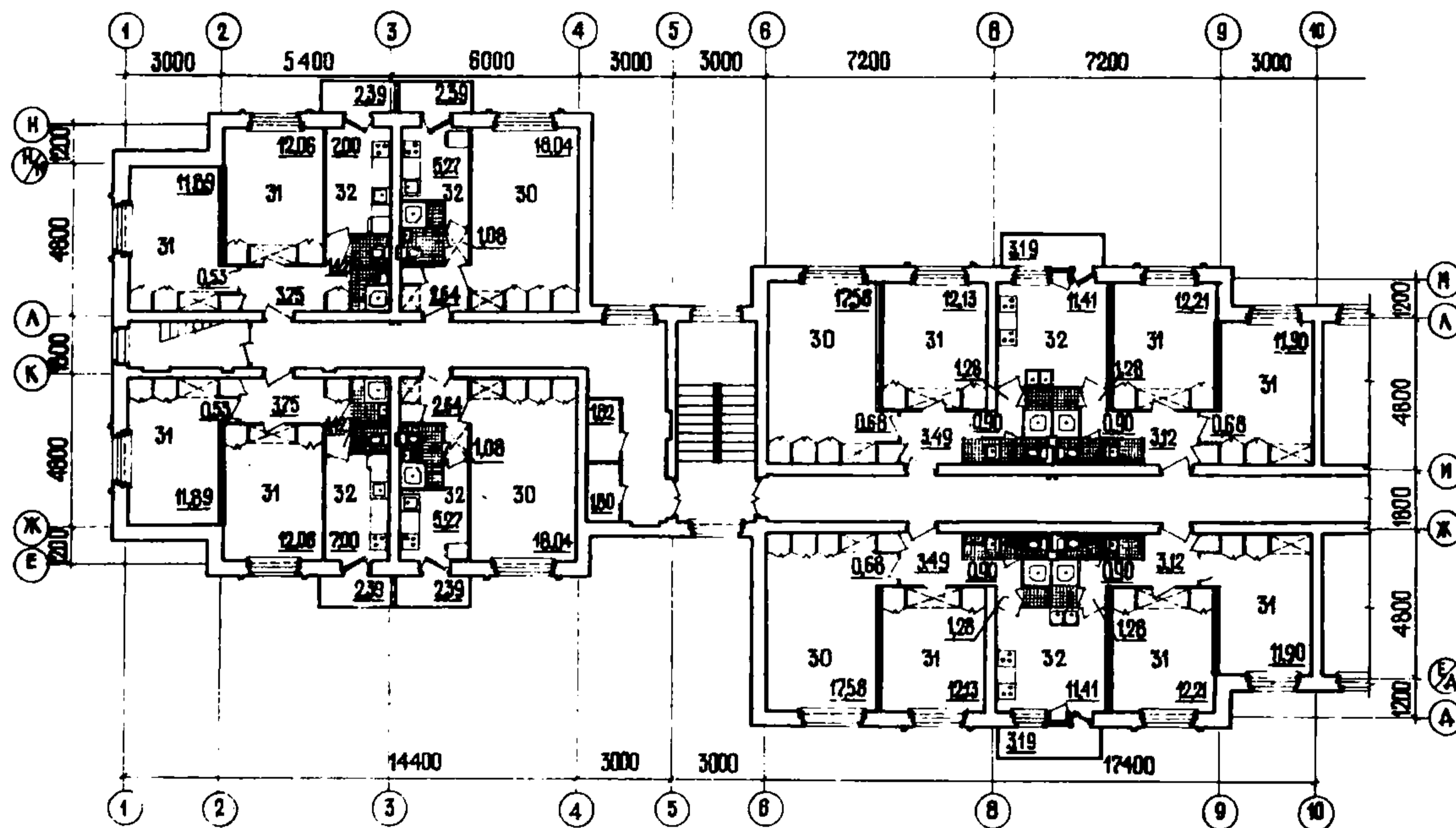
ФРАГМЕНТ ПЛАНА ТИПОВОГО ЭТАЖА
