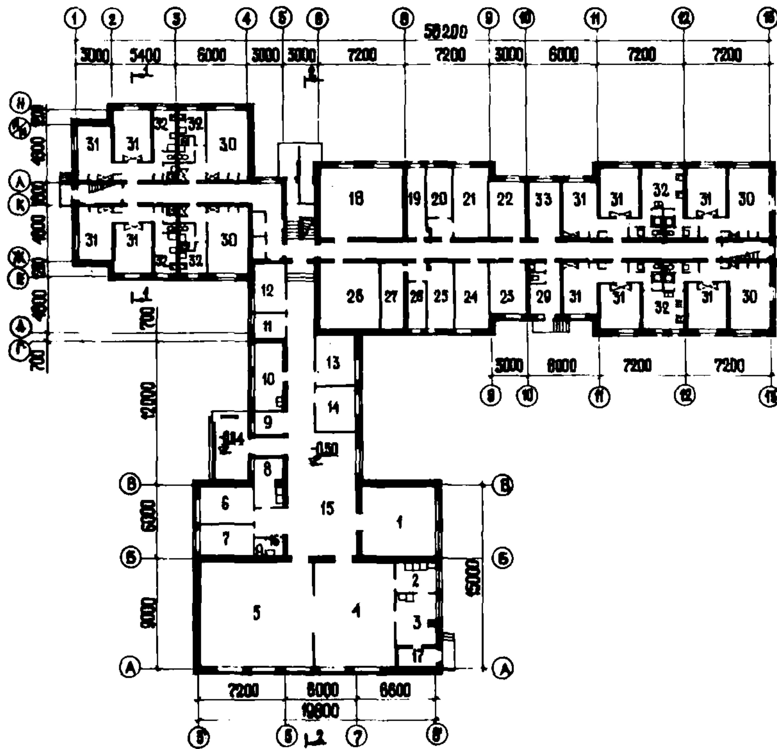
ПЛАН ПЕРВОГО ЭТАЖА
