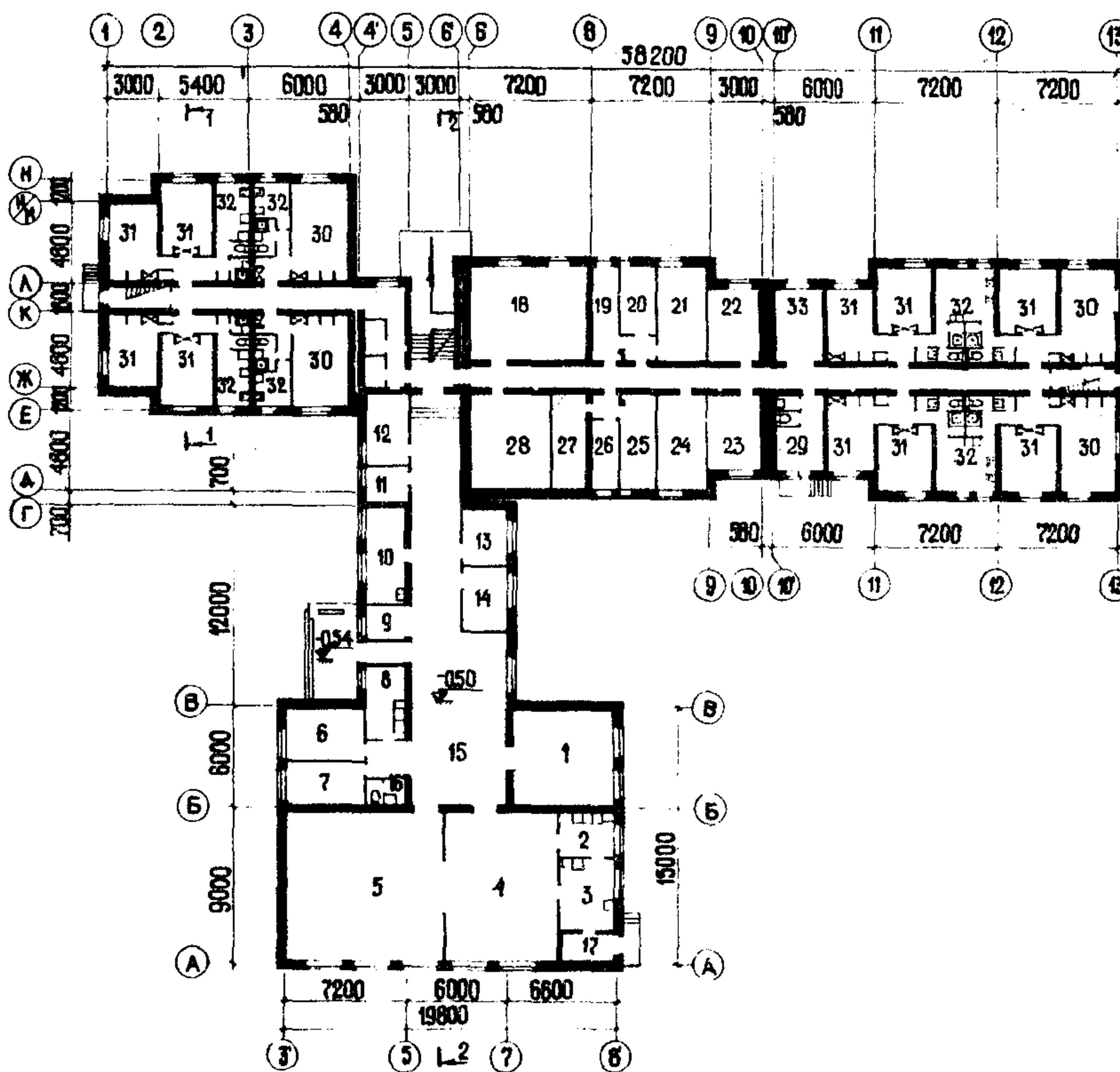
ПЛАН ПЕРВОГО ЭТАЖА
