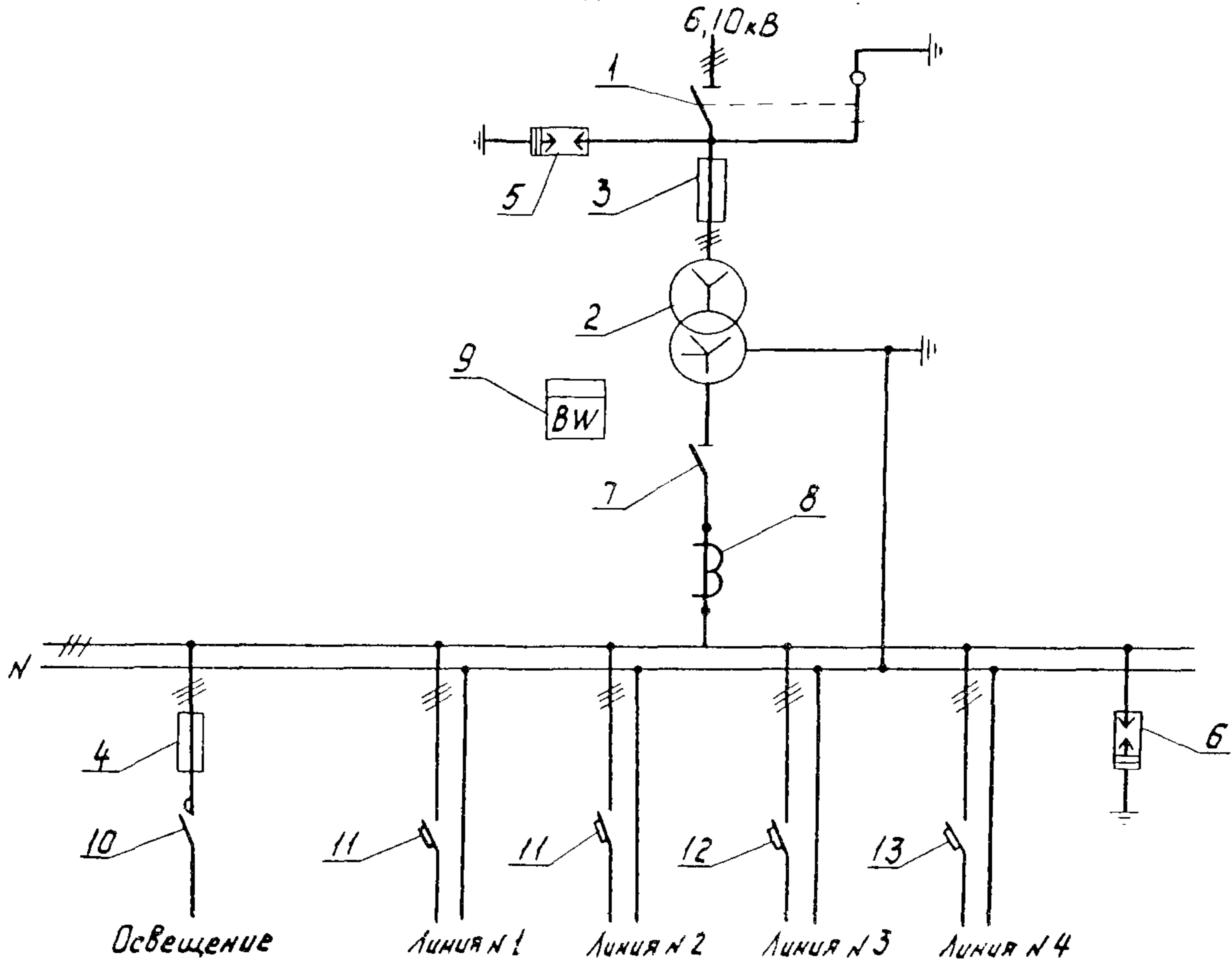
СХЕМА ЭЛЕКТРИЧЕСКИХ СОЕДИНЕНИЙ ПОДСТАНЦИИ
