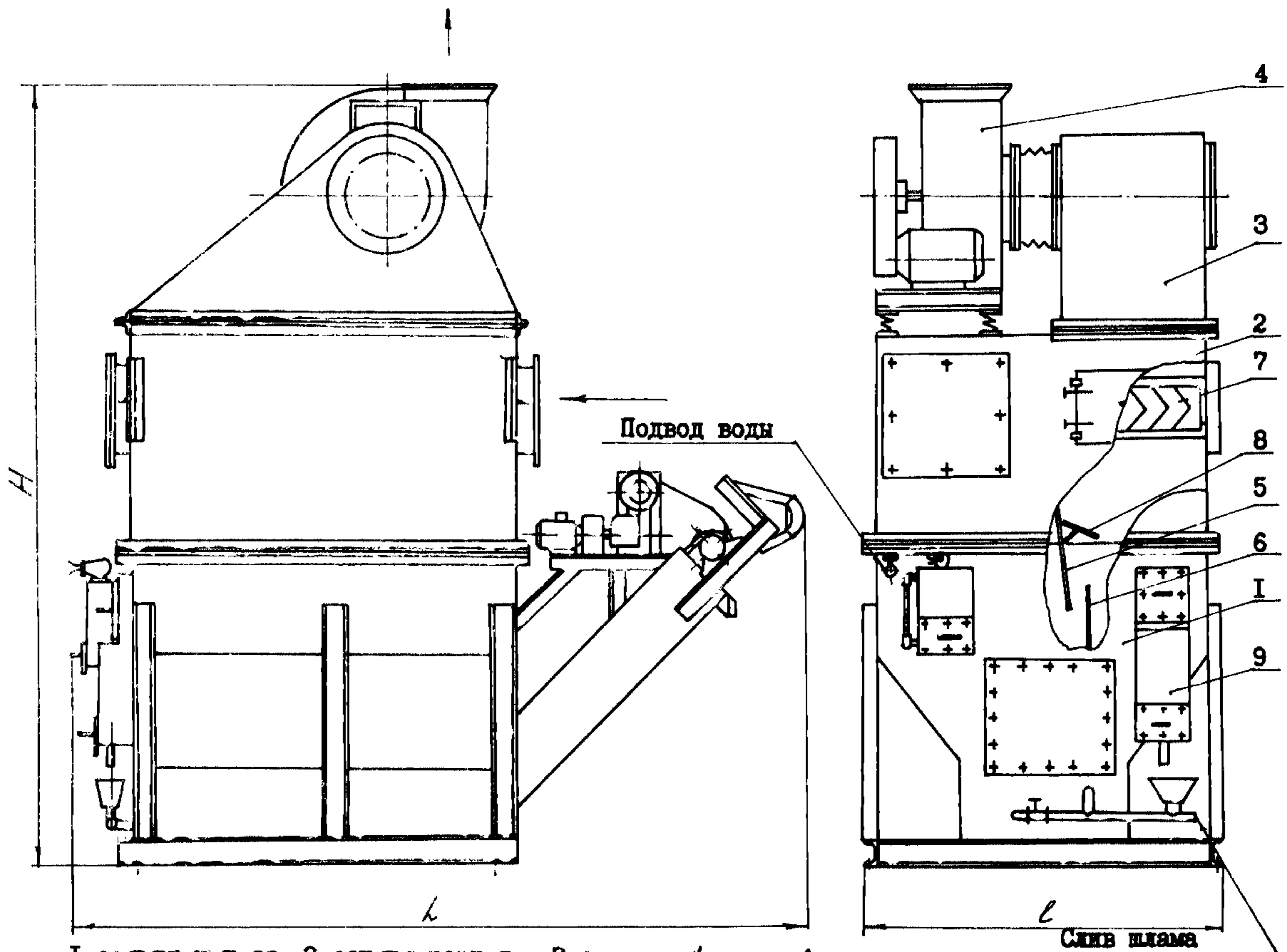
1-секция нижняя, 2-секция верхняя, 3-воздухосборник, 4-вентнагреват., 5-подъемная перегородка, 6-поддонная перегородка, 7-капельловитель, 8-конвейер, 9-лоток
