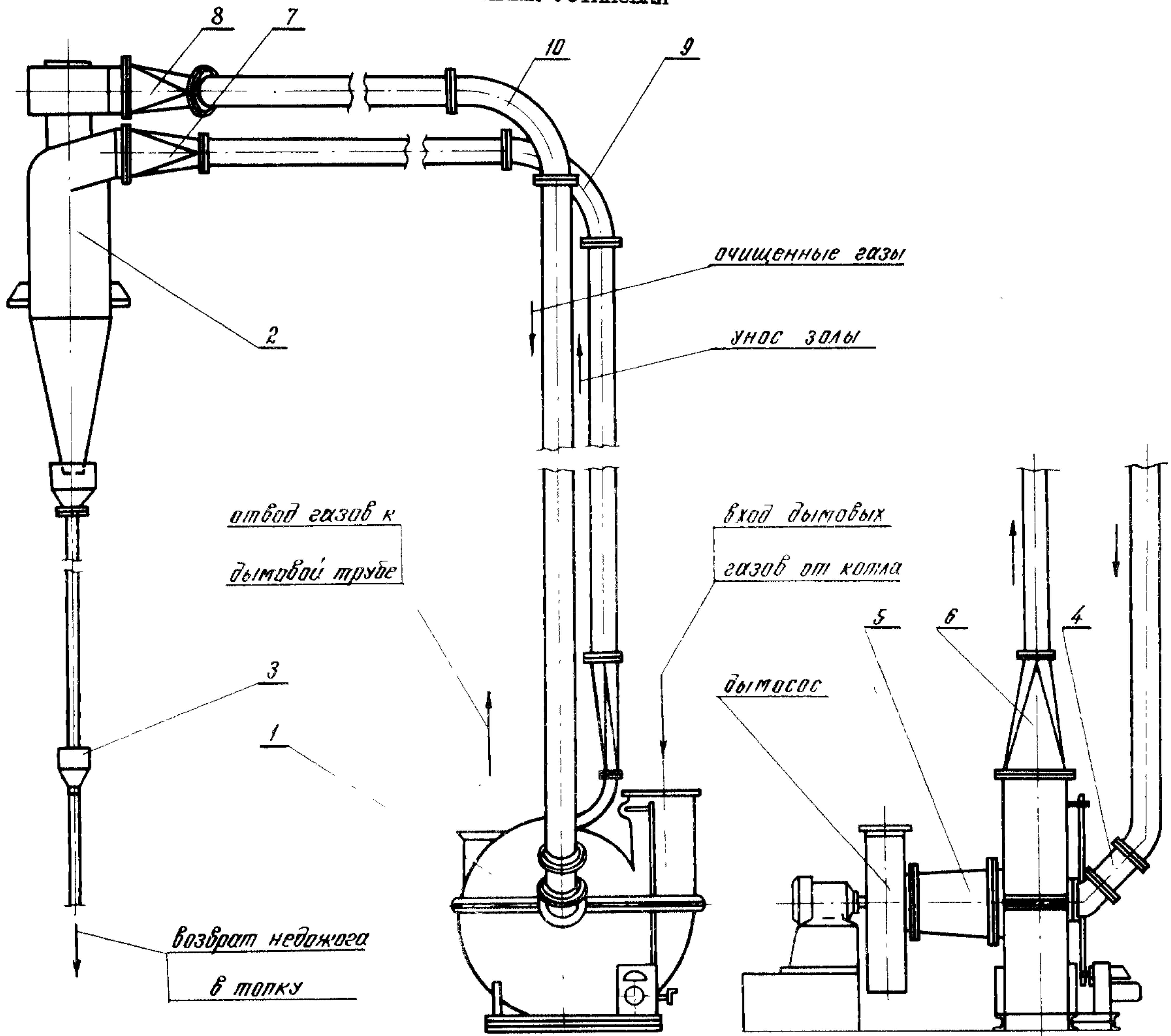
ЭКСПЛИКАЦИЯ ОБОРУДОВАНИЯ
