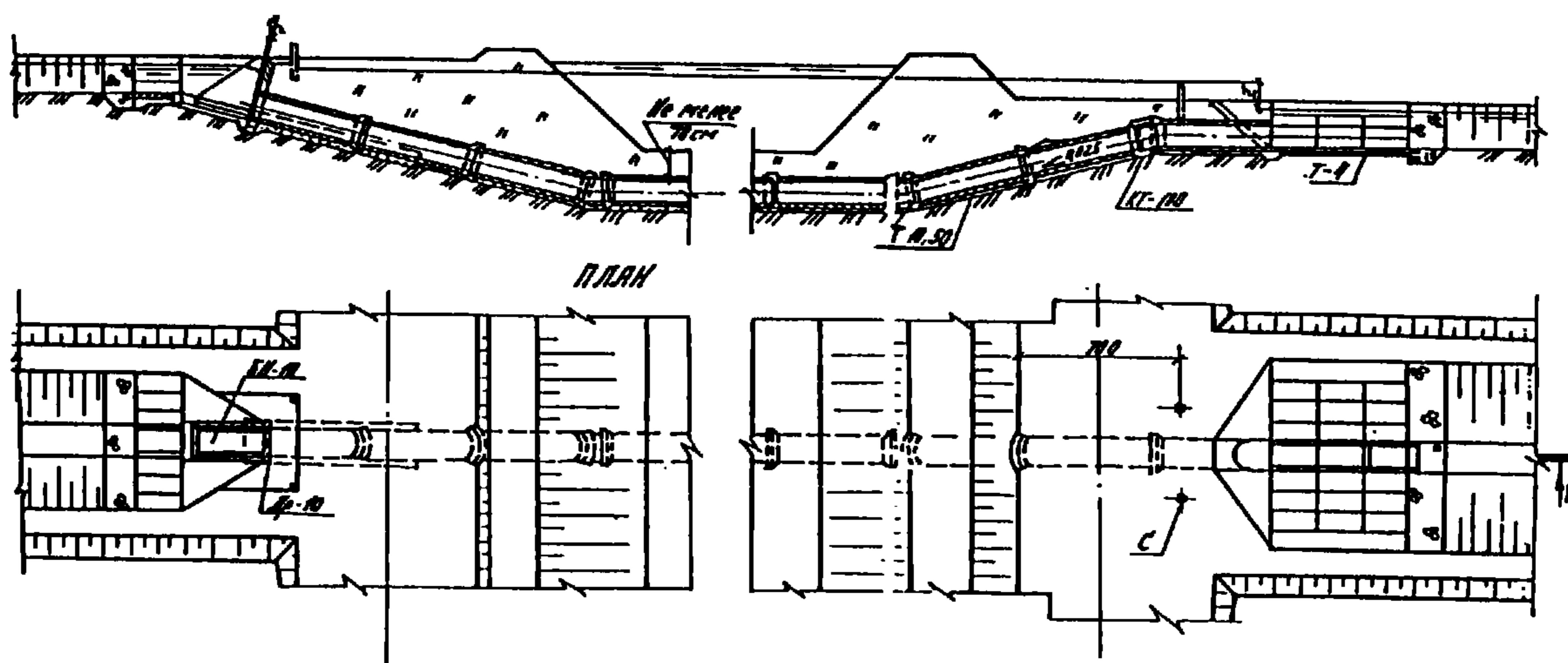
РАЗРЕЗ I-I
