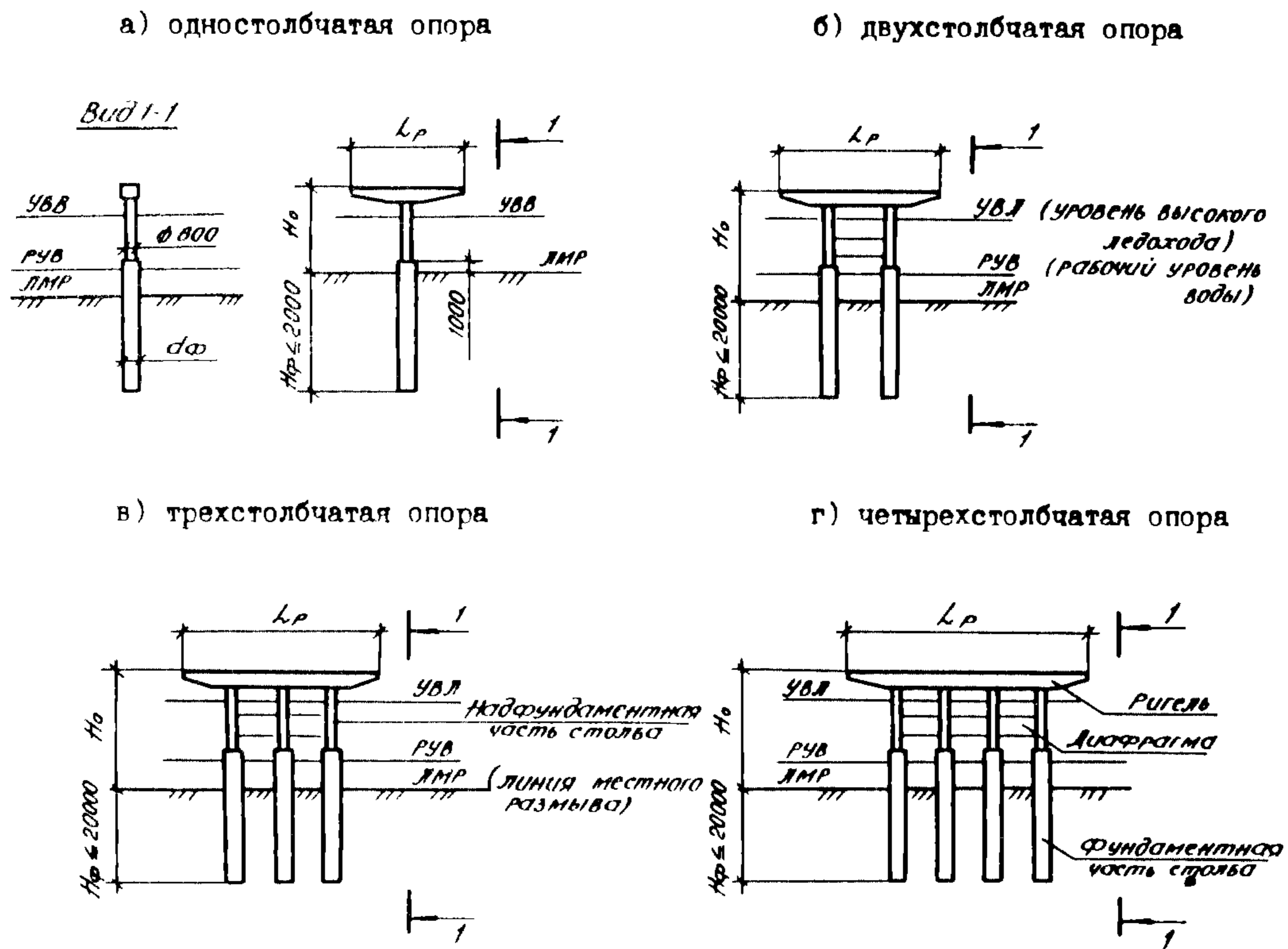
Рис.1 СХЕМЫ ПРОМЕЖУТОЧНЫХ ОПОР
