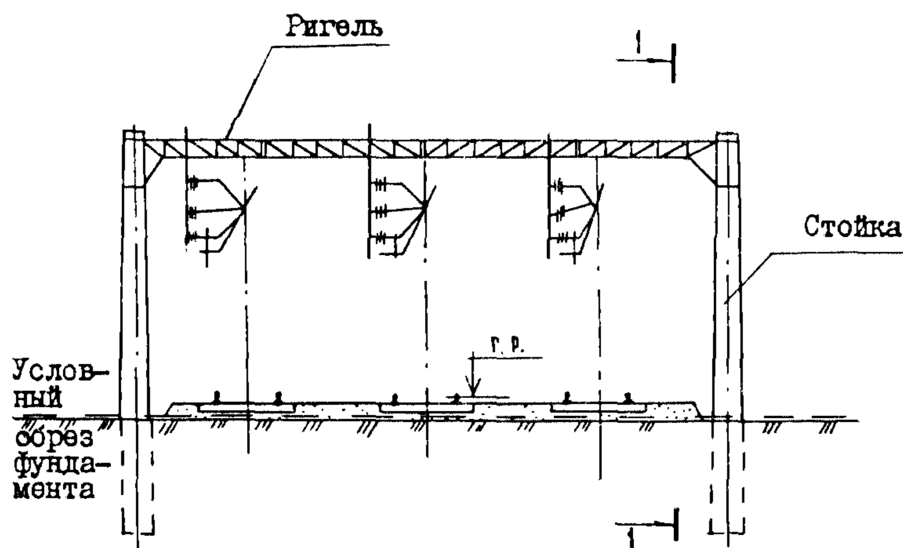
СХЕМА ПОПЕРЕЧИНЫ НА ПЕРЕГОНЕ
