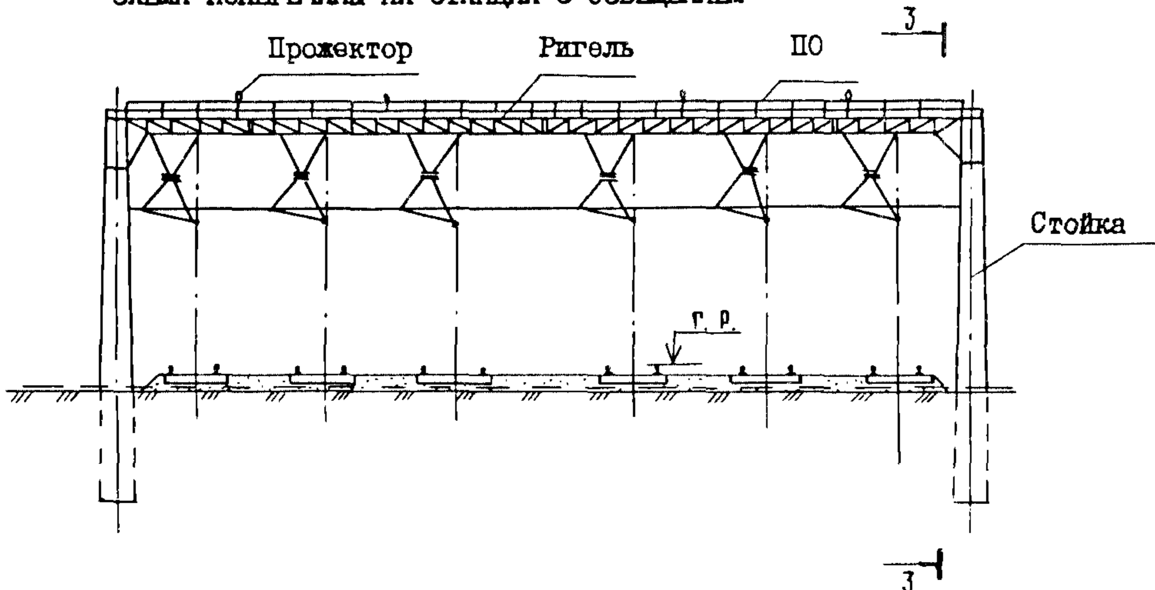
СХЕМА ПОПЕРЕЧИНЫ НА СТАНЦИИ С ОСВЕЩЕНИЕМ
