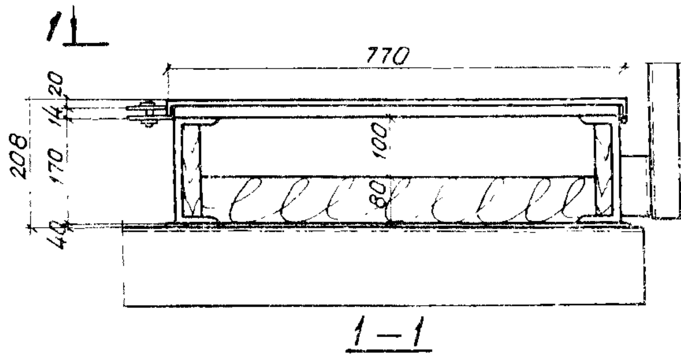
Металлический желоб
