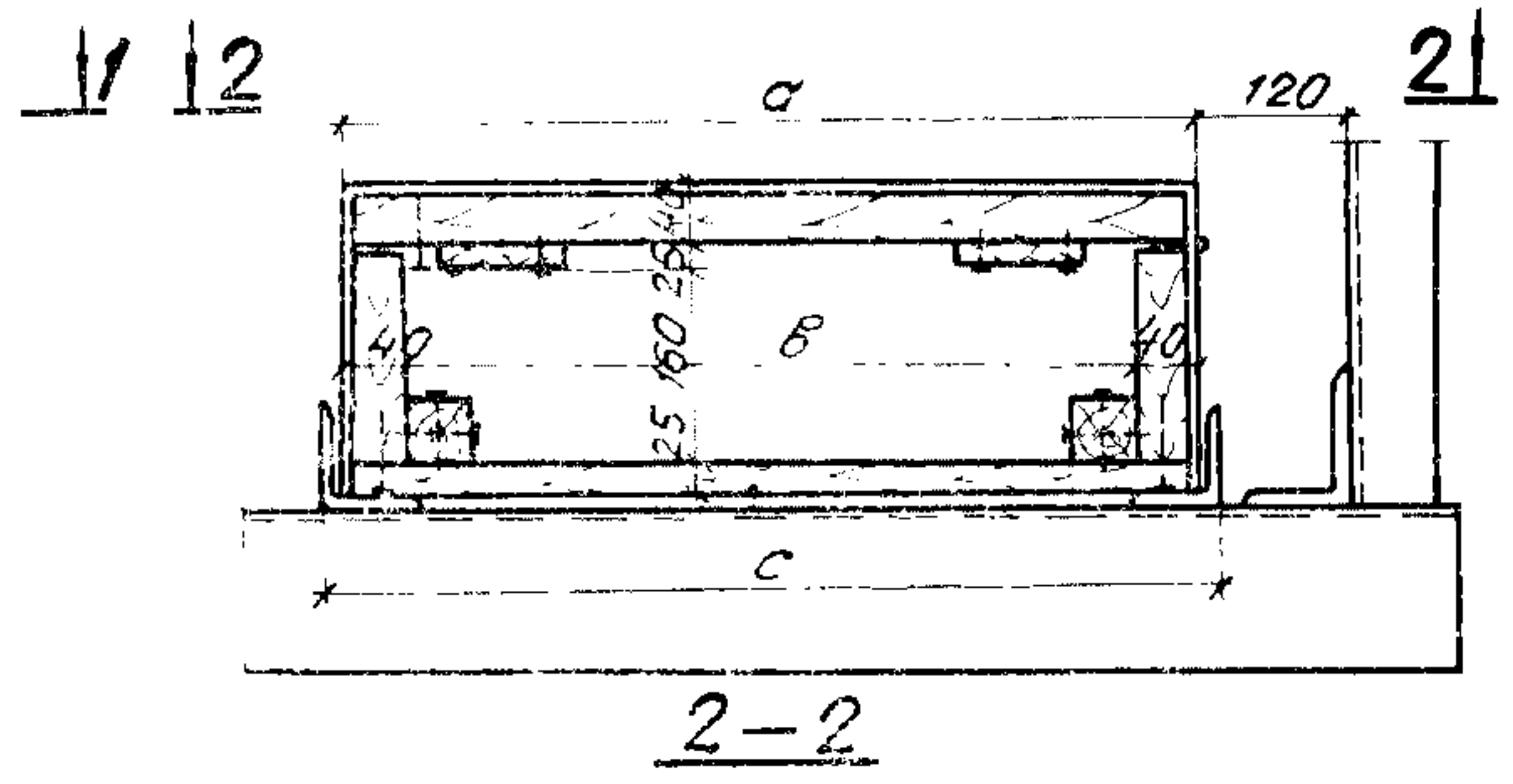
Деревянный желоб
