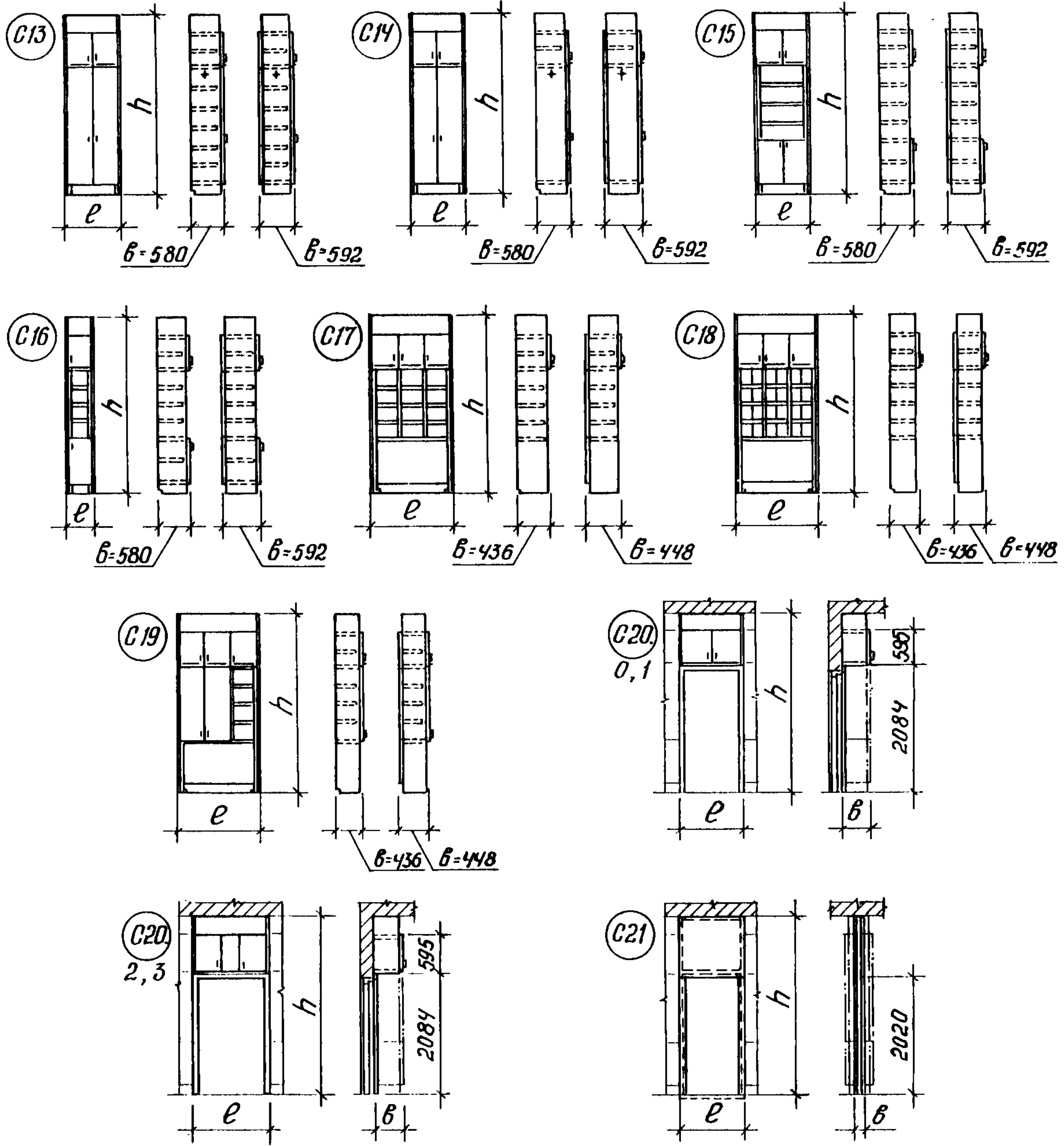
а) Встроенные шкафные отделения секций пристенных h=3,00 м под потолок
