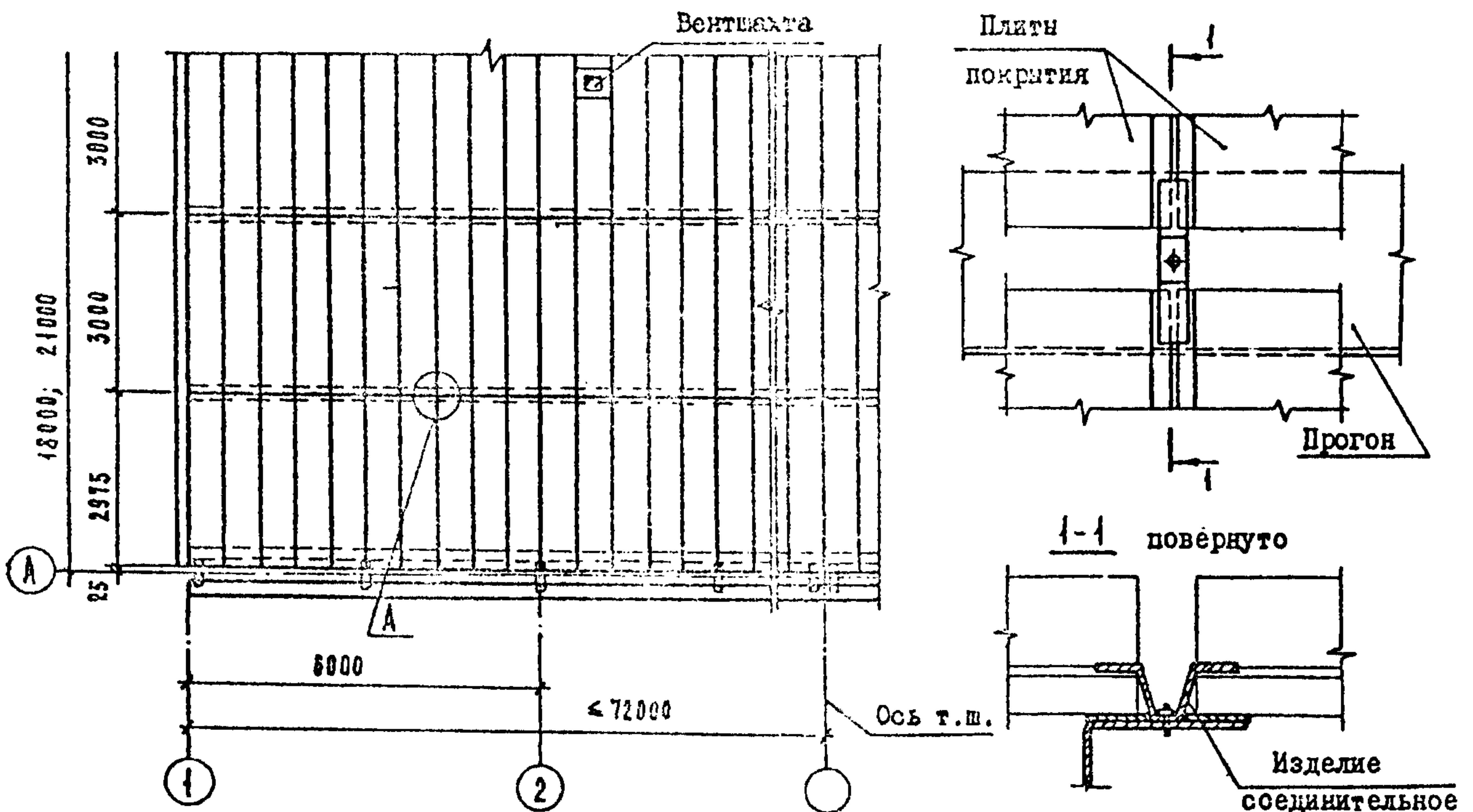
СХЕМА РАСПОЛОЖЕНИЯ ПЛИТ ПОКРЫТИЯ
