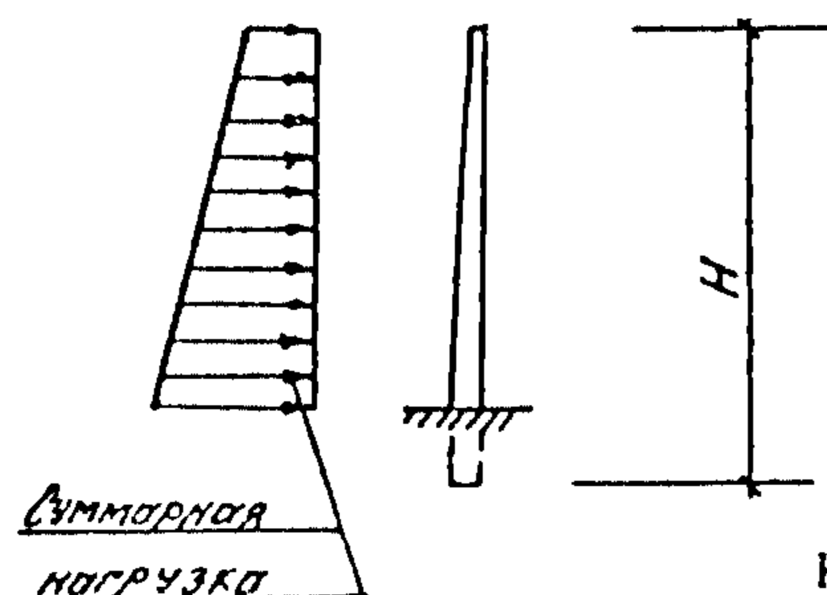
Расчетная схема панелей
