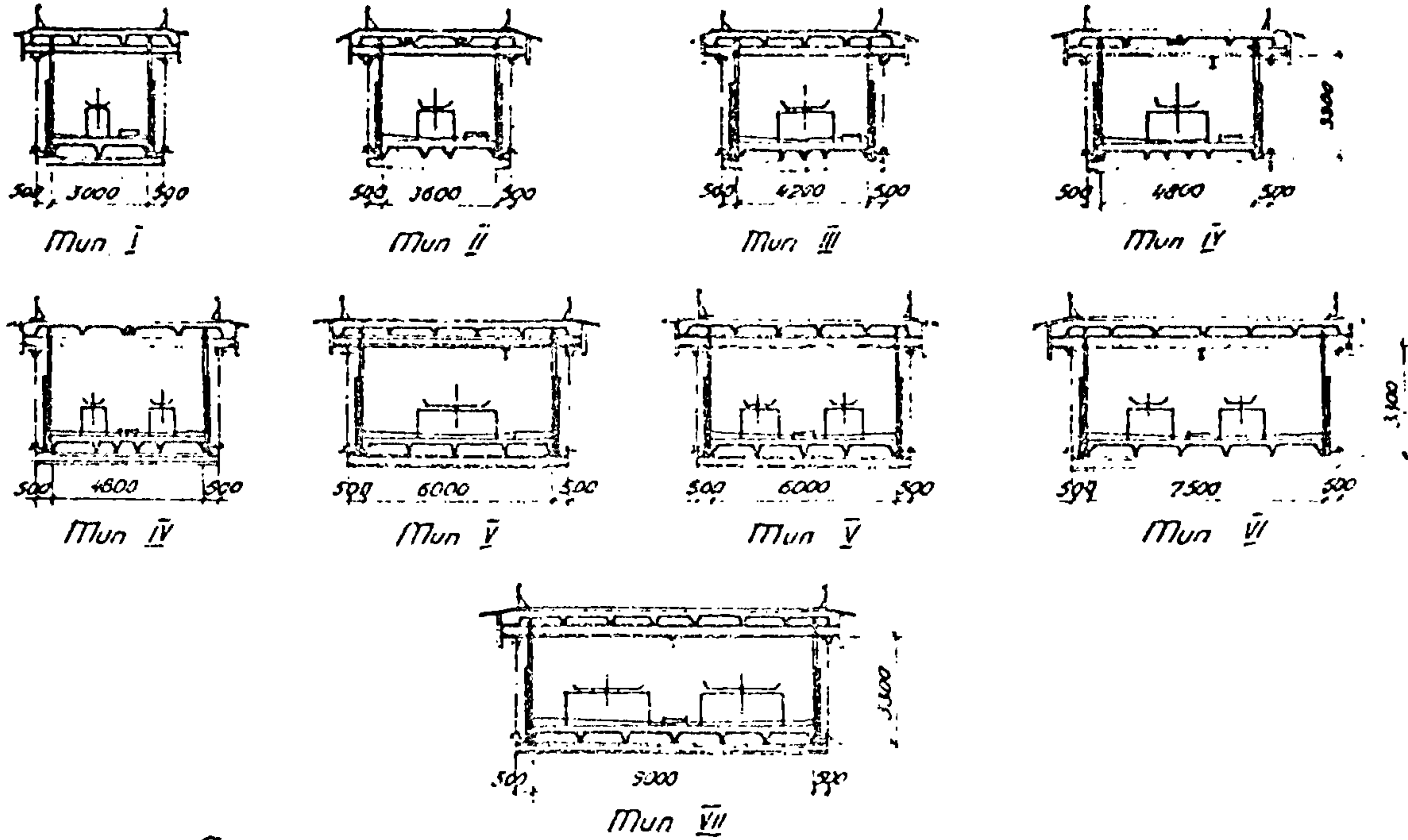
Схемы поперечных разрезов галерей
