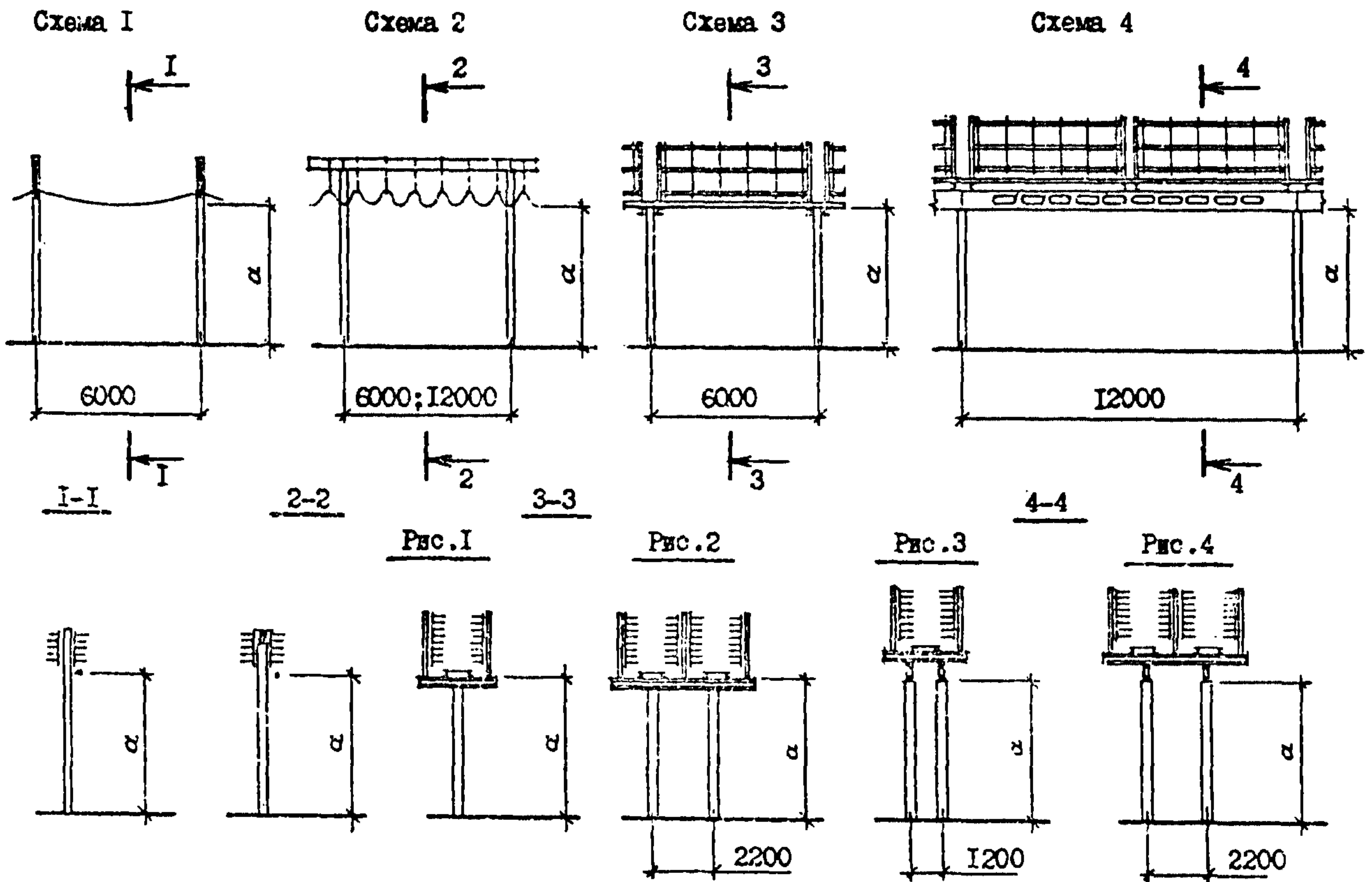
КЛЮЧ ПОДБОРА МАРКИ ЭСТАКАДЫ
