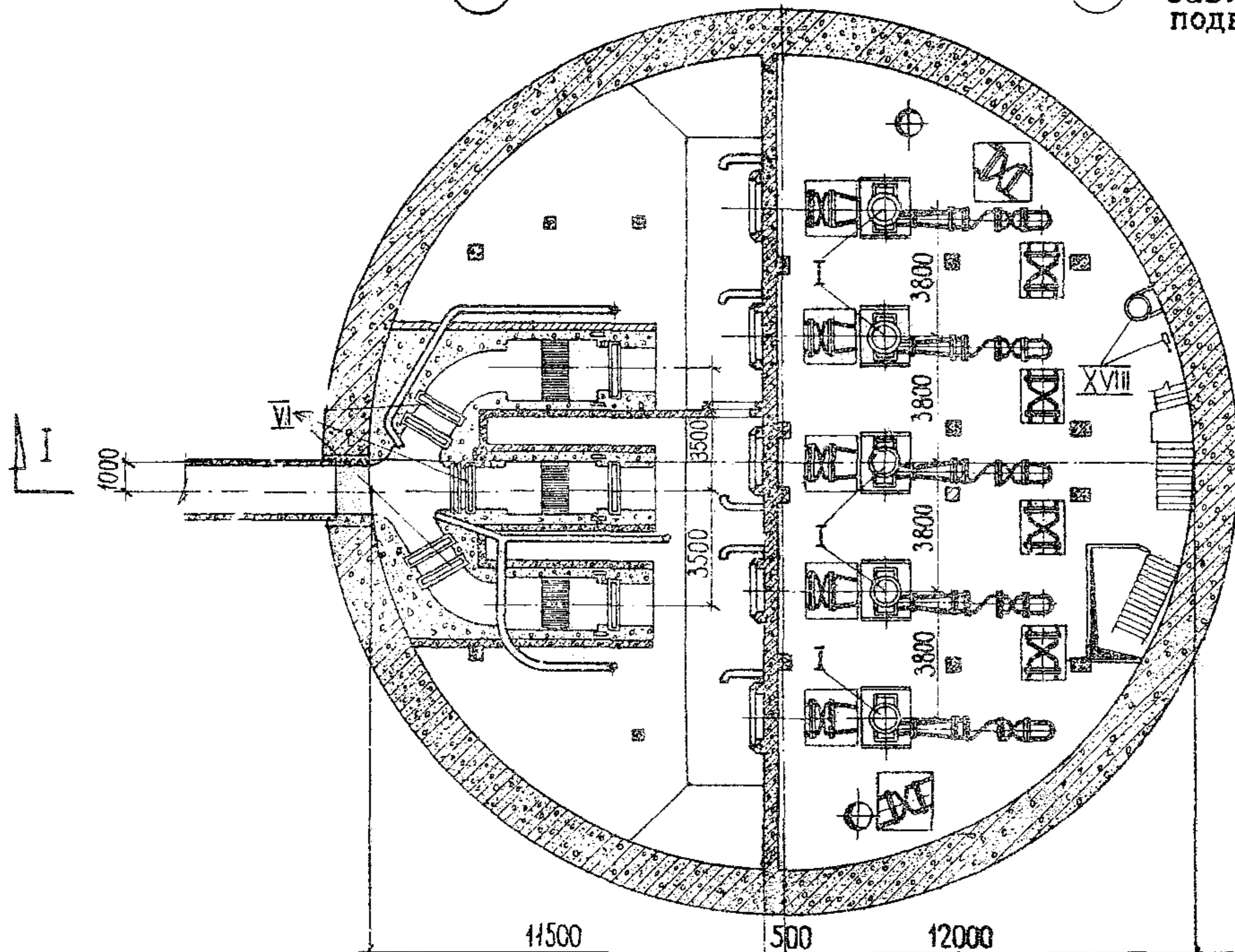
ПЛАН Б-Б
