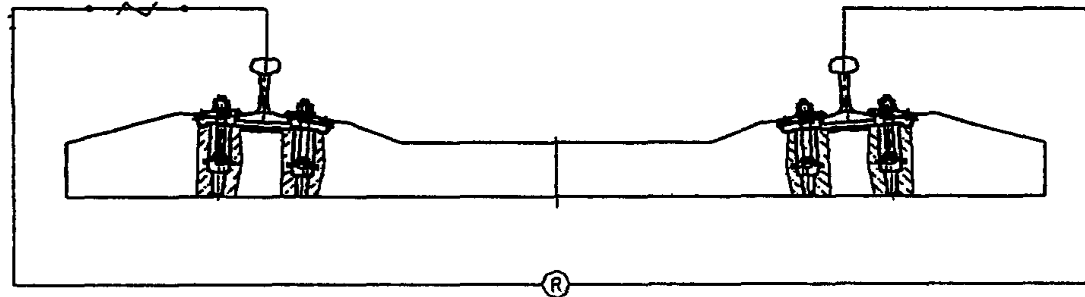
Схема измерения электрического сопротивления
