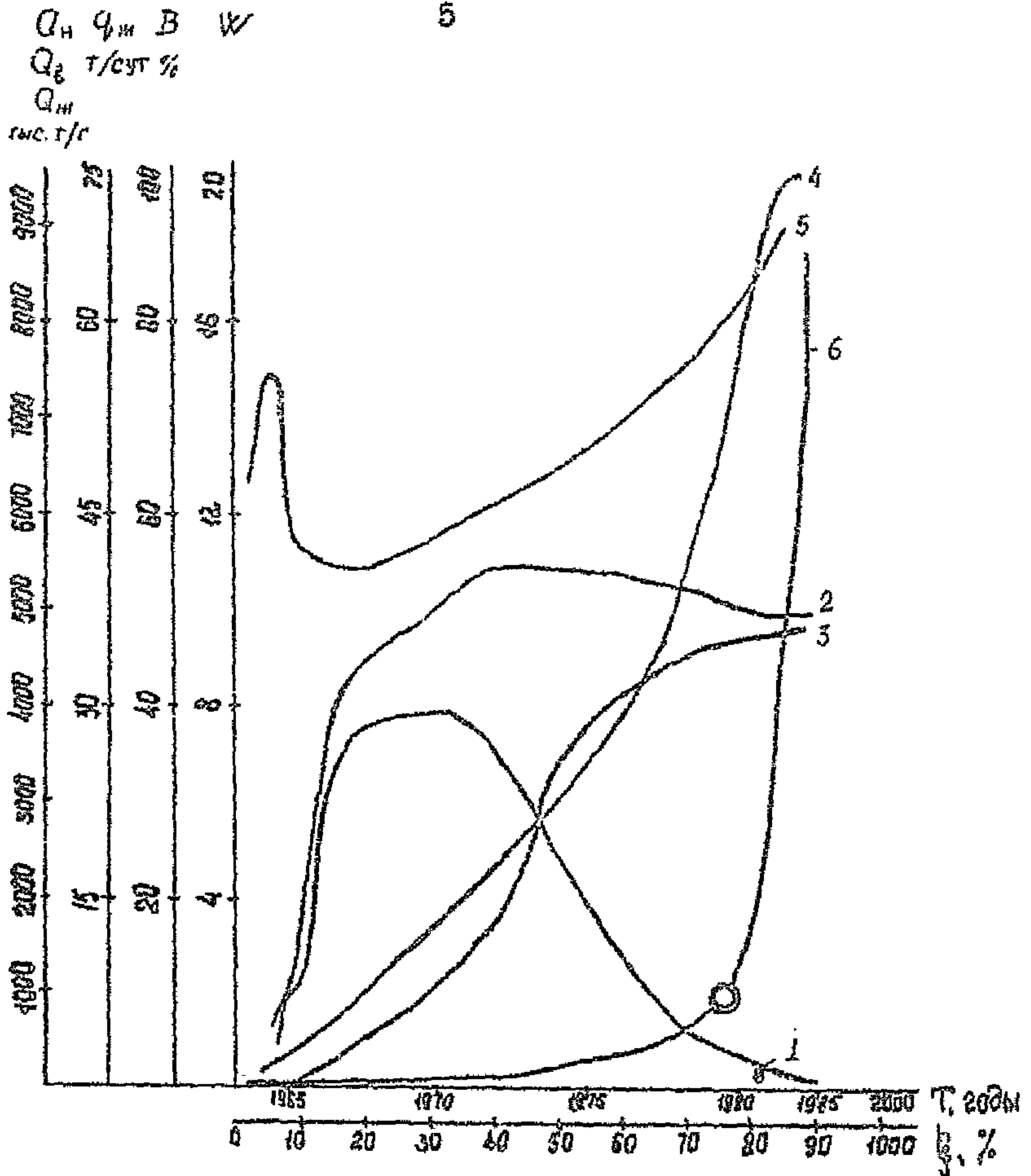
Рис. I. Графики изменения основных показателей Чишминской площади Ромашкинского месторождения:
