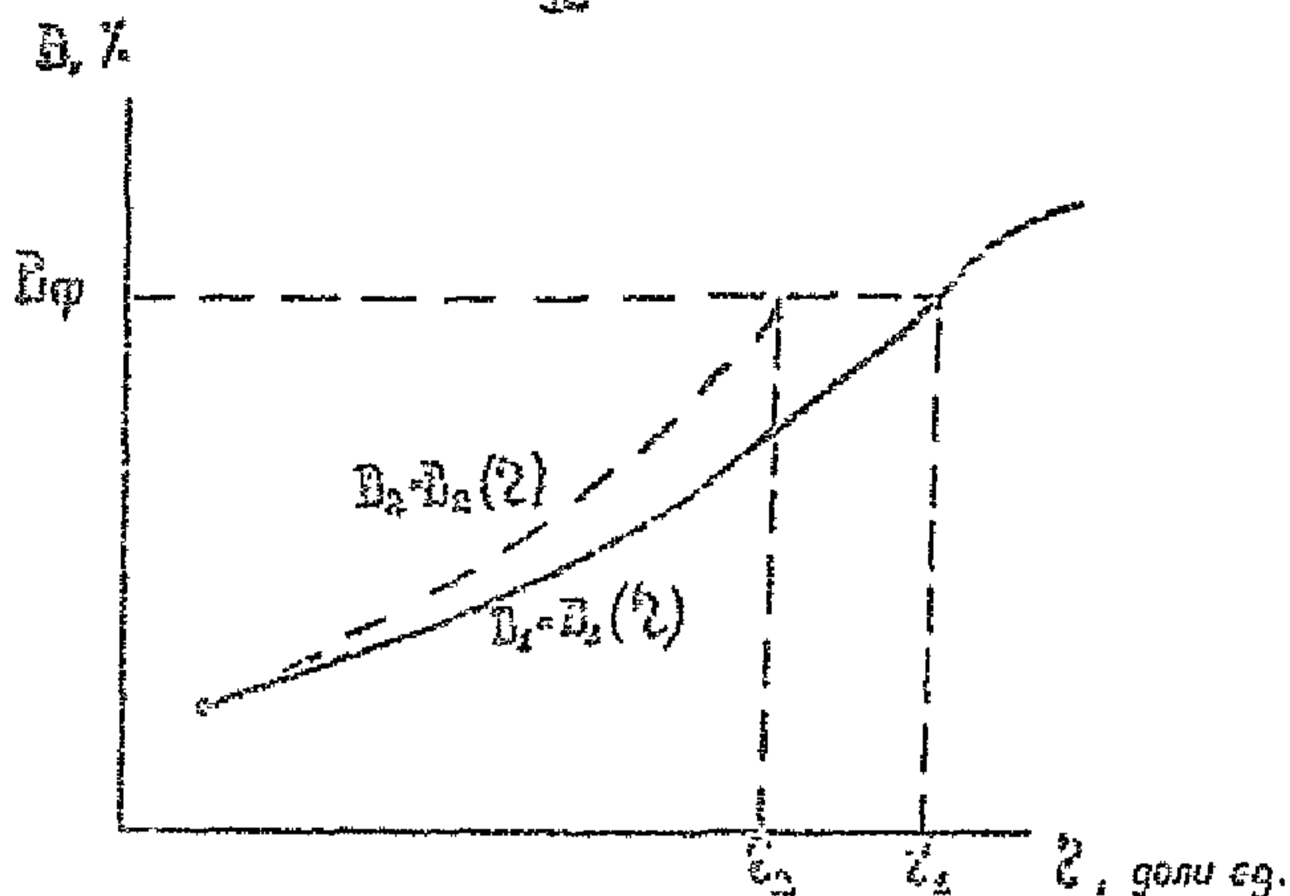
Рис. 2. Графики проектной B_1 = B_1(Z) и фактической B_2 = B_2(Z) зависимостей обводненности продукции от текущей нефтеотдачи.
