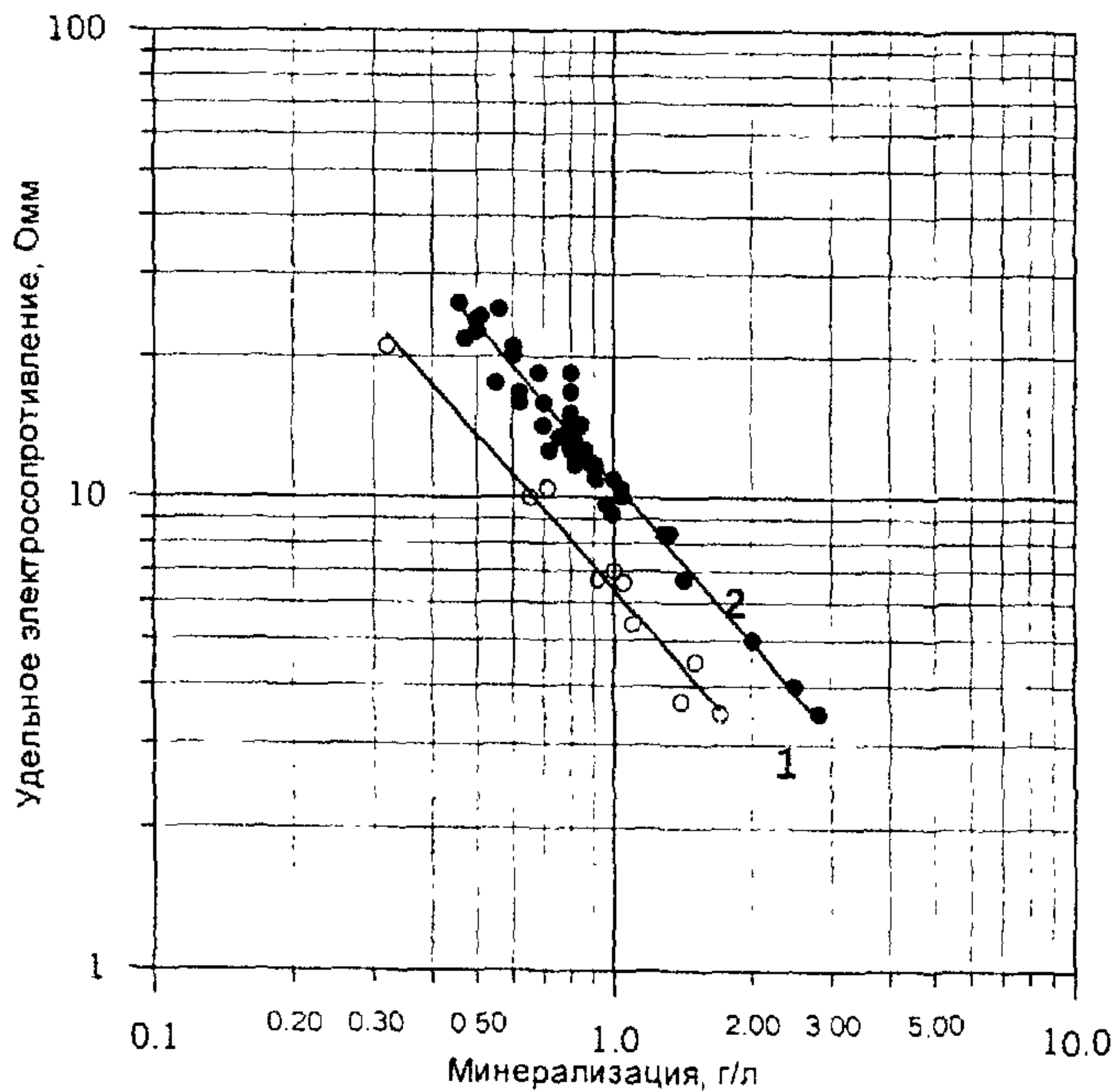
Рис.4.7. Эмпирические зависимости между удельным электросопротивлением и минерализацией воды. (1-Большекизильское МППВ, преимущественно гидрокарбонатные воды, 2- МППВ Татарстана, преимущественно сульфатные воды).
