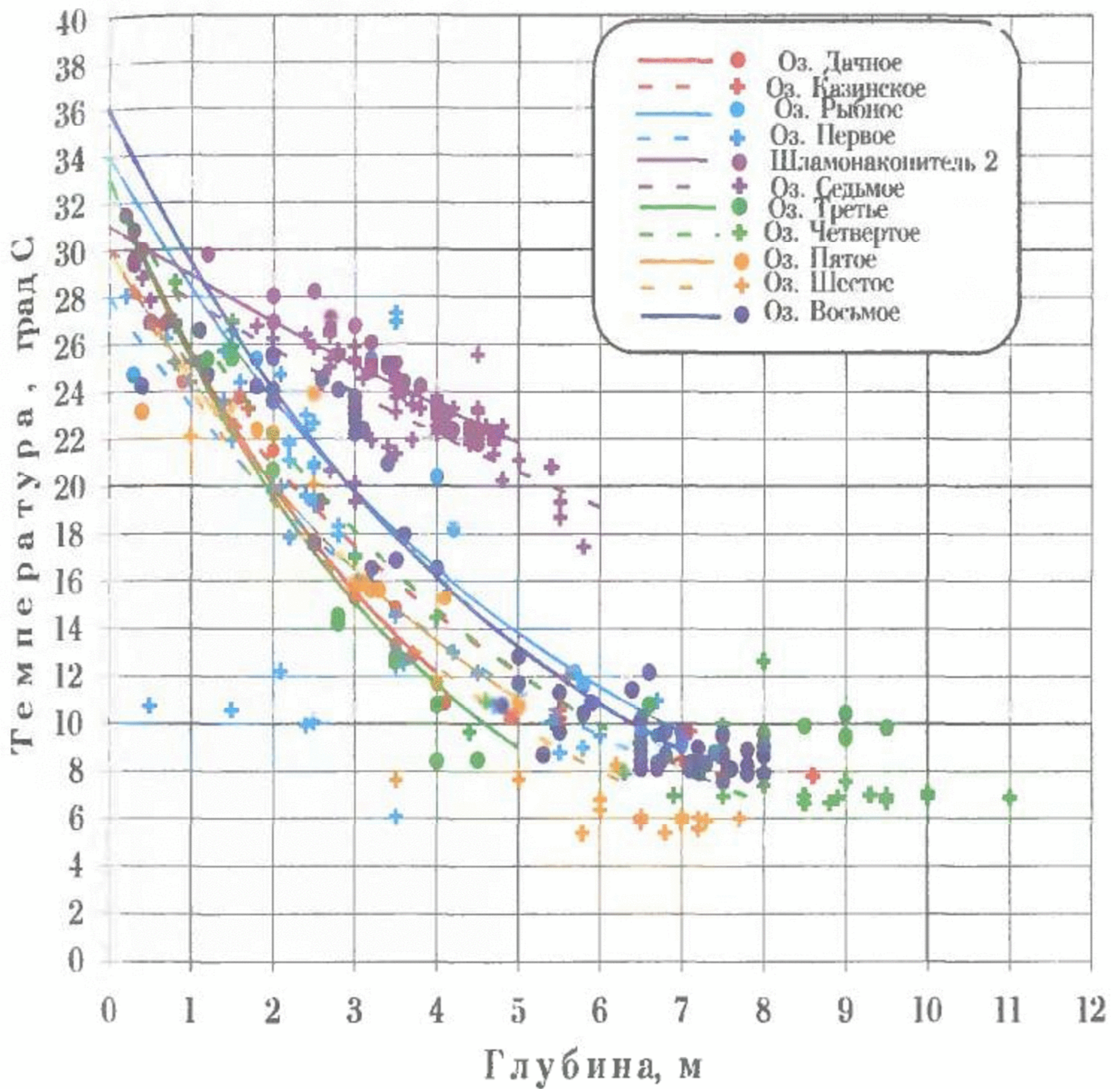
Рис. 4.5. Зависимость температуры придонного слоя воды от глубины по озерам в окрестности г. Тольятти
