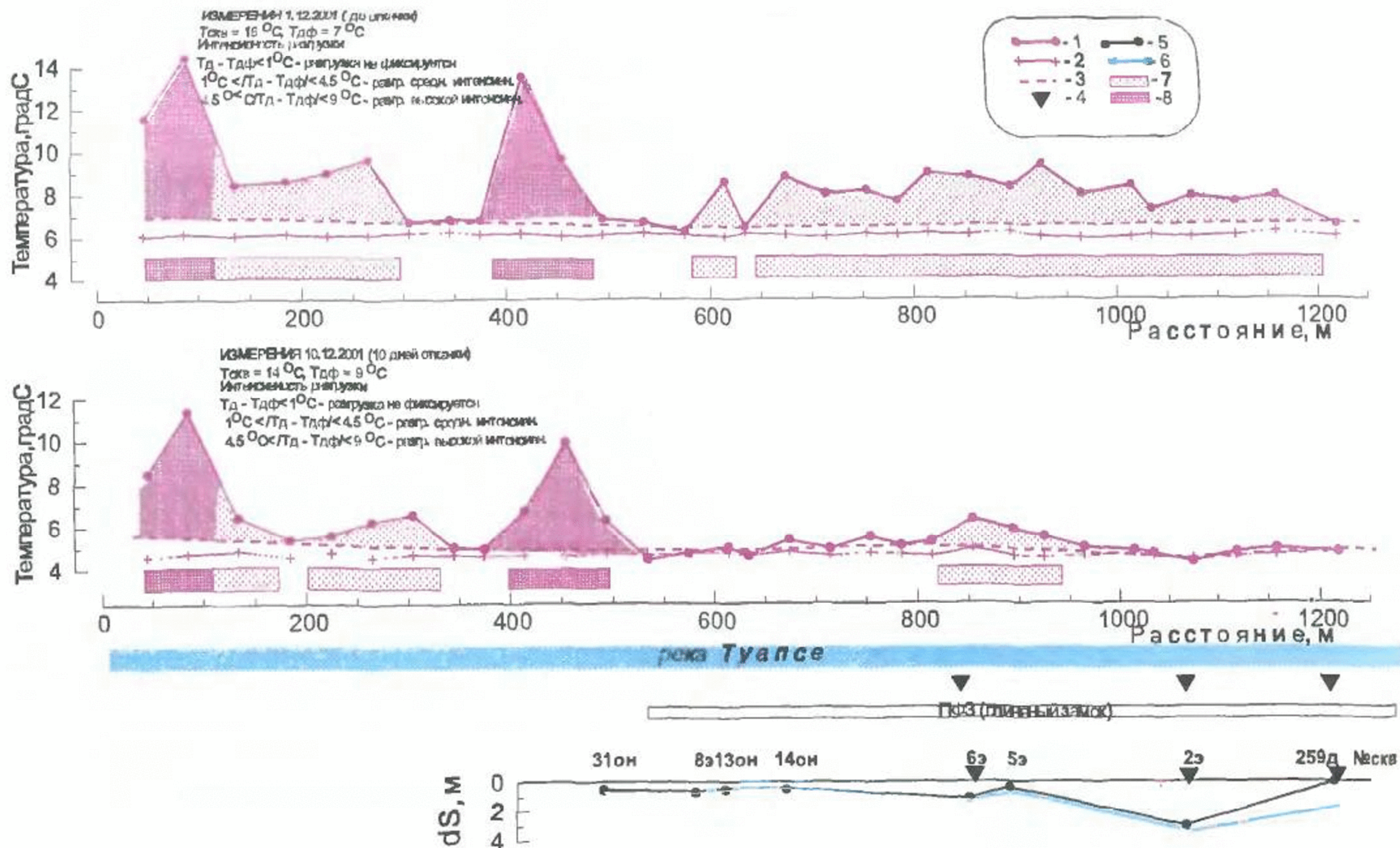
Рис. 4.11. Пример применения термометрии для оценки размеров зон субаквальной разгрузки при откачке из скважин защитной дренажной системы (1-температура донных отложений T_d , 2-температура воды, 3-фоновая температура донных отложений T_{дф} , 4-дренажные скважины, 5-понижение УНП, 6-понижение УПВ или ВНК, температурные аномалии и соответствующие им участки разгрузки: 7-средней интенсивности, 8-высокой интенсивности).
