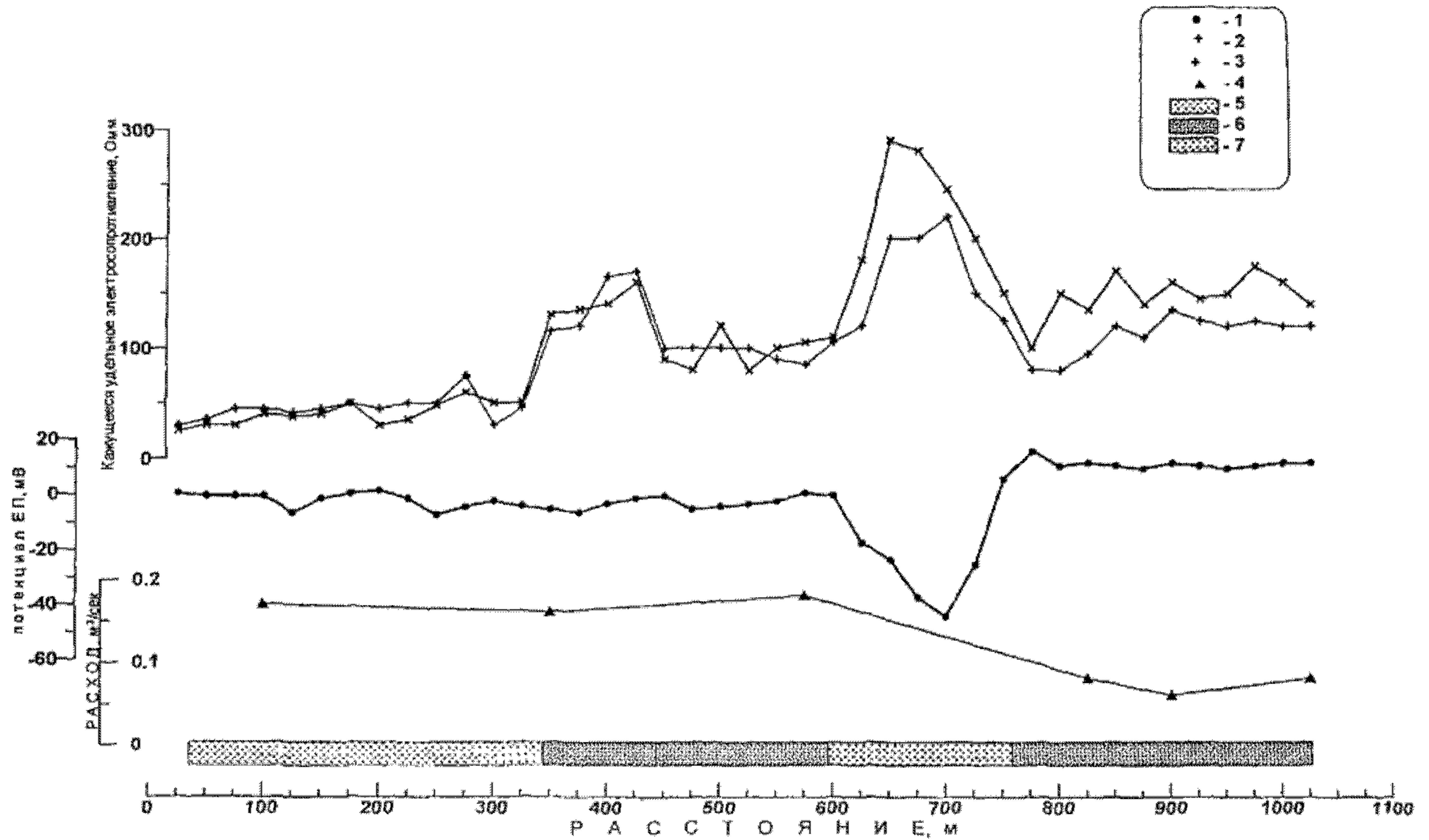
Рис. 4.9. Результаты работ методами ЭП и ЕП по р. Кедровка, Пушкинское МППВ (1 - Уеп, 2, 3 - КС для AD=6\text{м} и 20\text{м} , 4-результаты гидрометрии, 5, 6, 7 - песок глинистый, песок с гравием, песок с радулами и галькой)
