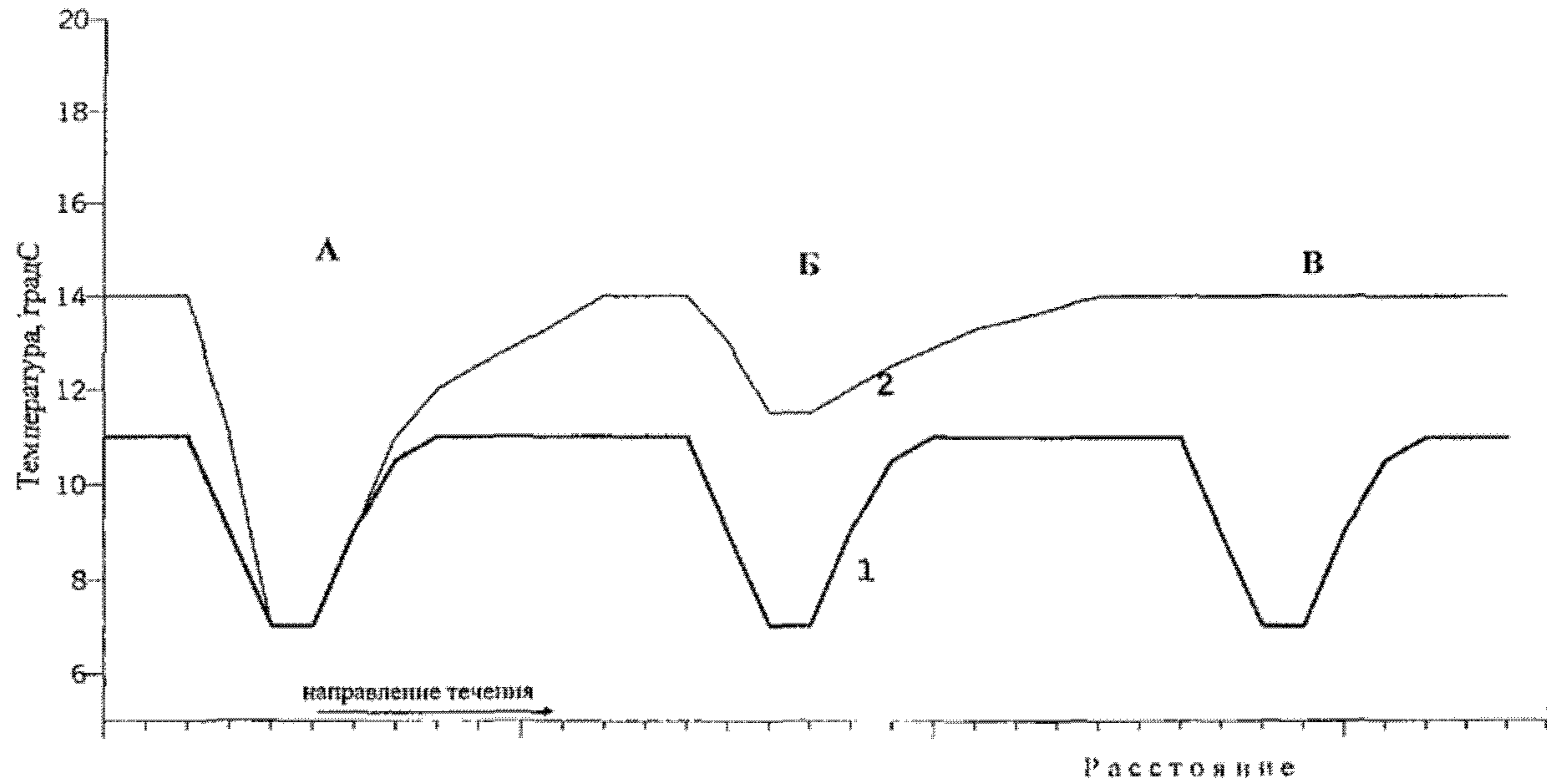
Рис. 4.1. Типовые термограммы на участках субканальной разгрузки по ручьям и рекам в летний период (1-температура придонных отложений, 2-температура воды; относительная интенсивность разгрузки: А-высокая, Б-средняя, В-слабая).
