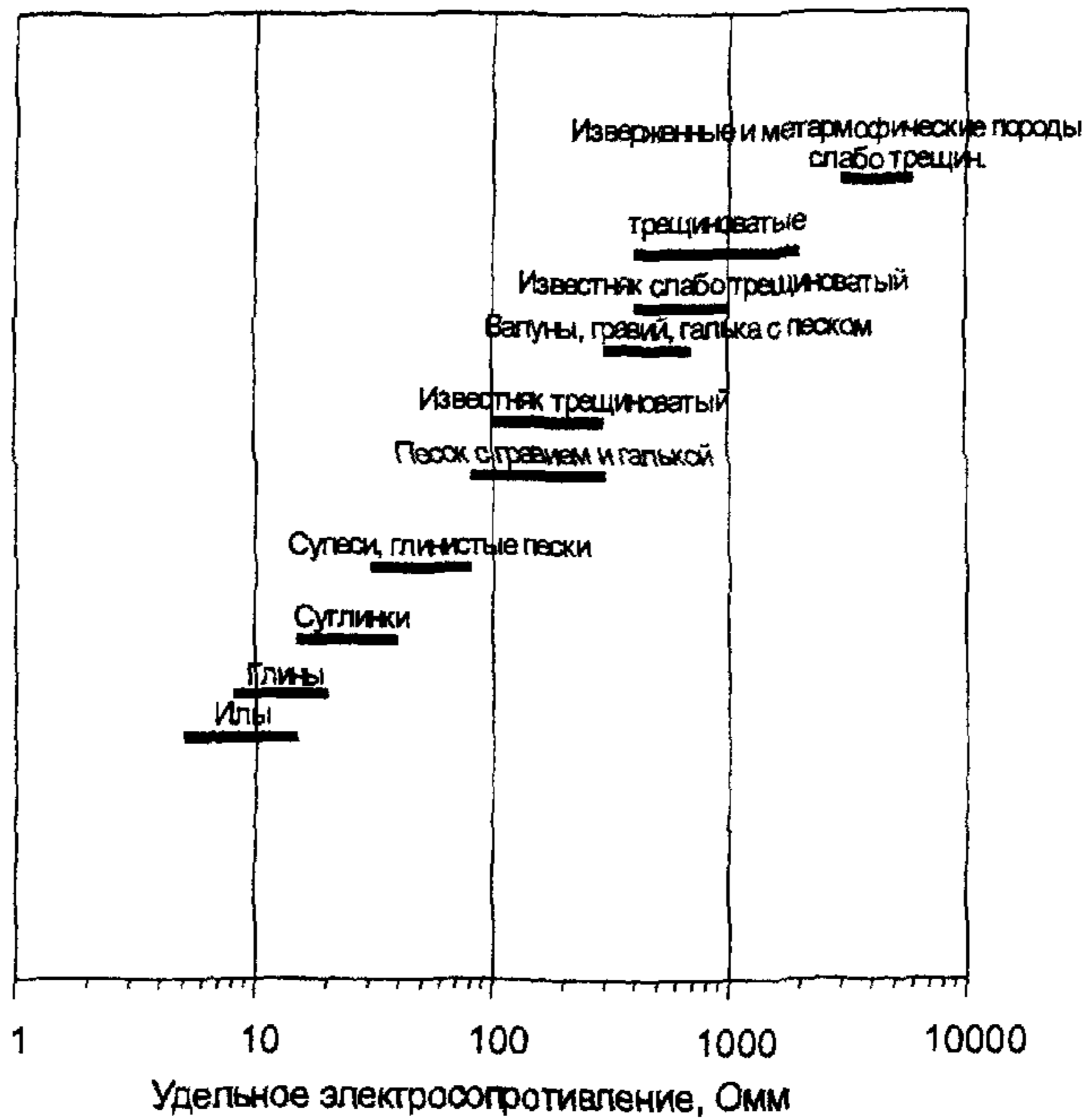
Рис. 4.8. Типовые значения удельного электросопротивления для основных литотипов.
