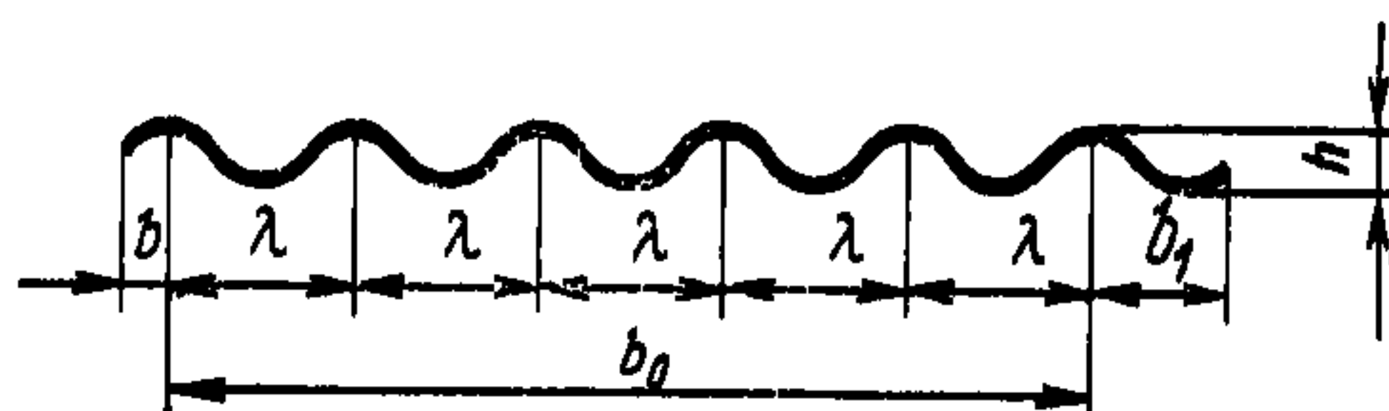
Профиль листа
